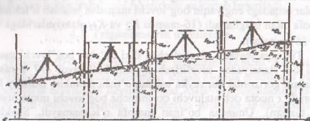
16-rasm. Ketma-ket geometrik nivelirlash.
