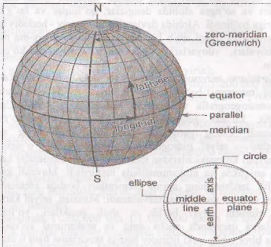
25-rasm. Yer yuzining kenglik va uzoqliklari.
