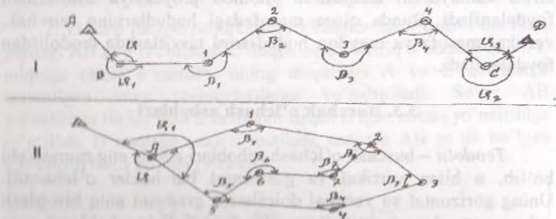
7-rasm. Teodolit yordamida burchaklarni o'lchash sxemasi.
