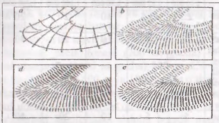
55-rasm. Relyefni shtrixlar bilan tasvirlash sxemasi. a) gorizontallarning ko'rinishi va qiyaliklarni ko'rsatuvchi chiziqlar; b) shtrixlarning joylashtirilishi; d) qiyaliklarning shtrixlar bilan ko'rsatilishi; e) shtrixlarning soyalaridan foydalanish.
