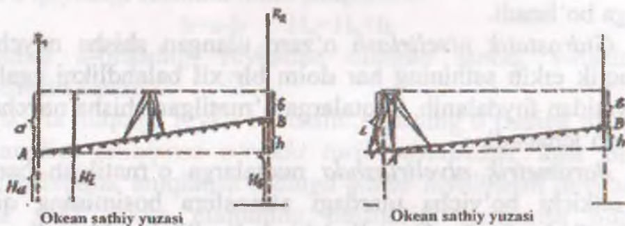
15-rasm. Nivelirlash sxemasi.
