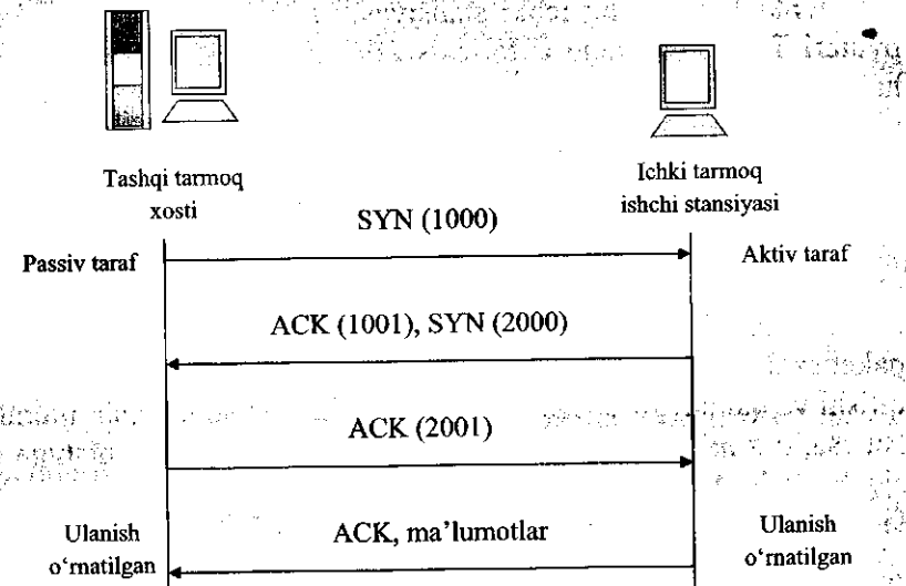
8.7-rasm. TCP protokoli bo'yicha aloqani kvitirlash sxemasi.
