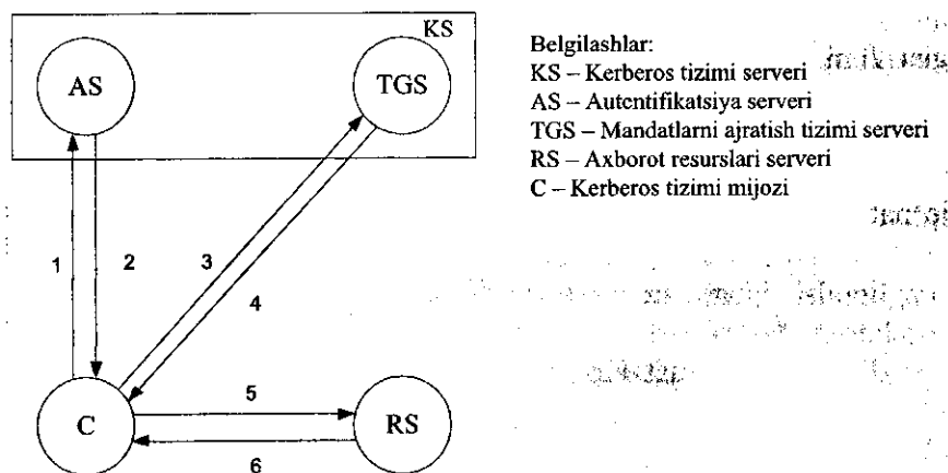
6.2-rasm. Kerberos protokolining ishlash sxemasi.
