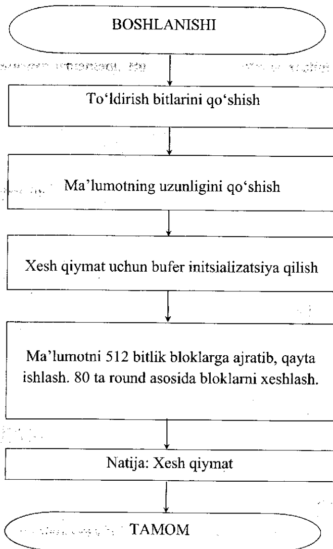
5.18-rasm. SHA1 algoritmi ishlash blok sxemasi.
