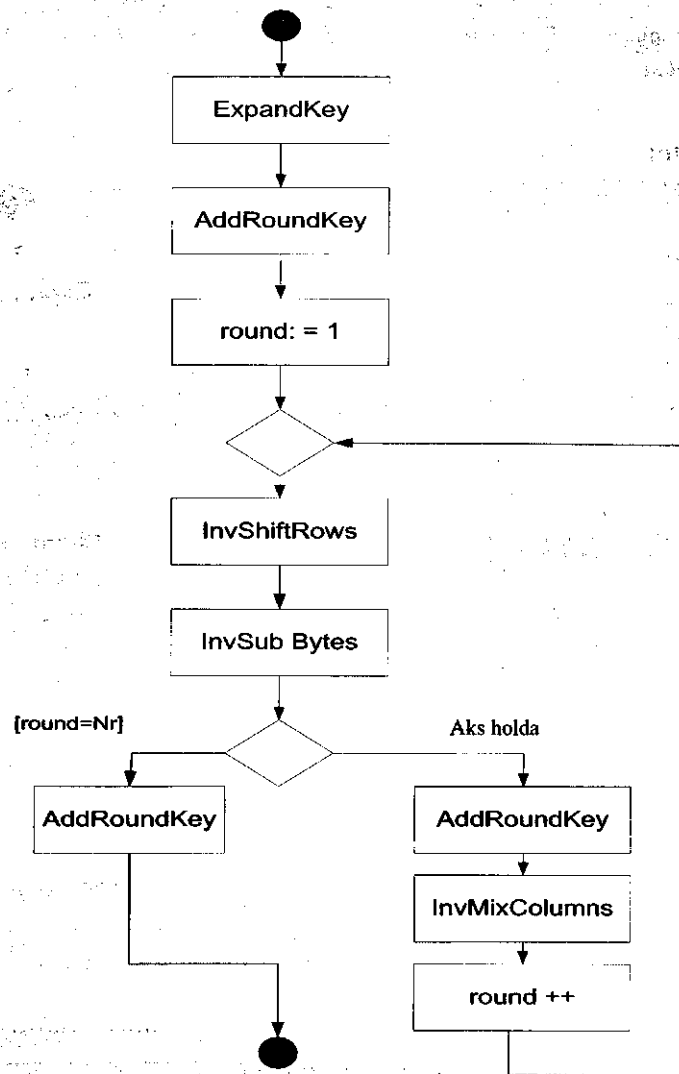
5.13-rasm. Deshifrlash jarayoni.
