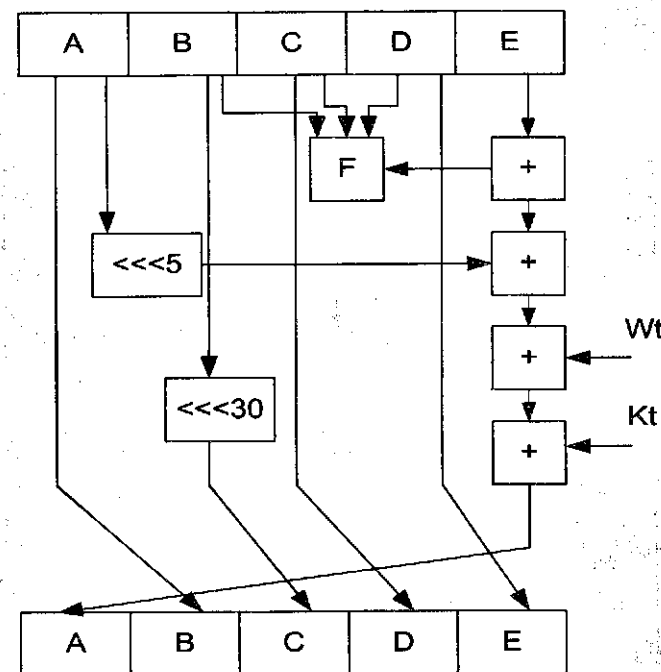
5.17-rasm. SHA-1 algoritmda bir iteratsiyasining sxemasi.
