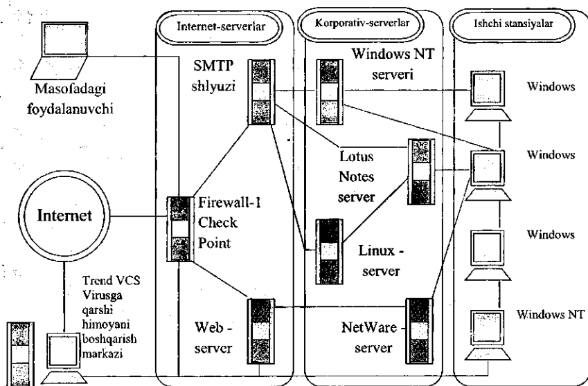
7.2-rasm. Korporativ tarmoqning namunaviy arxitekturası.
