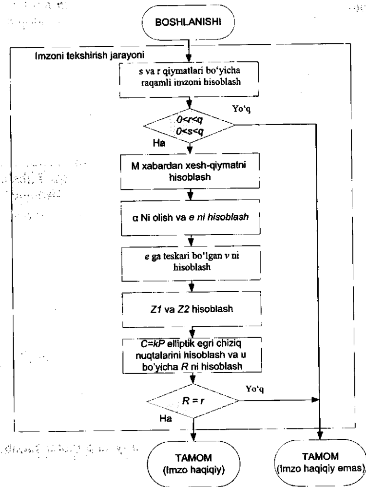
5.24-rasm. Elektron raqamli imzoni tekshirish jarayoni.
