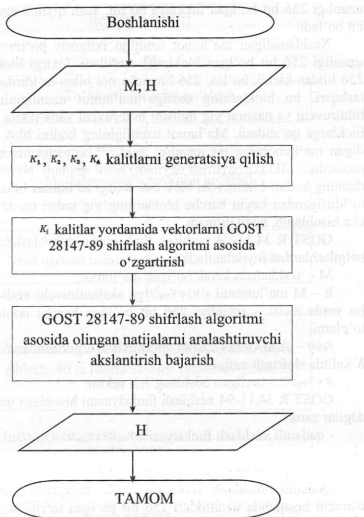
5.19-rasm. Xesh qiymatni hisoblash algoritmining blok-sxemasi.
