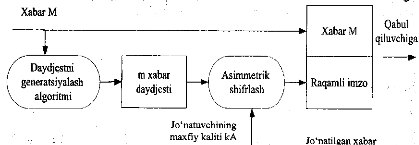
5.20-rasm. Elektron raqamli imzoni shakllantirish sxemasi.
