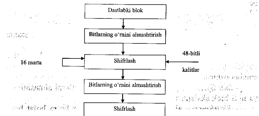
5.11- rasm. DES algoritmda shifrlash jarayonining blok-sxemasi.
