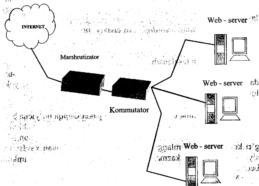
8.16-rasm. Taqsimlangan tarmoqlararo ekranlar yordamida korporativ serverlarni himoyalash.
