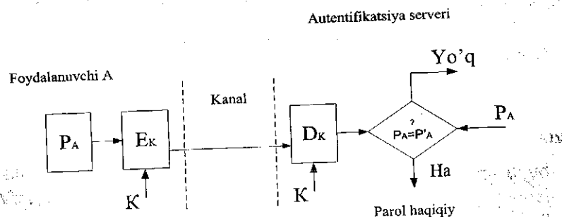
6.1-rasm. Paroldan foydalangan holda oddiy autentifikatsiyalash.
