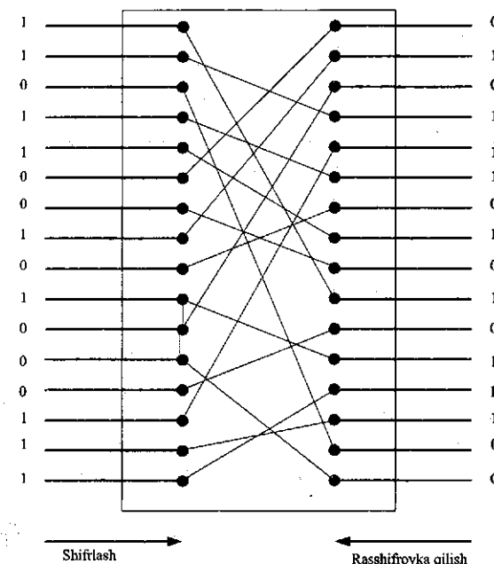
5.7-rasm. O'rin almashtirish sxemasi.
