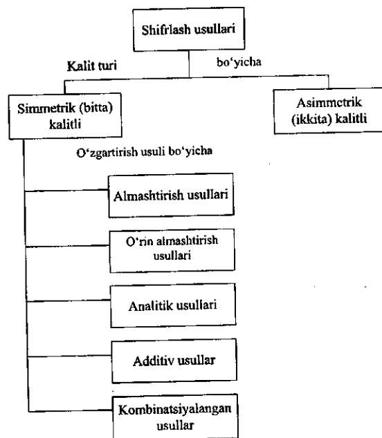
5.1-rasm. Shifrlash usullarining turkumlanishi.
