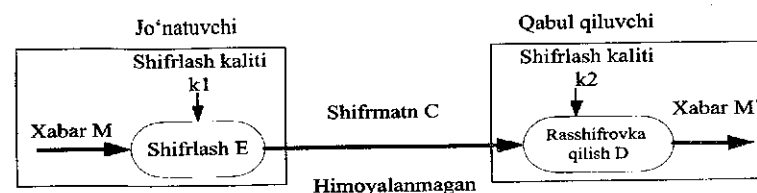
5.8-rasm. Shifrlash kriptotizimining umumlashtirilgan sxemasi.
