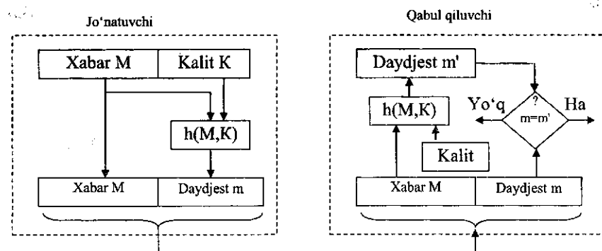
6.5-rasm. Ma'lumotlar yaxlitligini tekshirishda bir tomonlama xesh-funksiyaning ishlatilishi (II-variant).
