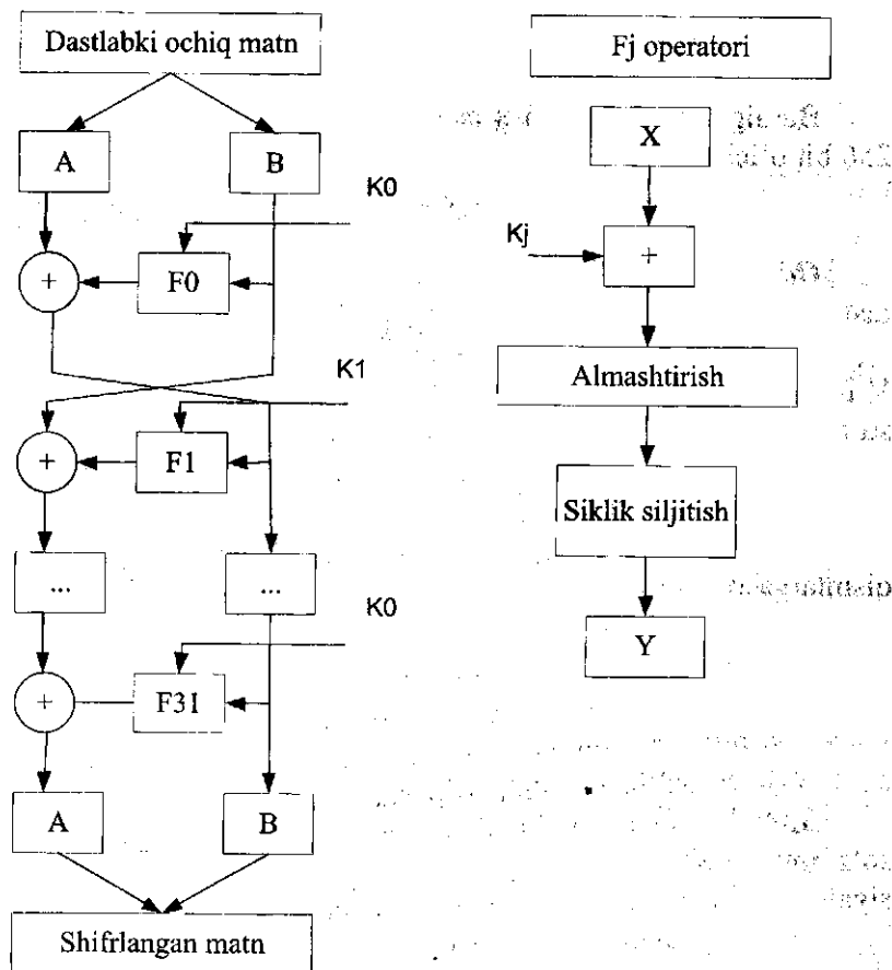
5.14-rasm. Oddiy almashtirish algoritmidagi shifrlash jarayonining blok-sxemasi.
