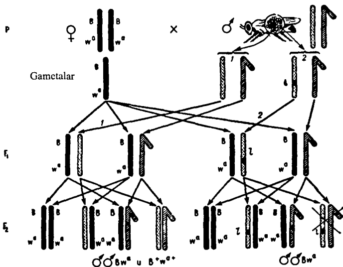
93-rasm. Drozofilada jins bilan birikkan retsessiv letal mutatsiyalarni aniqlashning M-5 metodi (B – qisqirgan ko'z, w^a – o'rik mevasi rangidagi ko'z, l – letal).
