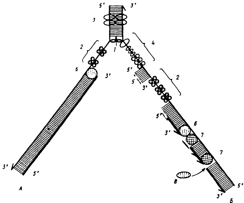
68-rasm. DNK molekulasi replikasiyasining yangi dalillar asosida tuzilgan molekular mexanizmi sxemasi.
