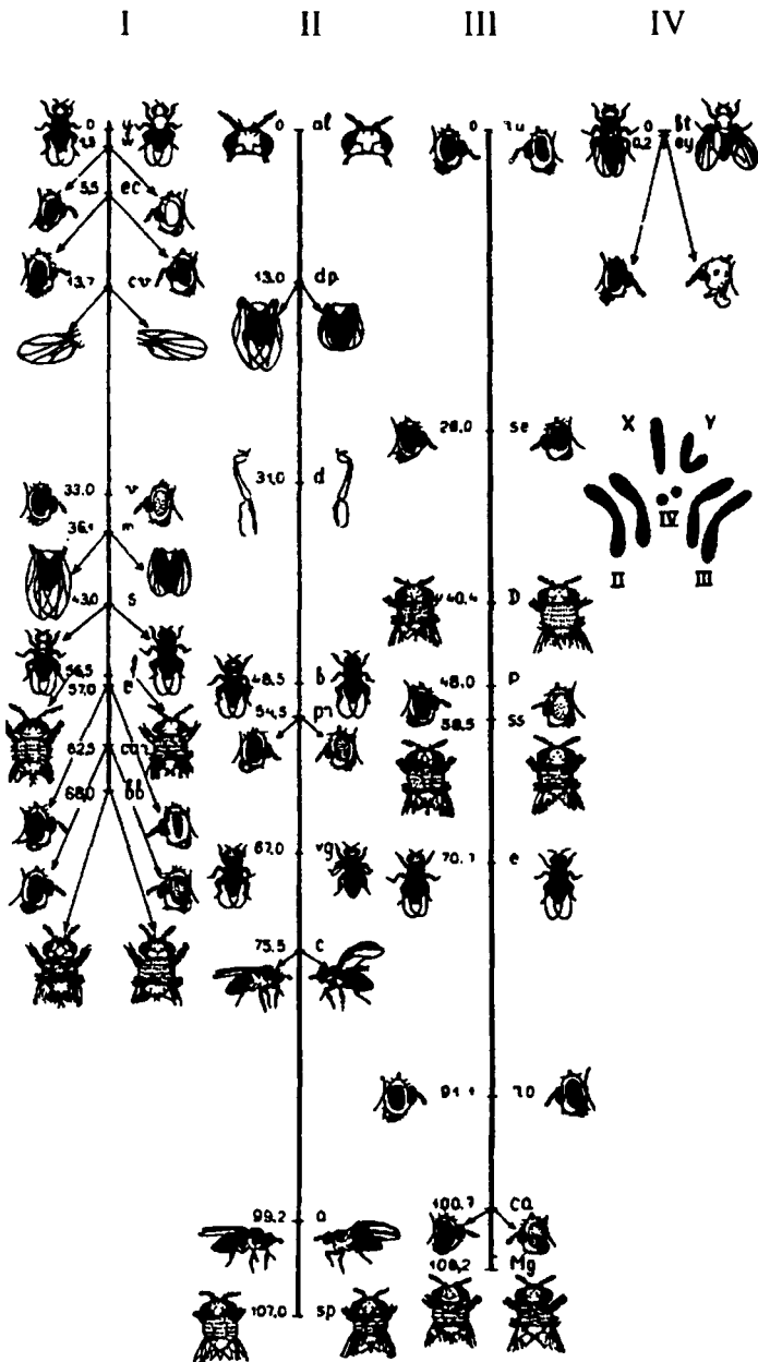
51-rasm. Drozofila xromosomalaringin genetik xaritasi.
