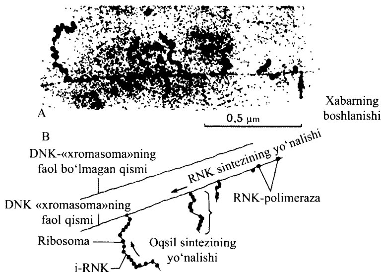
70-rasm. Bakteriyada transkripsiya jarayoni va polisomaning hosil bo'lishi: A. i-RNK ning ketma-ket hosil bo'lish bosqichlarini ko'rish mumkin bo'lgan xromosomaning elektron mikrografiyasi va ribosomaning birikishi. B. Mikrografiyada aks etgan jarayon strukturasi sxematik tasviri.
