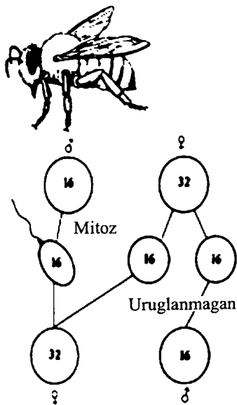
41-rasm. Jinsni belgilashning to'rtta tipi.
