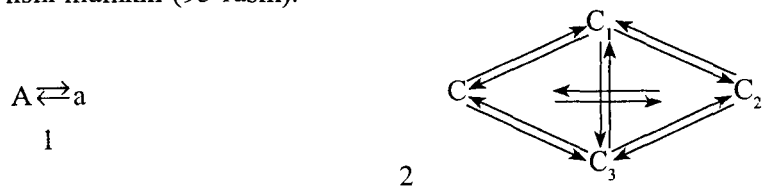
95-rasm. Ko'p allellilik tizimining vujudga kelish sxemasi: 1 – bir genning ikki alleli; 2 – to'rtta alleldan iborat tizim; strelkalar mutatsiyalarning yo'nalishini ko'rsatadi.
