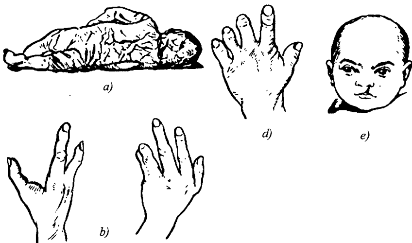
119-rasm. Odamda dominant mutatsiyalar: a – ixtiozis, b – sindaktiliya, d – braxidaktiliya, e – quyvon lab. (Uolles va Dobjansiy bo'yicha.)
