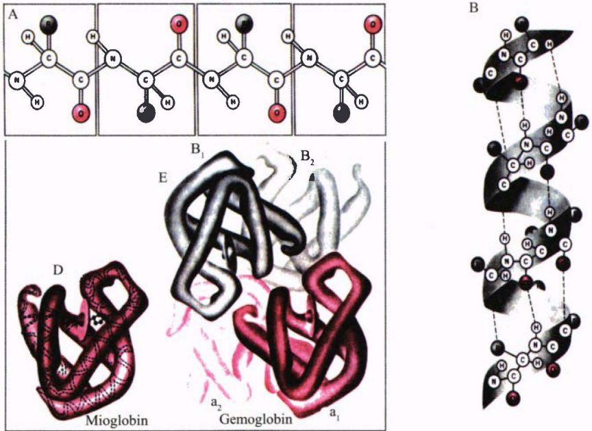
78-rasm. Oqsilning ikkilamchi, uchlamchi va to'rtlamchi strukturasi.
