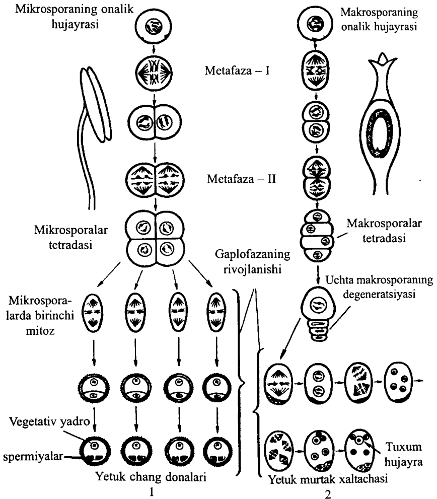
38-rasm. Rivojlanishning qiyosiy sxemasi. Gulli o'simliklarda erkaklik mikrosporangenez va mikrogametogenezi (1), urg'ochilik makrosporangenez va makrogametogenezi (2) hamda jinsiy hujayralarning yetilishi.
