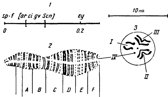
55-rasm. Drosophila IV xromomasining sitologik va genetik xaritalarini o'zaro taqqoslash. 1 – genlari ko'rsatilgan genetik xarita (genlarning belgilanishini 51-rasmdan qarang); 2 – so'lak bezidan olingan gigant xromosomaning sitologik xaritasi. (A – F – ketma-ket joylashgan qismlari); 3 – gangliya hujayrasidan olingan metafaza plastinkasi (so'lak bezining IV xromosomasi bilan metafaza plastinkasi kattaligi taqqoslangan, mashtablari bir xil).
