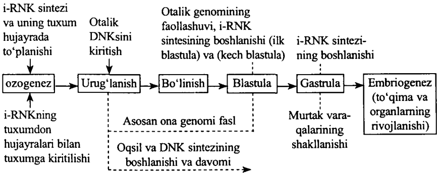
106-rasm. Baqaning ilk embriogenezida genlar faolligining o'zgarishi (Gerdon bo'yicha).
