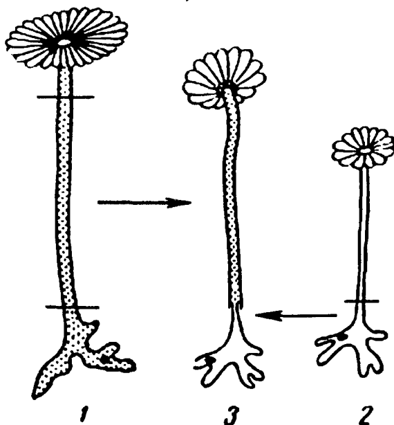
57-rasm. Bir hujayrali Acetabularia suv o'tlari sallasini shakllanishiga yadroning ta'siri.
