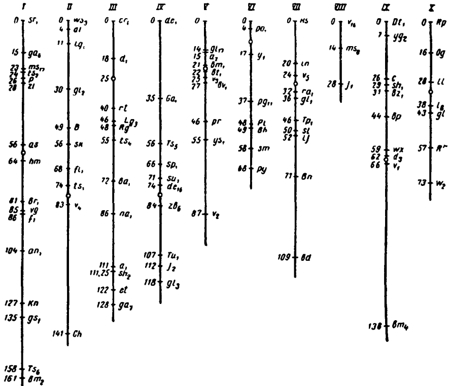
52-rasm. Makkajo'xori xromosomalarning genetik xaritasi.
