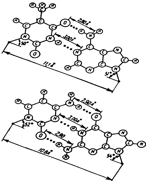
65-rasm. DNK molekulasida nukleotidlarning komplementar bog'lanish tartibi.
