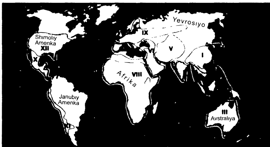
121-rasm. Madaniy o'simlik turlari kelib chiqishining birlamchi markazlari: I – Xitoy – Yaponiya; II – Indoneziya – Hindixitoy; III – Avstraliya; IV– Hindiston; V – O'rta Osiyo; VI – Old Osiyo; VII –O'rta dengiz; VIII – Afrika; IX – Yevropa – Sibir; X – Markaziy Amerika; XI – Janubiy Amerika; XII – Shimoliy Amerika.
