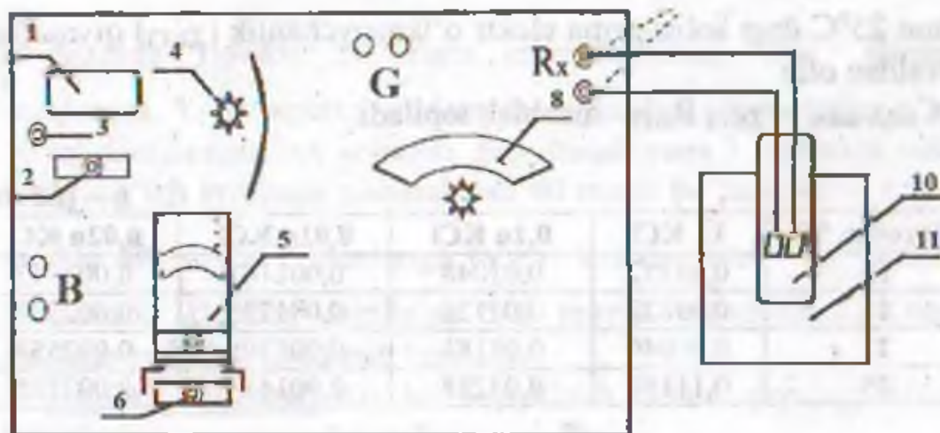
VII.11-rasm. Renxord ko'prigi R-38 qurilmasining tuzilish sxemasi
