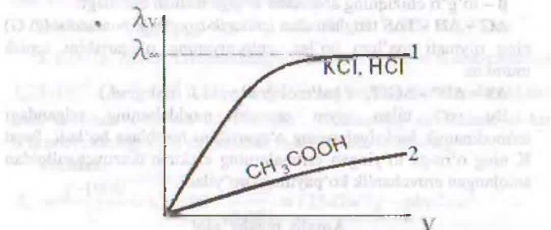
II.12 – rasm. Ekvivalent elektr o'tkazuvchanlikni suyultirish soniga bog'liqlik grafigi:
