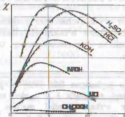
VII.1 - rasm. Solishtirma elektr o'tkazuvchanlikning eritma konsentratsiyasiga bog'liqligi
