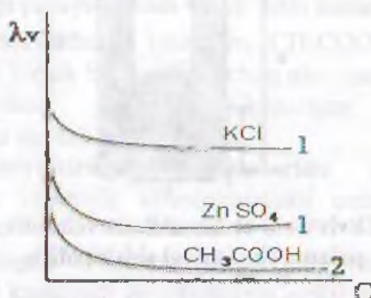
VII.3-rasm. Ekvivalent elektr o'tkazuvchanlikning konsentratsiyaga bog'liqlik grafigi.
