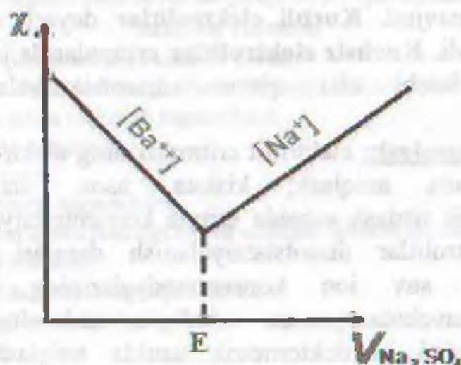
VII.10-rasm. \text{BaCl}_2 ni \text{Na}_2\text{SO}_4 bilan titrlash grafigi
