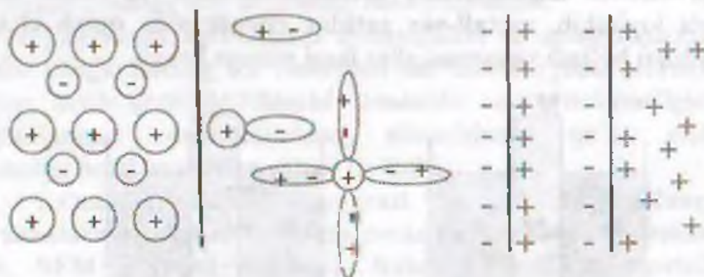
VIII.2-rasm. Qo'sh elektr qavat tuzilishi
