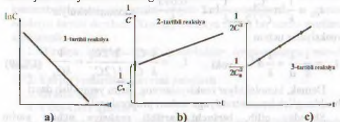
IX.2-rasm. Reaksiya tartibini ifodalovchi grafiklar:
