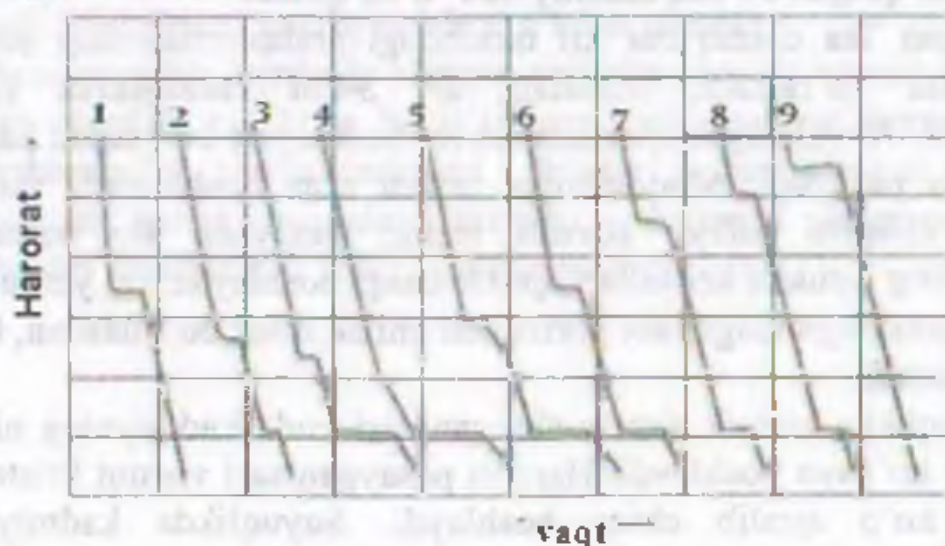
V.1 – rasm. Sovush egri chiziqlari
