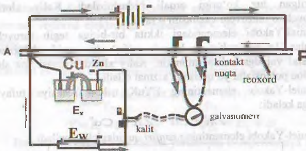
VIII.10 – rasm. EYuK o'lchashni kompensatsion sxemasi
