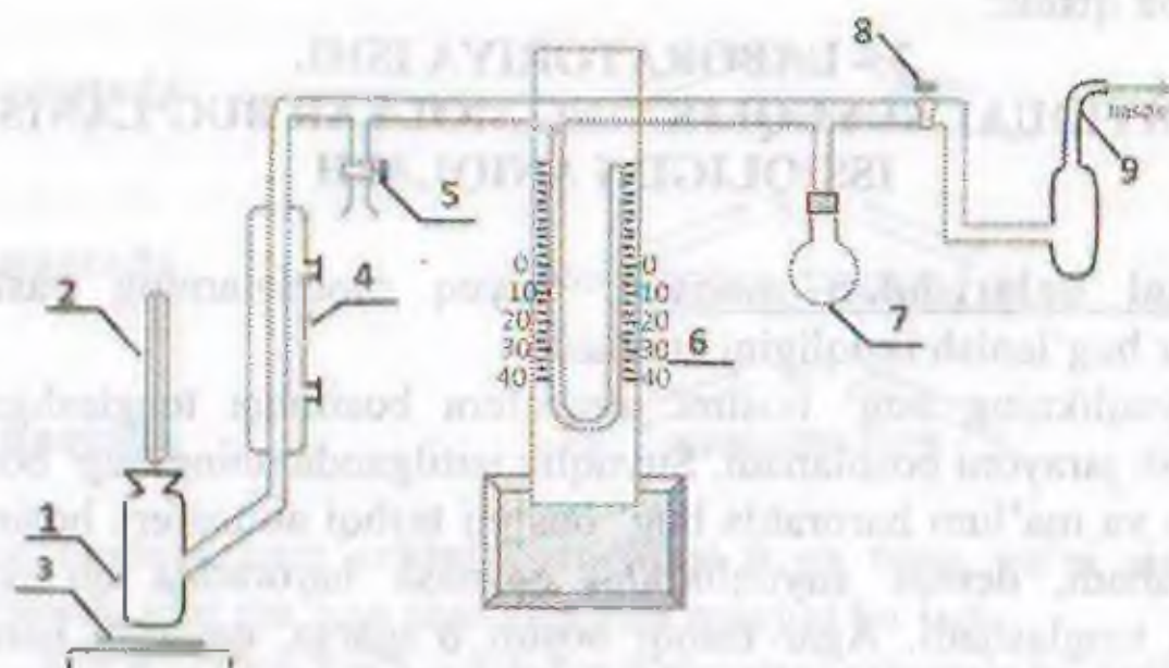
IV.3 – rasm. Tajriba uchun ishlatiladigan qurilma sxemasi
