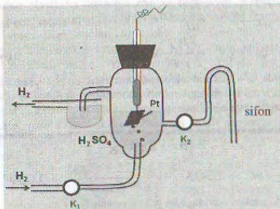
VIII.4 – rasm. Vodorod elektrodi
