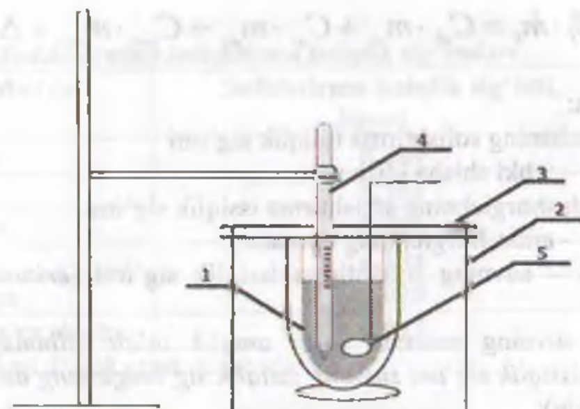
1.1-rasm. Laboratoriyada qo'llaniladigan oddiy kalorimetr qurilmasi
