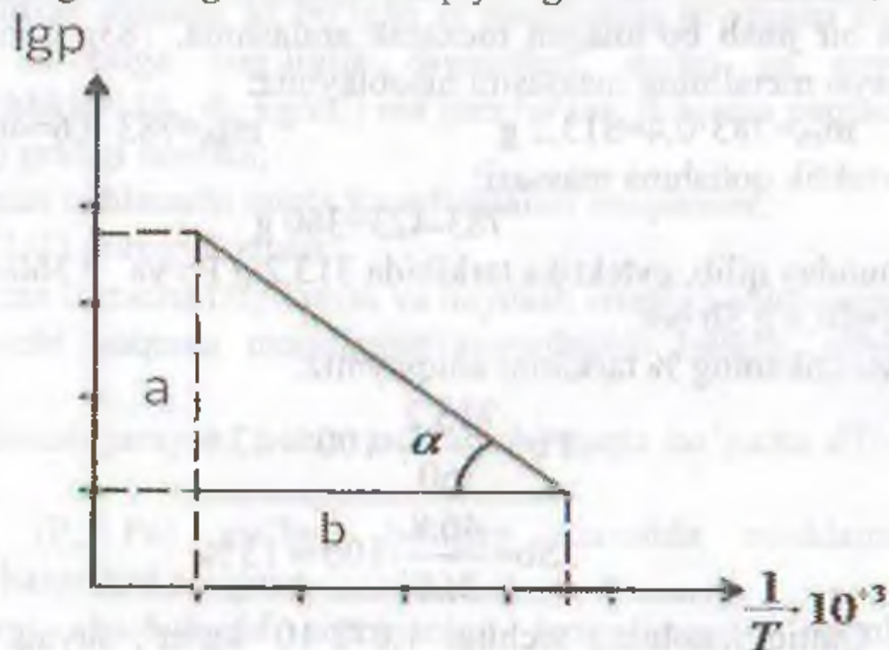
IV.4 – rasm. Haroratni bosim bilan bog'liqlik grafigi
