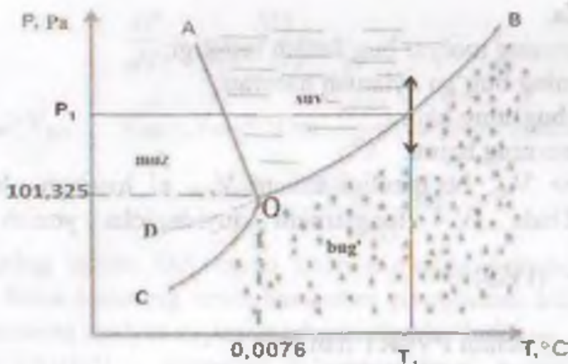
IV.1– rasm. Suvning holat diagrammasi
