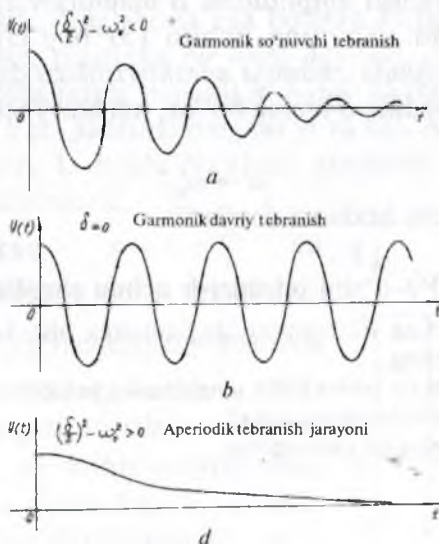
152-chizma.
