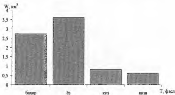
3.7.3-rasm. Oqim hajmlarining mavsumlar bo'yich taqsimlanishi
