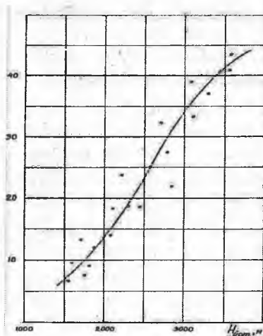
1.10.1-rasm. Oqim moduli ( M )ning havzaning o'rtacha balandligi ( H_{0,rt} ) ga bog'liqligini ifodalovchi chizma
