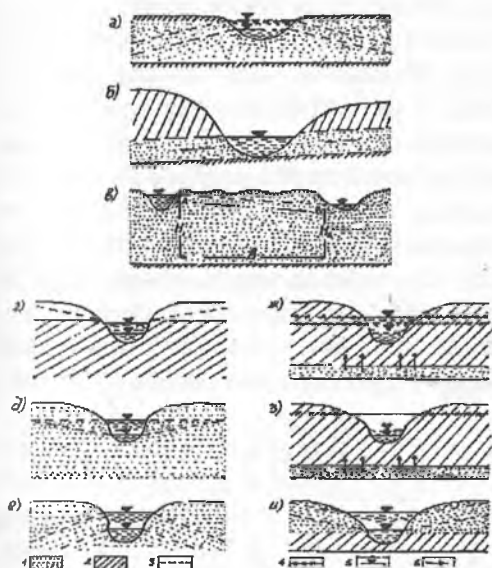
6.3-rasm. Grunt suvlarining daryo oqimi hisobiga to'yinishi (a, b, v), grunt hamda daryo suvlarining gidravlik bog'liqligi (d,e,j,z,i).
