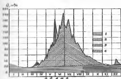
2.2-rasm. Daryo oqimi gidrografini vertikal bo'laklarga ajratish
