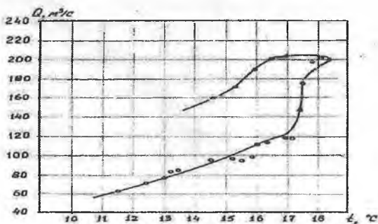
1.13.3-rasm. Seldara daryosi (mug'suv daryosi irmog'i) o'rtacha dekadali suv sarflarining Oltinmazor mete- orologik stansti- yasida kuzatilgan havo harorati bilan bog'liqligi.
