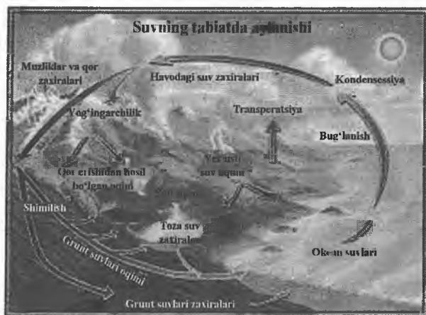
1-rasm. Tabiatda suvning aylanishi.
