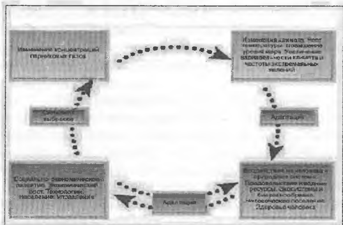
2.5.2 – rasm. Iqlim o‘zgarishi va majmuali yondoshuv Manba: birinchi o‘n yillik, RKIK OON, 2004
