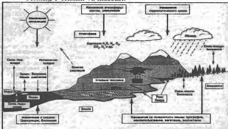
1.1-рasm. Iqlimiy sestimaning sxematik tasviri (Manba: IPCC 1995)
