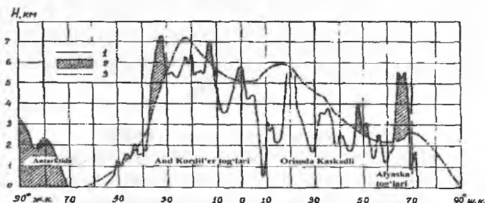
1.13.1-rasm. Qor chizig'i balandligining And va Kordiller tog'lari orqali o'tkazilgan kengliklar bo'yicha o'zgarishi (V.M.Kotlyakov ma'lumoti).
