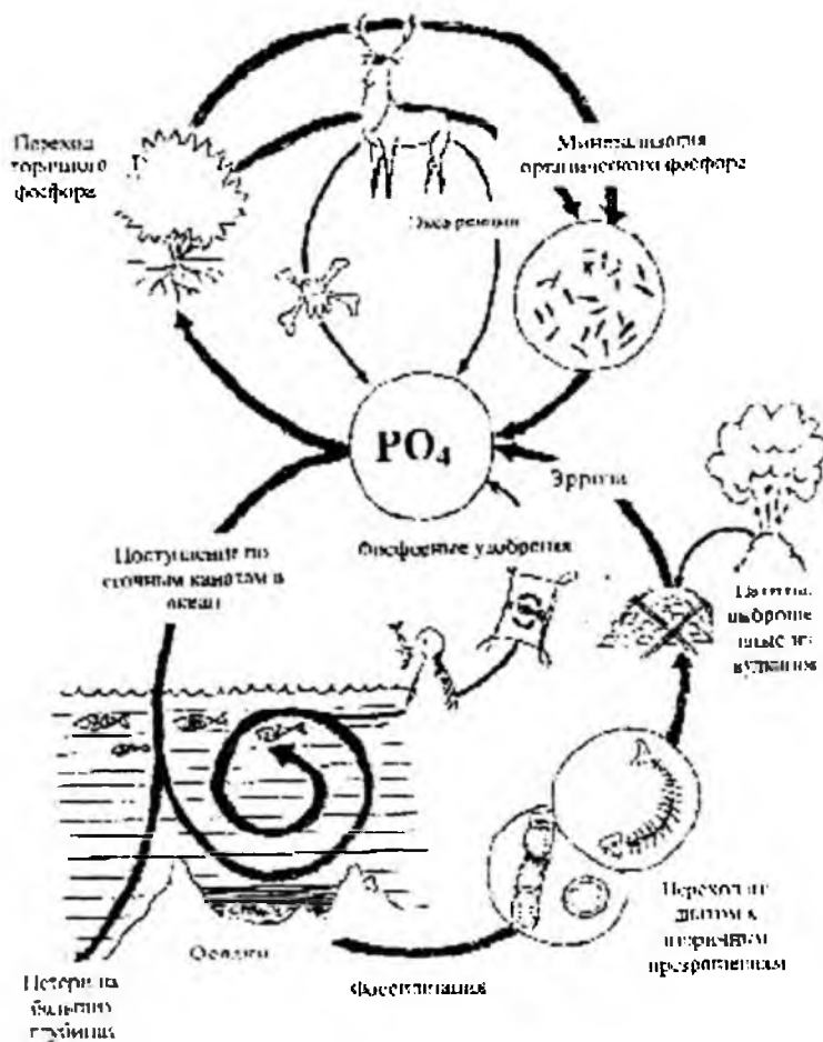
Рис. 13. Круговорот фосфора (по Риклефсу)
