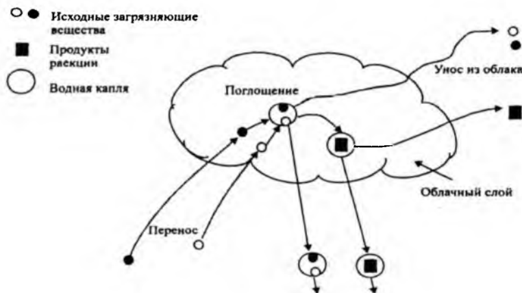
Рис. 22. Схема процессов с участием облачного слоя
