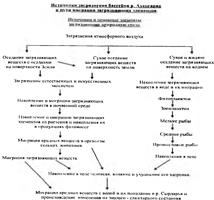
Рис.18, Источники загрязнения бассейна р. Ахангаран и пути миграции загрязняющих элементов
