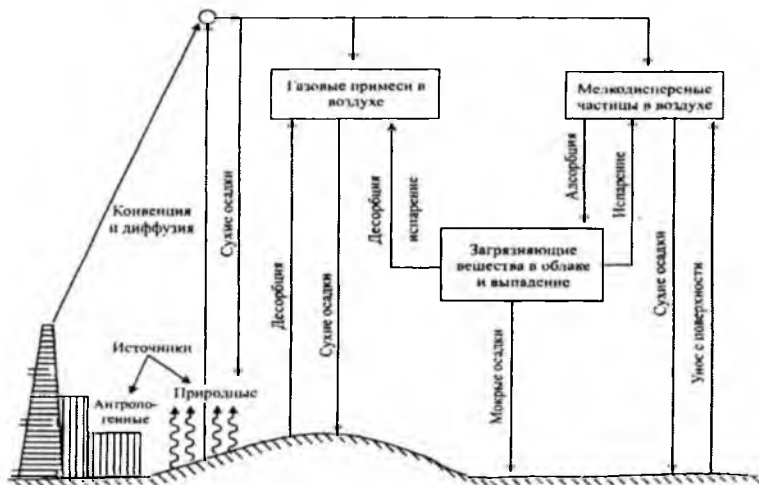
Рис. 21. Схема процессов выбросов веществ в атмосферу и трансформация исходных веществ в продукт с последующим выпадением в виде осадков
