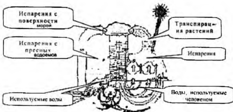
Рис. 11. Круговорот воды в природе.
