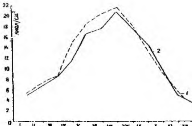
Рис.16. Месячные суммы суммарной солнечной радиации ккал/см 2 (1 - 1976 г.; 2 - 1988 г.) на территории Узбекистана.
