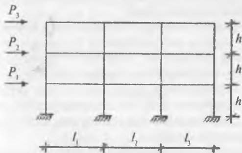
13.9- rasm. Temir-beton rama.
