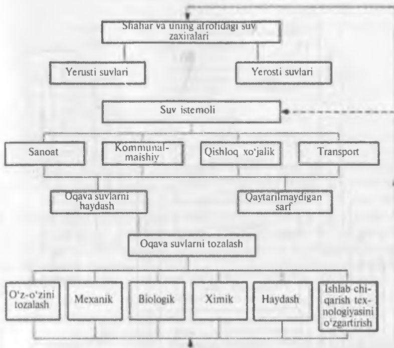
2.2- rasm. Suv zaxiralardan foydalanish va ularni qayta ishlash.
