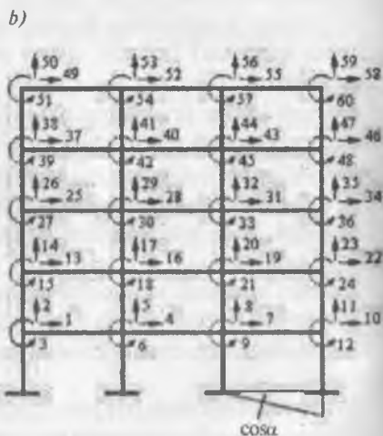
12.4- rasm. 5 qavatli rama: a) berilgan sxema; b) hisobiy sxema.
