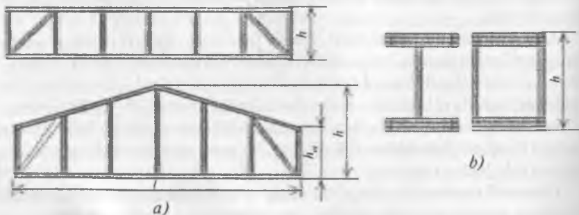
10.1- rasm. Yogʻoch konstruksiyali fermalar.
