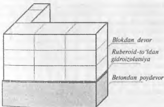
7.2- rasm. Blokli devor konstruksiyasi.
