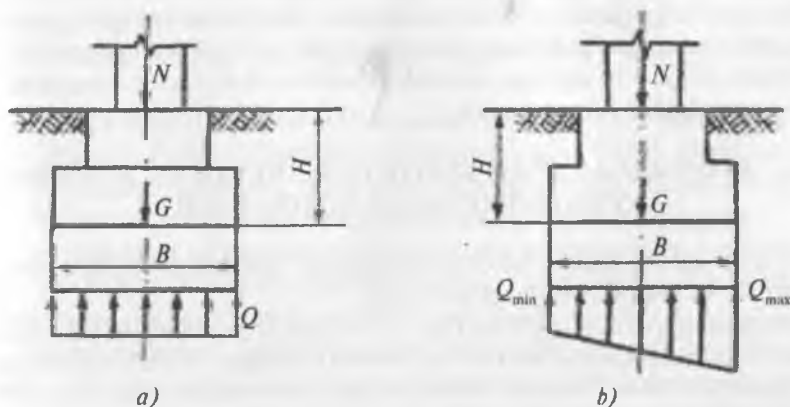
4.13- rasm. Markaziy (a) va markazdan tashqari (b) yuk ta'siridagi poydevorni hisoblash chizmasi.
