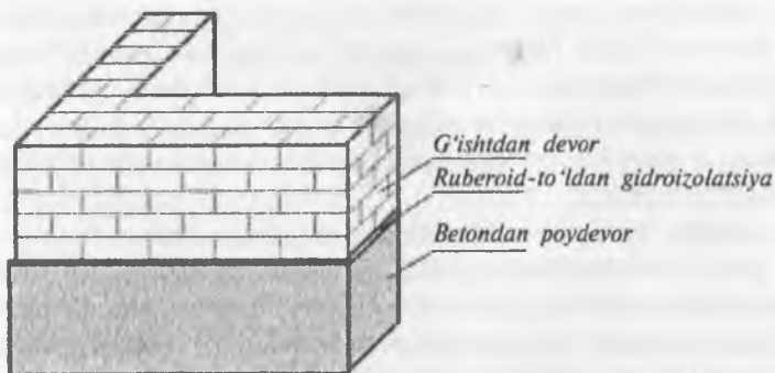
7.1- rasm. G'isht devor konstruksiyasi.
