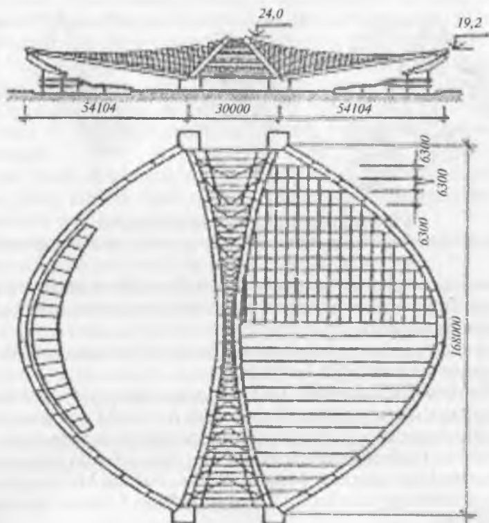
6.4- rasm. Krilatskiydagi (Rossiya) vclopoyga o'yingohi yopmasi.
