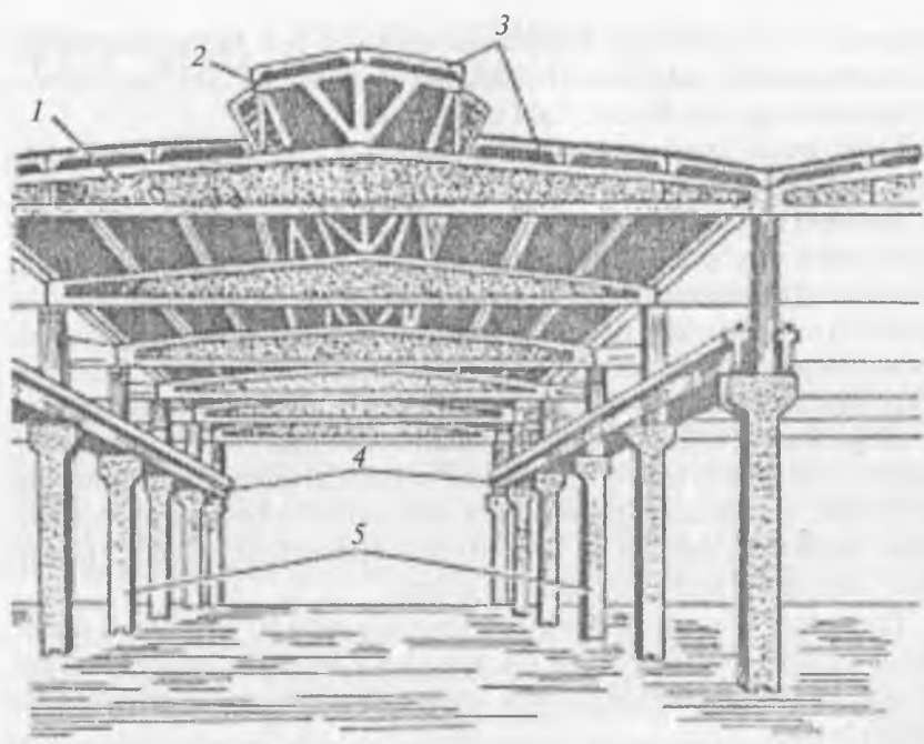
8.1- rasm. Sanoatda qo'llaniladigan temir-beton sinchli konstruksiya: 1 – to'sin; 2 – fonar; 3 – yopma panellar; 4 – kranosti to'sinlar; 5 – ustunlar.
