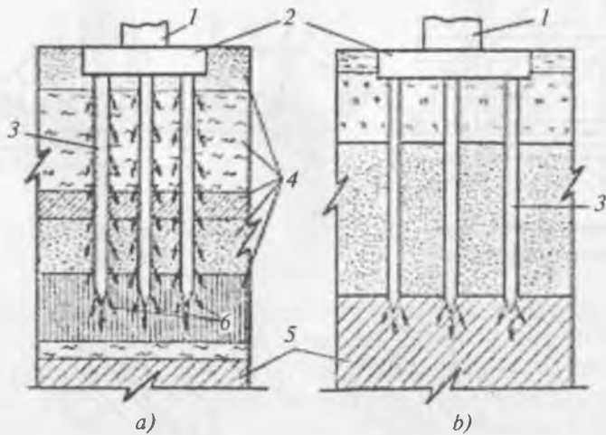
4.7- rasm. Qoziqli poydevorlar:
