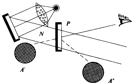
54-rasm. A' — mavhum tasvir; A'' — haqiqiy tasvir.
