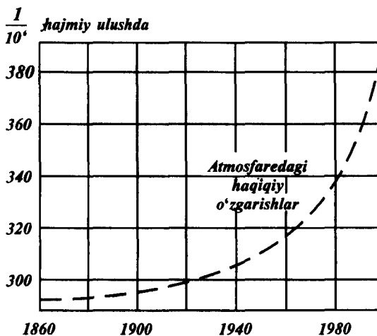
3-rasm. Atmosferada karbonat angidrid konsentratsiyasi.
