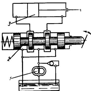
3.45- рasm. Золотникли бошқарувчи дроссел қурилмаси.
