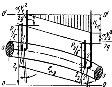
1.38-расм Гидравлик ва пьезометрик қияликлар.
