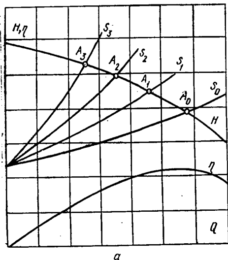
2.14- расм. Дросселнинг очилиш даражасига қараб сарфни бошқаришга доир схема.
