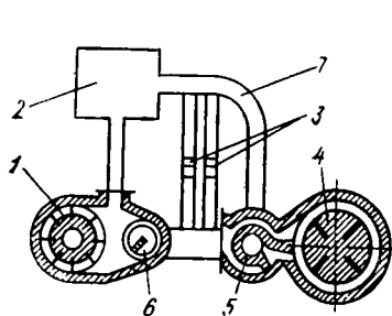
3.1- расм. Ҳажмий гидроузатманинг ишлаш принципи.
