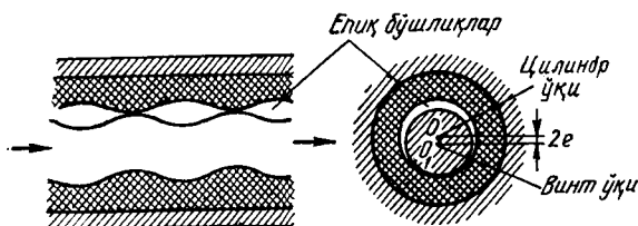
2.39- расм. Цилиндр — винт жуфти.
