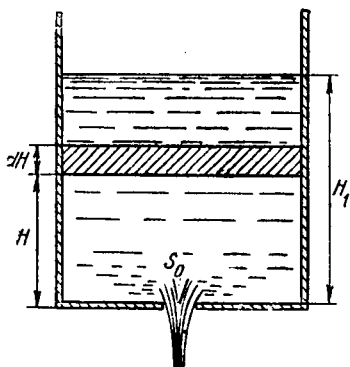
1.81-рasm. Идишнинг суюқлик-дан бўшашига доир чизма.
