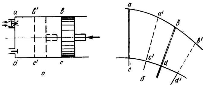
2.27-расм. Ҳажмий насосларнинг ишлаш принципи.
