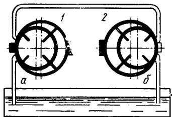
3.26- расм. Роторли ёпиқ ҳажмий гидроузатма.
