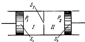
1.84-расм. Дросселларни тушунтиришга онд чизма.
