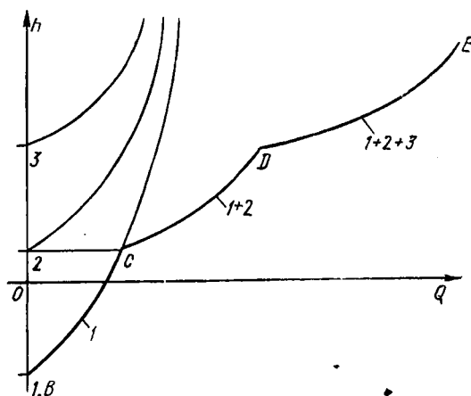
1.95- расм. Тармоқларга бўлинган трубаинг характеристикаси.
