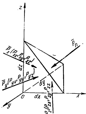
1.34-расм. Реал суюқликларда зўриқиш тензорини тушунтиришга доир чизма.
