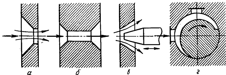
3.43-рasm. Дросселлар.
