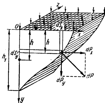
1.24-расм. Эгри сиртга тушадиган босимни тушунтиришга доир чизма.
