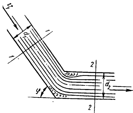
1.68- расм. Тирсак.
