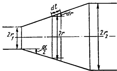
1.74-рasm. Диффузорларда босимнинг камайишини ҳисоблашга доир чизма.
