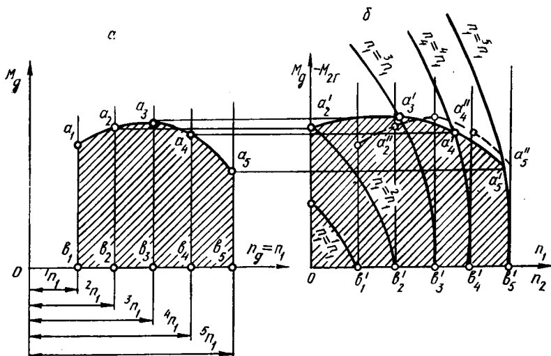
3.13-расм. Гидромуфтанинг двигатель билан биргаликда ишлашига доир.
