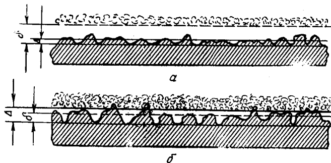
1.57-расм Гидравлик силлиқ ва ғадир-будир трубаларни тўқатиришга доир чизма.
