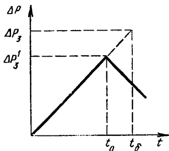
1.104-расм Тўғри ва нотўғри зарбада босимнинг ортиши.
