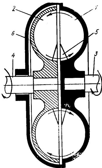
3.5-рasm. Торсиз гидромуфта.
