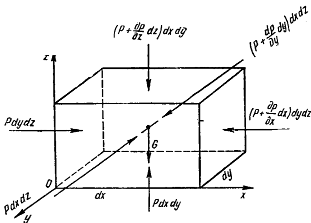
1.6-расм. Суюқликлар мувозанатининг Эйлер тенгламасига доир чизма.
