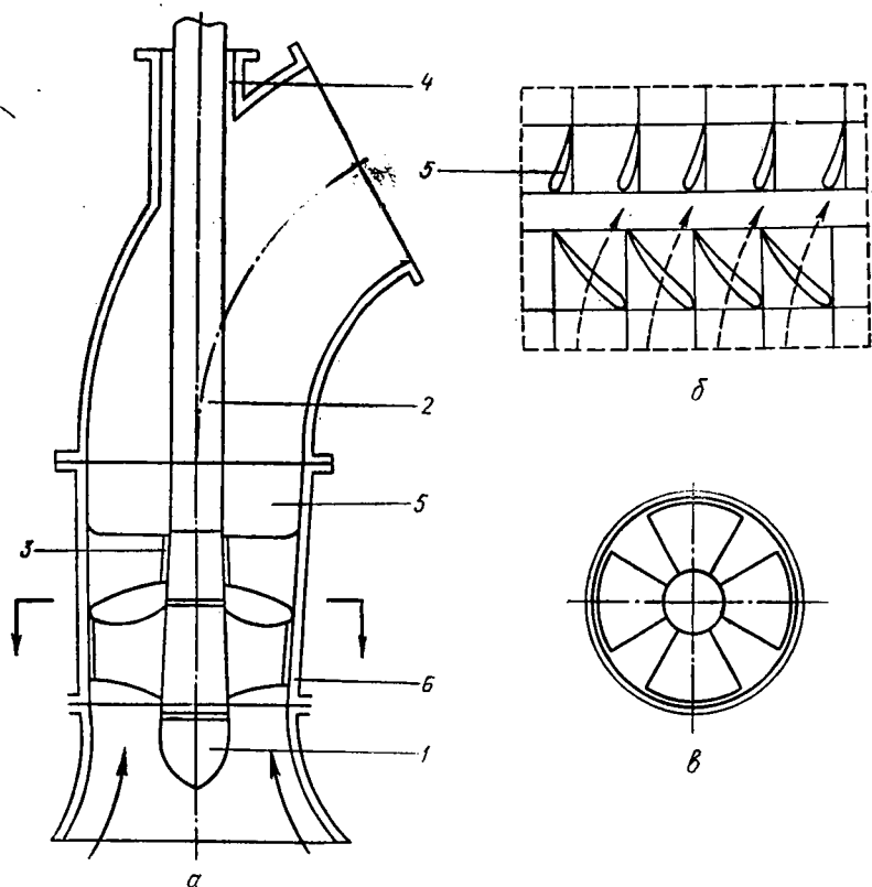
2.11- расм. Ўқий насосларнинг схемаси.
