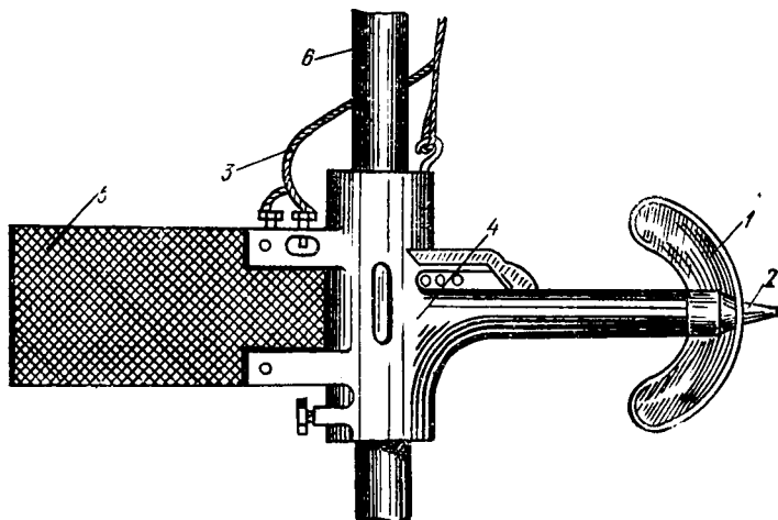
1.42- расм. Пирилдоқ.
