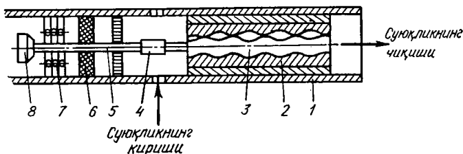
2.38-расм. Чўқтирма бир винтли насосларнинг схемаси.
