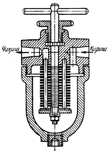
3.47- расм. Пластикали содда филтр.
