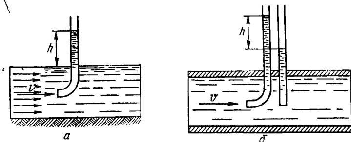
1.44- расм. Тезлик ўлчагич найчалар.
