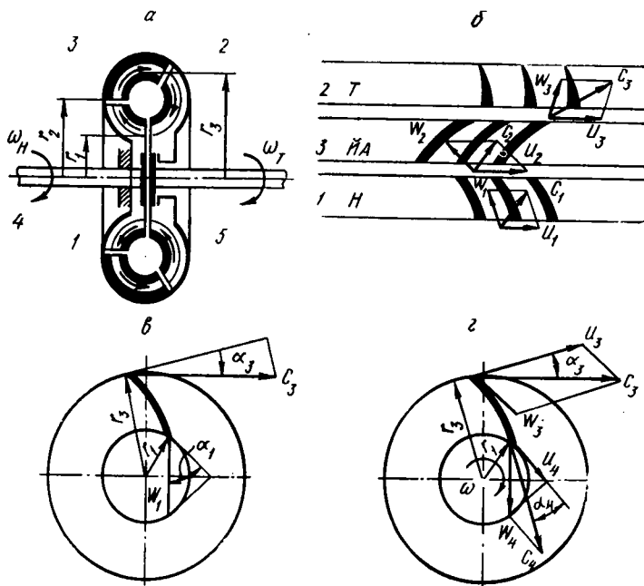
3.15- расм. Гидротрансформаторнинг кенгайтирилган схемаси.
