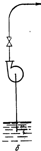
2.14- расм. Дросселнинг очилиш даражасига қараб сарфни бошқаришга доир схема.
