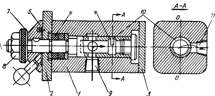
3.44- рasm. Г-77 турдаги бошқариладиган дроссел қурилмаси.
