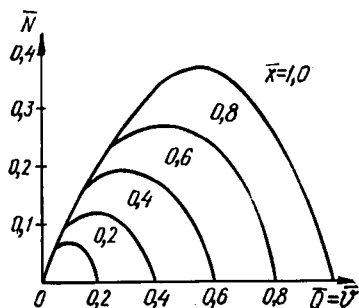
3.53-рasm. Гидроқучайтиргичларда нисбий қувватнинг \bar{Q} га боғлиқлиги графиги.
