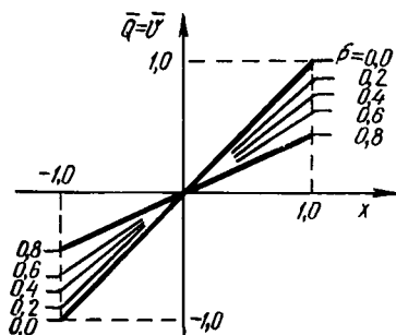
3.50- расм. Гидрокучайтиргичнинг статик характеристикаси ( \bar{Q} ёки \bar{v} ва \bar{x} координатларида).
