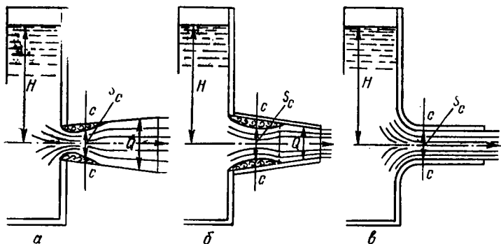
1.80-рasm. а — конуссимон кенгаювчи найча, б — конуссимон тораювчи найча, в — коноидаль найча.
