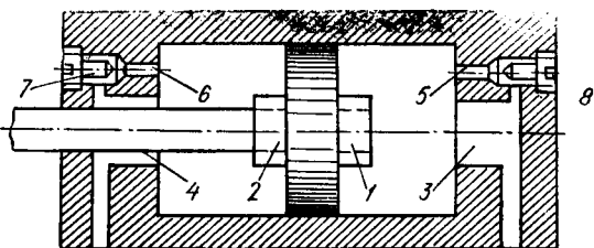
3.32- расм. Икки ҳаракатли куч гидродвигатель.
