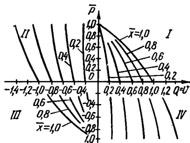
3.49- расм. Гидрокучайтиргичнинг статик характеристикаси ( \bar{p} ва \bar{Q} ёки \bar{x} координатларида).
