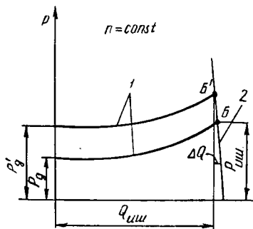
2.47- расм. Ҳажмий насосларнинг трубалар тармоғига ишлаши.
