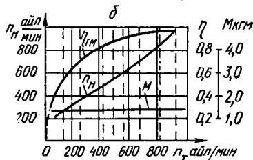
3.12- расм. Универсал характеристикадан фойдаланиб тортиш характеристикасини қуришга доир.
