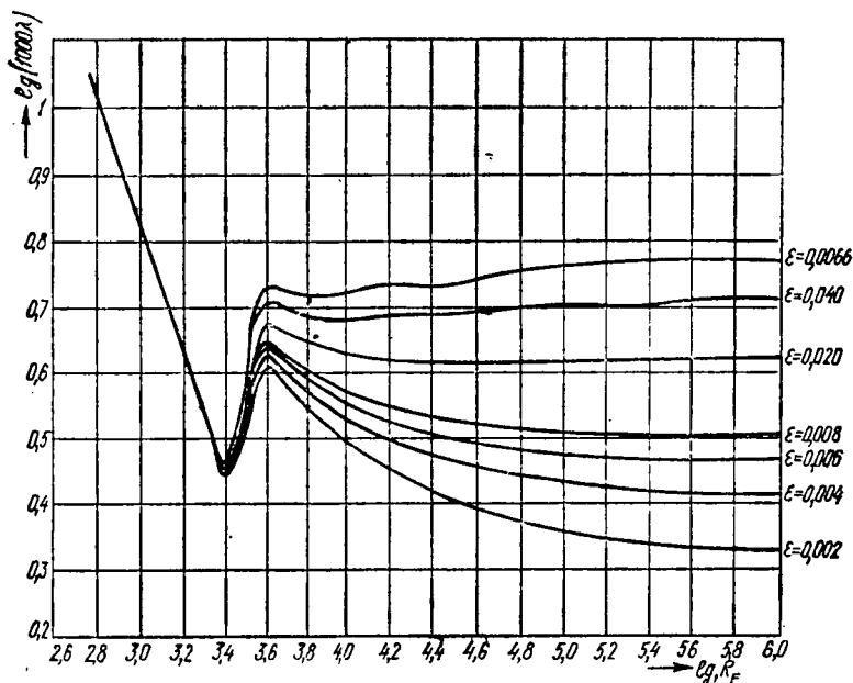
1.60- расм. λ нинг (6.34) формула бўйича ҳисобланган графиги.
