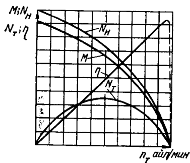
3.9-расм. Гидромурфатинг ташқи характеристикалари.
