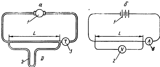
1.97-расм. Суюқлик ва ток ўтказгичларда ўхшашликка доир чизма.
