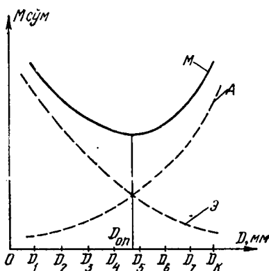
1.88-расм. Тежамли қулай диаметри ҳисоблашга оид чизма.
