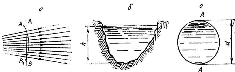
1.30- расм. Ҳаракат кесимиға онд чизма.
