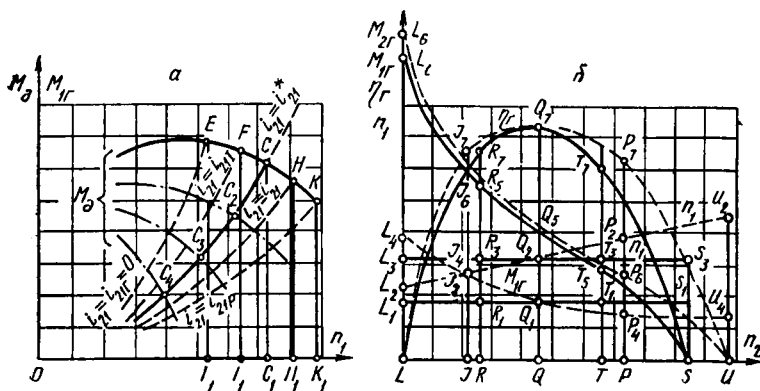
3.20- расм. Двигатель характеристики ва кириш характеристикаси.
