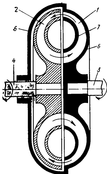
3.3- рasm. 1 гидромурфта.
