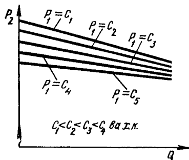
3.42-рasm. Редукцион клапан характеристикаси.
