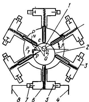
2.42- расм. Радиал-плунжер-ли насос.
