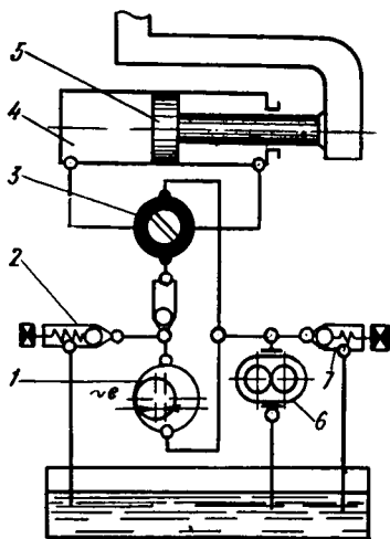
3.28- расм. Ҳажмий бошқариладиган илгарилама-қайта гидроузатма.
