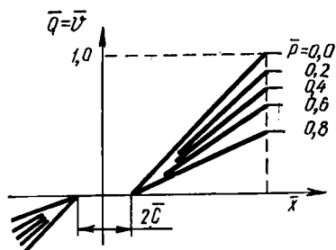
3.52-рasm. Мусбат беркитишли золотник қўлланилган гидроқучайтиргичларда статик характеристика ( \bar{Q} ёки \bar{v} ва \bar{x} координатларида).
