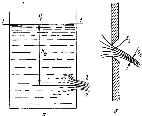
1.77-расм. Суюқликнинг тешиклардан оқиб кетишга доир чизма.
