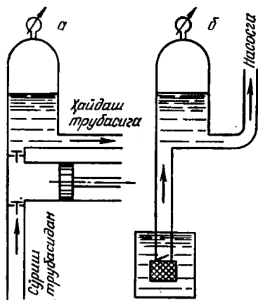
2.34- расм. Ҳаво қалпоғининг ҳайдаш ва сўриш трубасига ўрнатиш схемаси.
