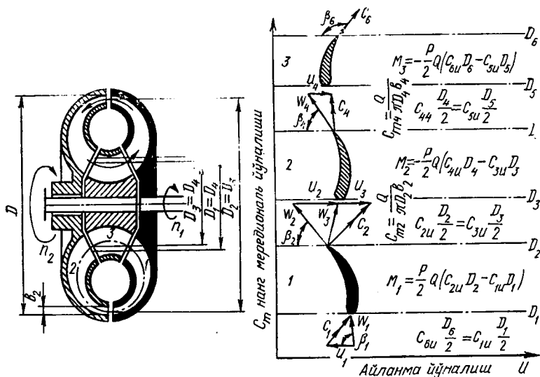
3.14- расм. Гидротрансформатор.
