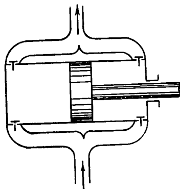
2.29-расм. Икки ҳаракатли поршенли насоснинг принципал схемаси.
