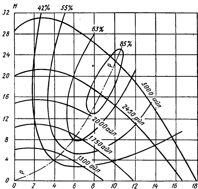
2.9- расм. Марказдан қочма насосларнинг универсал характери-стикаси.
