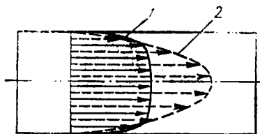
1.56- расм. Турбулент-ва ламинар ҳаракатда тезлик эпюралари.
