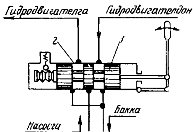
3.34- расм. Золотникли тақсимлагич-лар.
