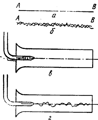
1.46-рasm. Ламинар ва турбулент ҳаракатга оид чизма.
