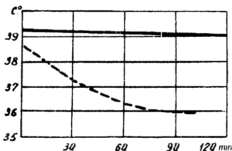
46-rasm. Sun'iy yo'l bilan sovutilgan normal mushuk (uzluksiz chiziq) va desimpatizatsiya qilingan mushuk (uzuq-uzuq chiziq)ning gavda harorati (U.Kennondan)
