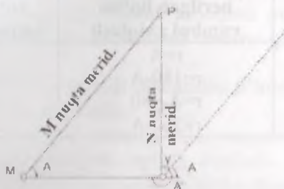
1.7.-rasm. Oriyentirlash burchaklari o'rtasidagi munosabat
