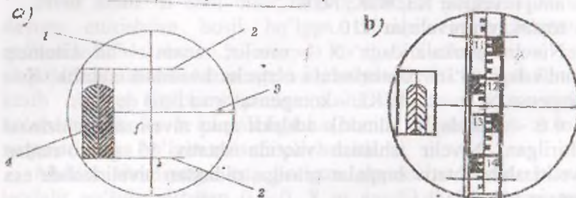
6.7-rasm. 1-vertikal ip; 2-dalnomer iplari; 3- o'rta ip; 4- silindrik adilak pufakchasinig uchlari ,bir-biriga to'g'ri keltirilgan (kontakt) holati; 5) qarash trubasida reyka tasviri
