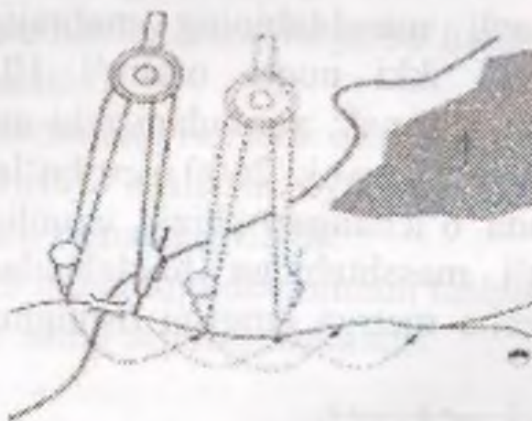
3.2- rasm. Mikroo'lchash sirkuli yordamida chiziq uzunligini aniqlash
