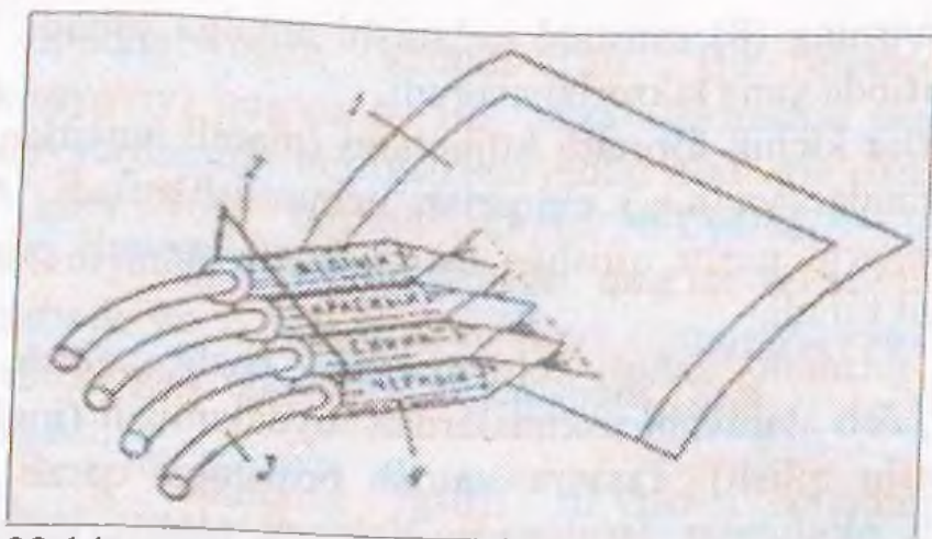
22.14-rasm. Oqimli (struyali) printyerni tuzilishi 1 – qog'oz, 2 – bosma kallak, 3 – siyoh eritmalari keladigan shlanglar, 4 – purkaluvchi moslamalar
