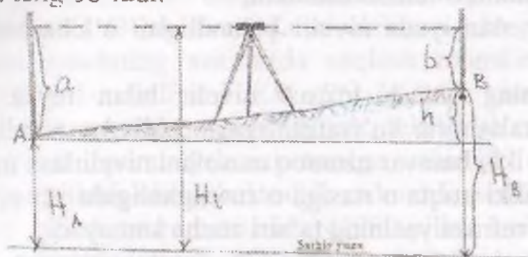
6.11-rasm. O'rtadan nivelirlash
