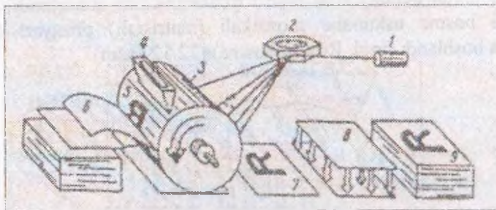
22.13-rasm. Elektronografik (lazyer) printyerlarning ishlash chizmasi.
