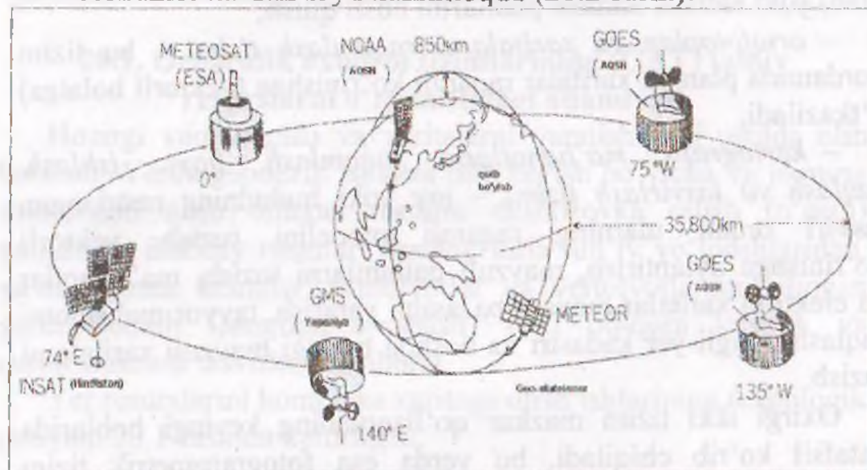
20.3-rasm. Yer shari atrofida harakatlanayotgan sun'iy yo'ldoshlar
