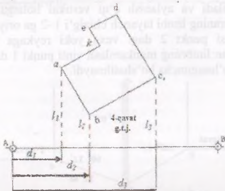
6.2-rasm. Perpendikulyar usul
