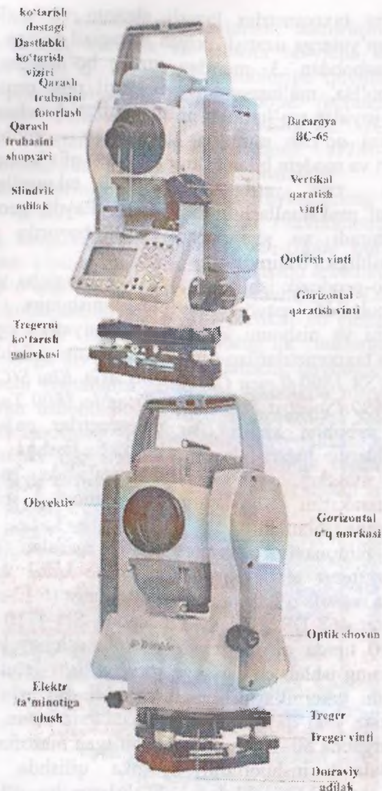
6.13-rasm. Elektron taxometr
