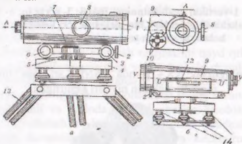
6.6-rasm. H3 niveliri tuzilishi
