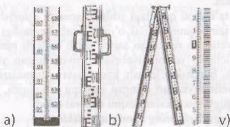
6.9-rasm. Nivelirlash reykalari
