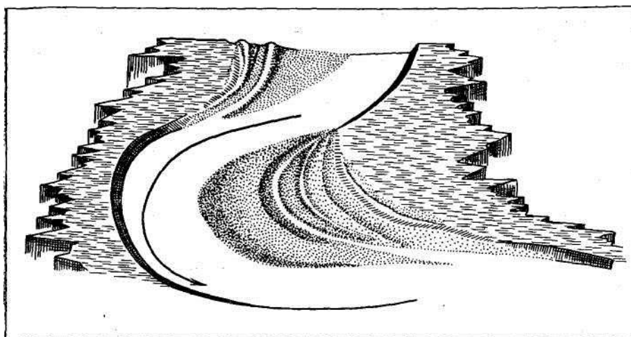
Рис.10. Растущая прирусловая отмель у выпуклого участка берега (по А.Р.Ярмухамедова)
