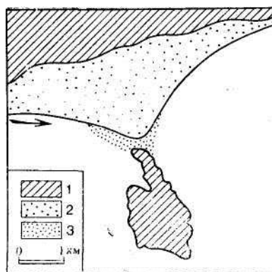
Рис. 24. Остров Габо и формирующаяся в его волновой тени перейма : 1 — коренная суша; 2 — надводная аккумулятивная форма; 3 — ее подводное продолжение
