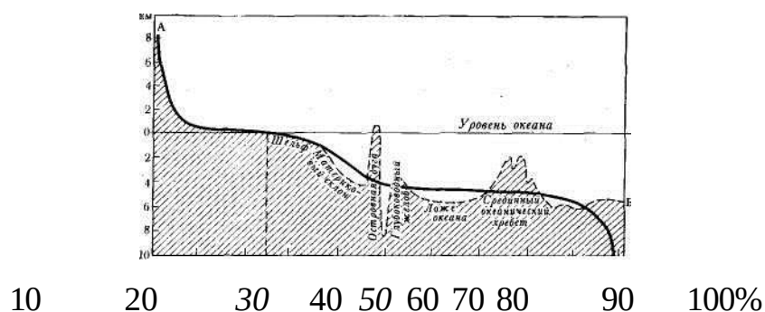
Рис. 1. Гипсографическая кривая (А) и обобщенный профиль дна океана (Б)
