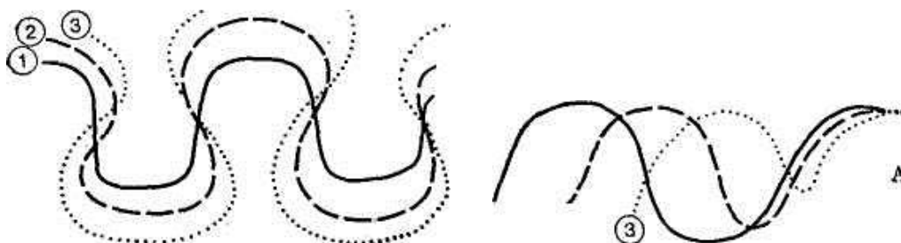
Рис. 12. Переформирование излучин: А — сжатие и «стачивание» колена меандры; Б — образование омеговидных меандр и «пережимы» их шеек вследствие размыва вогнутых берегов; 1, 2, 3 — последовательные положения русла быстро мелеет в результате аккумуляции наносов, остальная сохраняется ряд лет сначала в виде затона (изолированного от меженного течения только в верхней части), а затем в виде старицы — пойменного озера.
