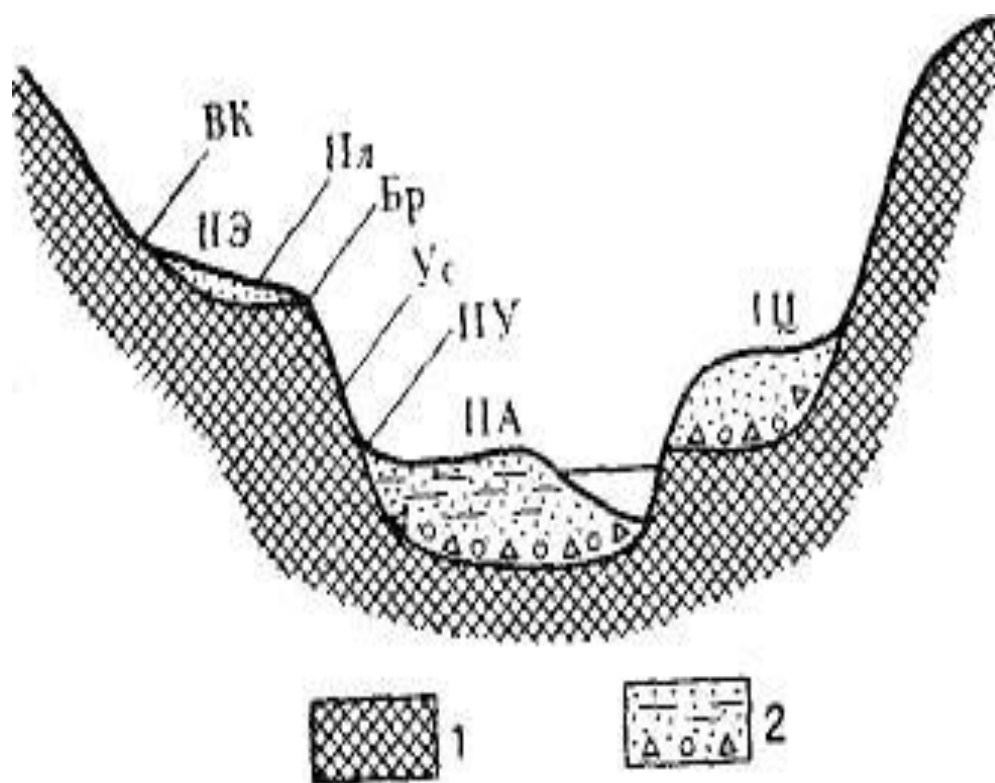
Рис. 15. Схема строения речных террас:
