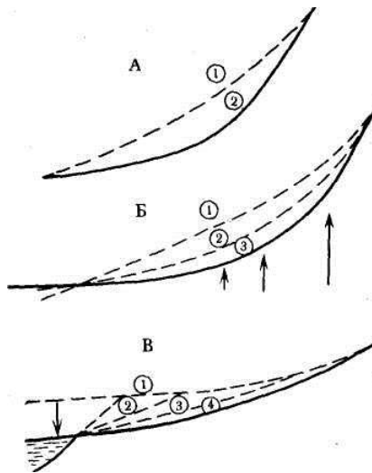
Рис. 14. Врезание реки и образование хордовых террас вследствие увеличения расхода воды (А), в результате преимущественного поднятия верховьев речного бассейна (Б) (длина направленных вверх стрелок соответствует относительным величинам скорости поднятия), и при пониженном уровне моря (В), имеющего относительно крутосклонный подводный береговой склон (стрелка указывает направление изменения уровня моря); 1, 2, 3, 4 — последовательные положения продольного профиля
