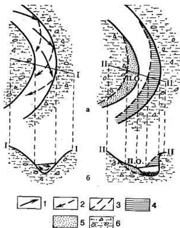
Рис 9. Схема образования приустьевой отмели:
