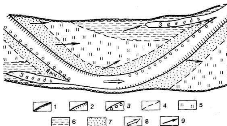
Рис. 13. Схема массива поймы (по Н. И. Маккавееву):
