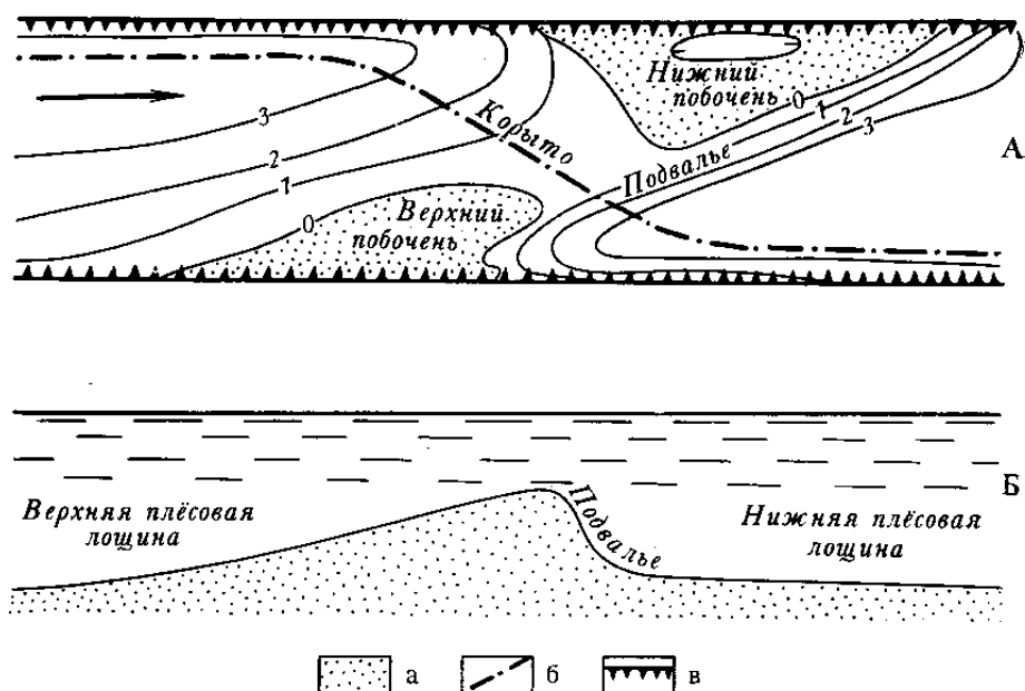
Рис.5. Элементы переката: А - план в изобатах, Б – профиль по линии стрежня (по Н.И.Маккавееву); а-поверхность побочней, возмывающихся над меженным уровнем воды, б- линии стрежня, в- берега меженного русла, 1, 2, 3 -изобаты. изгибы, образованные рекой
