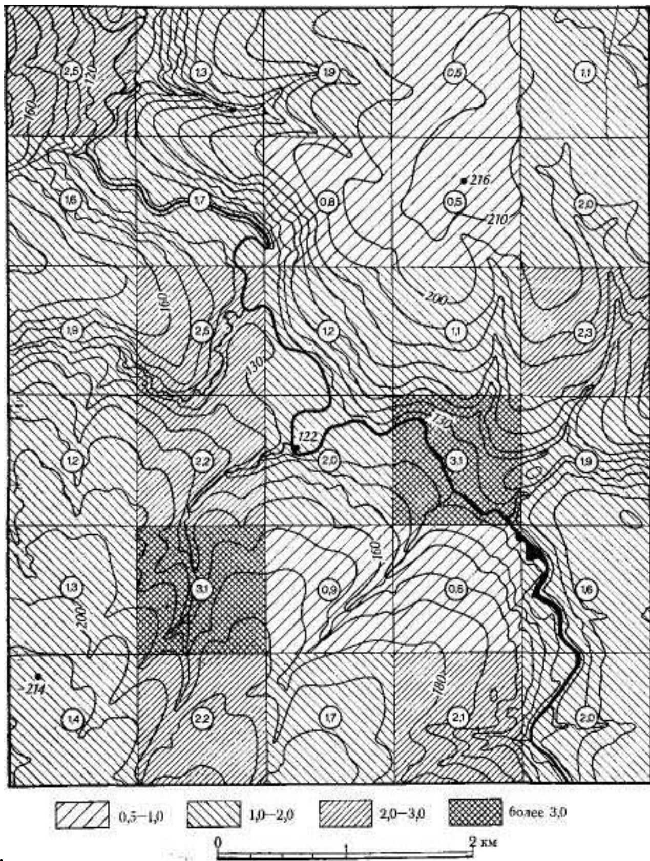
Рис. 2. Картограмма густоты долинно-балочной сети (в километрах на 1 км 2 , по А. И. Спиридонову)
