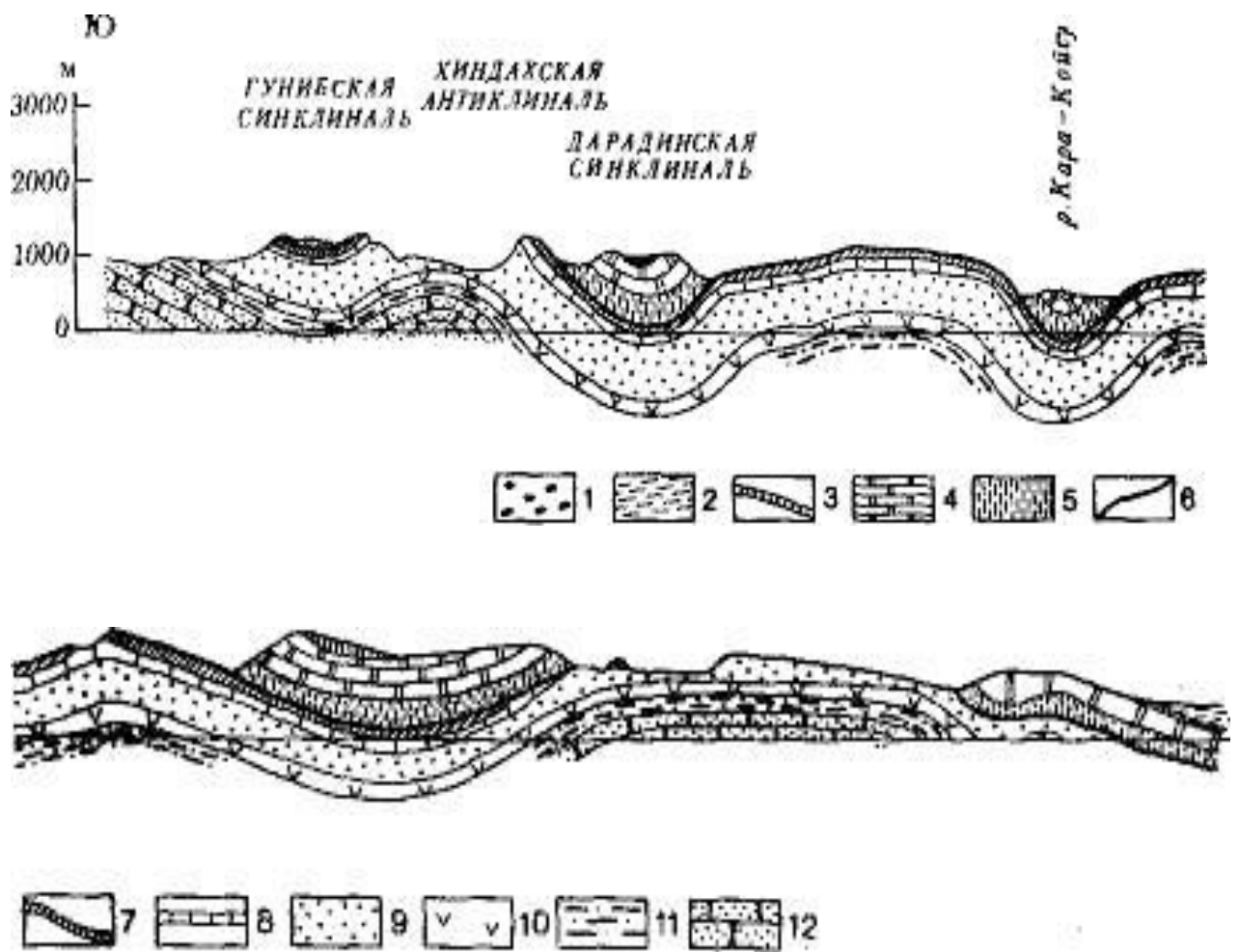
Рис.4. Структурно-денудационный рельеф Известнякового Дагестана (по А. Е. Кривоуцкому): (1-песчано-глинистые породы миоцена; 2 - глинистые нестойкие породы верхнего палеогена - нижнего миоцена (Майкон); 3 - карбонатные породы эоцена и палеоцена; 4 - стойкие известняки позднего мела; 5 - малостойкие песчано-глинистые породы альба — верхнего баррема; 6-основной бронирующий горизонт - известняки нижнего баррема; 7 -алевролиты, песчаники и известняки готерива; 8 - стойкие известняки валанжина и верхней юры; 9 - аргиллиты и алевролиты бата и верхнего байоса; 10 - песчаники и аргиллиты нижнего байоса; 11 - нестойкие аргиллиты и алевролиты верхнего аалена; 12 - повышенной стойкости песчаники нижней юры хребты северного склона Большого Кавказа и др.).
