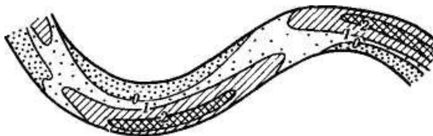
Рис. 6. Распределение плёсов и перекатов у меандрирующих рек: а — поверхность побочной, возвышающаяся над неженным уровнем воды; б — тела перекатов; в — плёсовые лощины (густота штриховки пропорциональна глубине); 0, 1, 2,— изобаты
