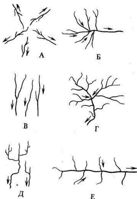
Рис 19. Типы речной сети: А-радиальный центробежный; Б – радиальный центростремительный; В - параллельный; Г — древовидный; Д — ортогональный решетчатый; Е — перистый
