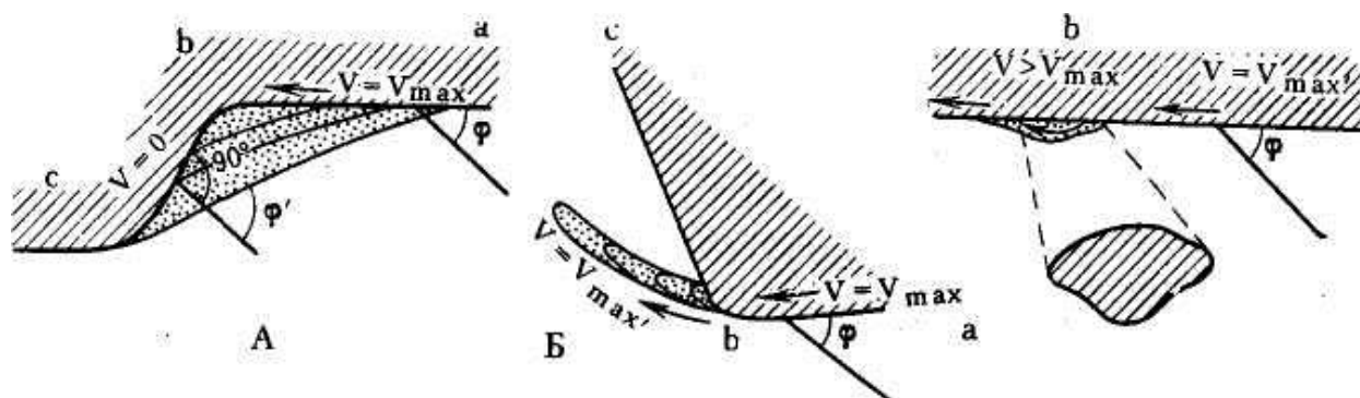
Рис.23. Схема образования простейших береговых аккумулятивных форм (по Якубова Ж.Х.): А — заполнение входящего угла контура берега, Б — огибание выступа берега, В — внешняя блокировка
