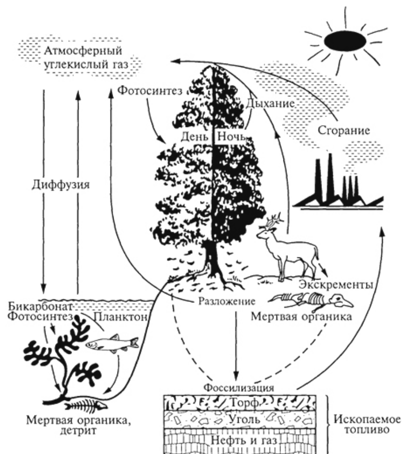
Рис. 3. Круговорот углерода (J.Smith,
