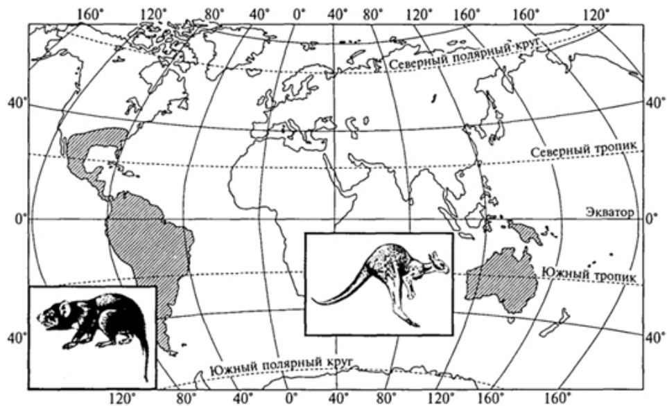
Рис. 49. Дизъюнктивный ареал сумчатых млекопитающих (Г. М.Абдурахманов и др., 2001)
