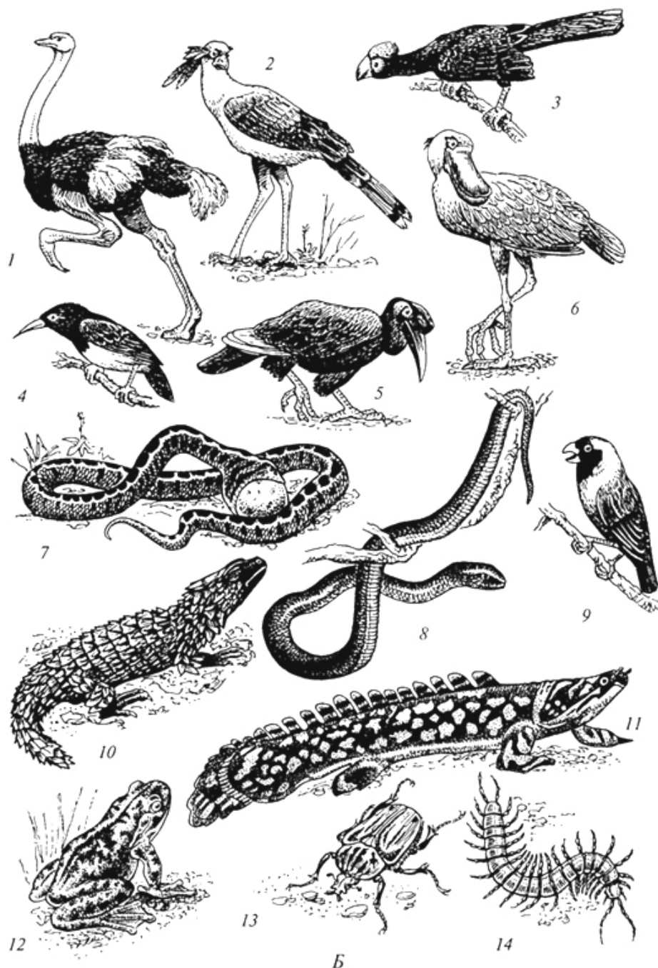
Рис. 56 б. Характерные представители фауны Эфиопской области (Г. М. Абдурахманов и др., 2001): Б -от птиц до насекомых: 1 - двупалый страус; 2 -птица-секретарь; 3 -туруко; 4 -нектарница; 5- рогатый ворон; 6 -китоглав; 7-яичная змея; 8 -зеленая мамба; 9 -красноклювый ткачик; 10 -поясная ящерица; 11 - многопер; 12 -веслоногая лягушка; 13 -жук-голиаф; 14 -сколопендра
