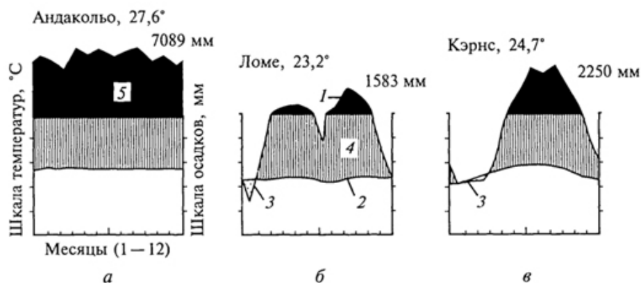
Рис. 21. Климадиаграммы
