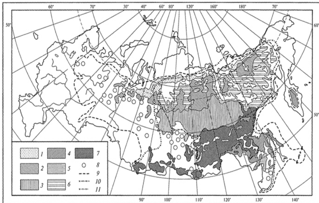
Рис. 28. Распространение лиственных лесов в Северной Евразии (В.Б.Сочава, 1956): 1 - предтундровые лиственные редколесья; 2 -северотаежные лиственные леса; 3- среднетаежные лиственные леса; 4 -среднетаежные багульниковые и сфагновые лиственные леса (мари); 5 - южнатаежные лиственные леса; 6 -горные редкостойные лиственные леса; 7 -горные таежные лиственные леса, местами кедрово-лиственные; 8 -лиственные леса на небольших площадях; 9 -обобщенная граница распространения всех видов лиственницы; 10 -восточная граница распространения лиственницы сибирской; 11 - изолиния показателя средней континентальности климата (по Н.Н.Иванову)
