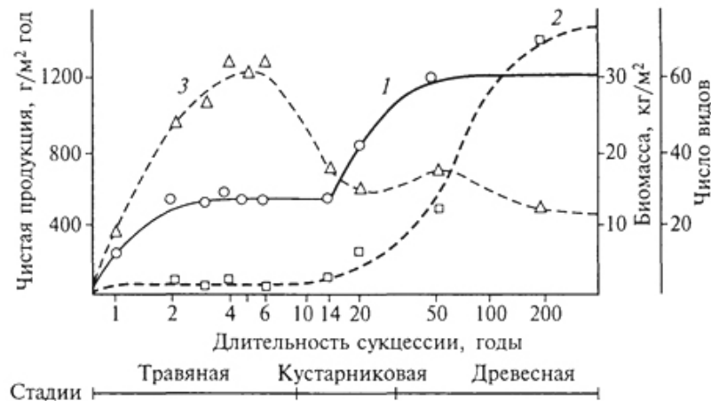
Рис. 18. Изменение чистой продукции (1), биомассы (2) и видового разнообразия (3) дубово-соснового леса (Брукхейвен, штат Нью-Йорк) в ходе сукцессии (Р.Уиттекер, 1980): 1 - чистая продукция увеличивается до стабильного уровня в травяной стадии, затем, поскольку в сообщества внедряются деревья, вновь возрастает до уровня, который может сохраняться в климаксе; 2- биомасса низка в травяных стадиях, но быстро увеличивается при накоплении древесных тканей кустарников и деревьев; климаксовый уровень биомассы, вероятно, может быть достигнут не ранее чем через 400 лет; 3 -видовое разнообразие (число видов на площади 0,3 га) возрастает в последних травяных стадиях, далее снижается в кустарниковых стадиях (14-20 лет), несколько увеличивается в молодом лесу (50 лет) и вновь уменьшается в климаксе (время дано в логарифмическом масштабе, что позволяет расширить ранние и сжать поздние стадии сукцессии)
