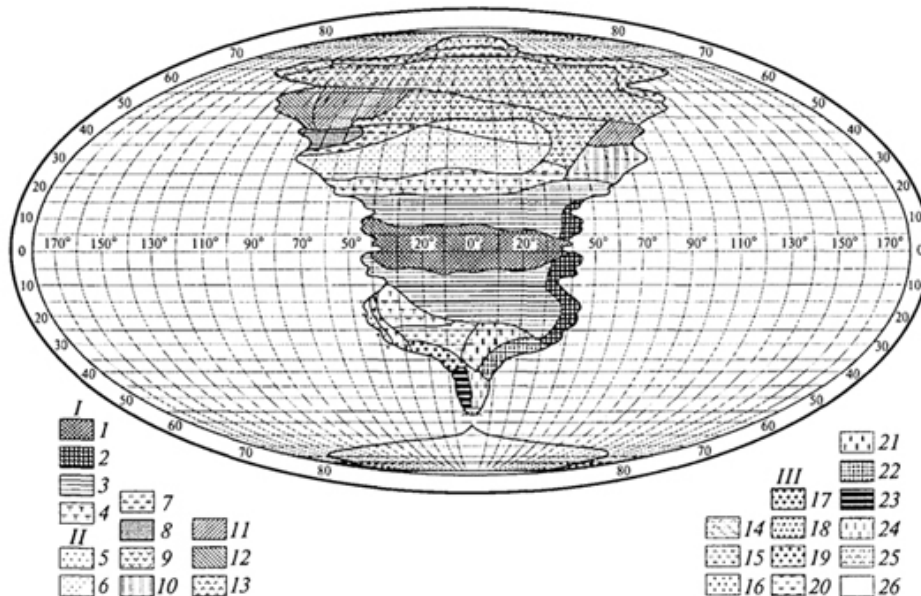
Рис. 23. Распределение растительности на "идеальном" континенте, составленное К.Троллем (Г.Вальтер, 1968): I. Тропические зоны: 1 -экваториальный дождевой лес; 2- тропические дождевые леса; 3 -тропические саванны (влажные саванны) и листопадные леса; 4 -тропические сухие саванны и колючие леса. II. Внетропические зоны северного полушария: 5-сухие пустыни; 6- холодные внутриматериковые пустыни; 7 - субтропические зимнезеленые степи; 8 -жестколистные леса и кустарники; 9 -зона степей с холодной зимой; 10- зона влажных муссонных и лавровых лесов; 11- летнезеленые леса; 12 - океанические летнезеленые листопадные и лавровые леса; 13 -бореальные хвойные леса; 14 -бореальные березовые леса; 15 - субарктические тундры; 16-высокоарктические тундры. III. Внетропические зоны южного полушария: 17 -прибрежные пустыни; 18 -пустыни, развитые в пределах пояса "Гаруа"; 19- жестколистные леса и кустарники; 20- субтропические колючие степи; 21- субтропические злаковники; 22- субтропические дождевые леса; 23 -умеренно холодные дождевые леса; 24 -степи Патагонии и Новой Зеландии; 25 -субантарктические туссоковые луга и болота; 26- антарктическая область материкового льда
