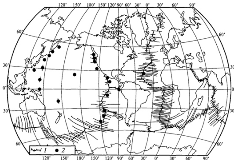
Рис. 90. Зоны разломов (1) и районы обнаружения сообществ хемобиоса (2) в Мировом океане (А.М.Сагалевиц, Л.И.Москалев, 1991)
