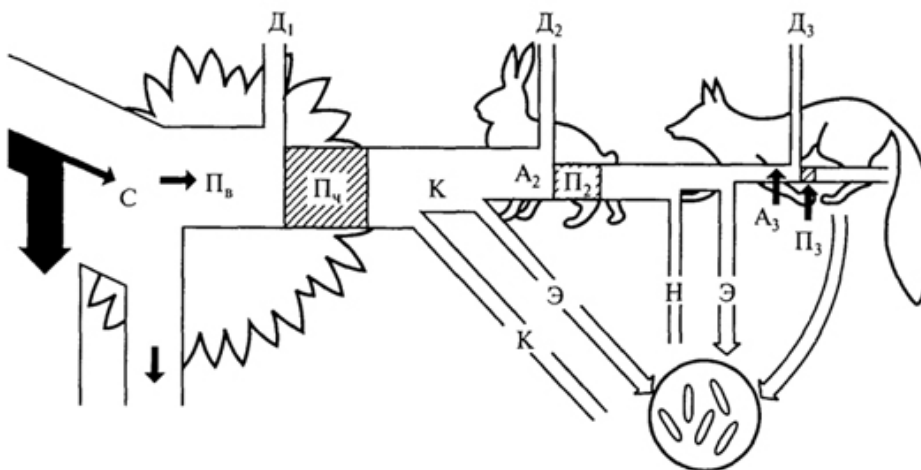
Рис. 2. Поток энергии
