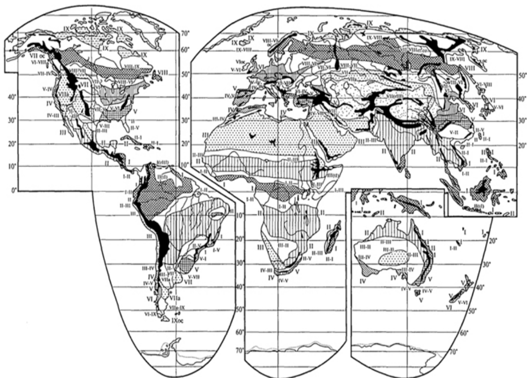
Рис. 60. Зональные типы биомов суши (Г. Вальтер, 1985): I - вечнозеленые тропические дождевые леса, почти без сезонных аспектов; II - тропические листопадные леса или саванны; III - субтропическая пустынная растительность; IV - субтропические склерофильные леса и кустарники, чувствительные к морозам; V - умеренные вечнозеленые леса, чувствительные к морозам; VI - широколиственные листопадные леса, устойчивые к морозам; VII - степи и пустыни областей с холодной зимой, устойчивые к морозам; VIII - бореальные хвойные леса (тайга); IX - тундры, обычно на многолетне-мерзлых почвах; залитые контуры - высокогорная растительность
