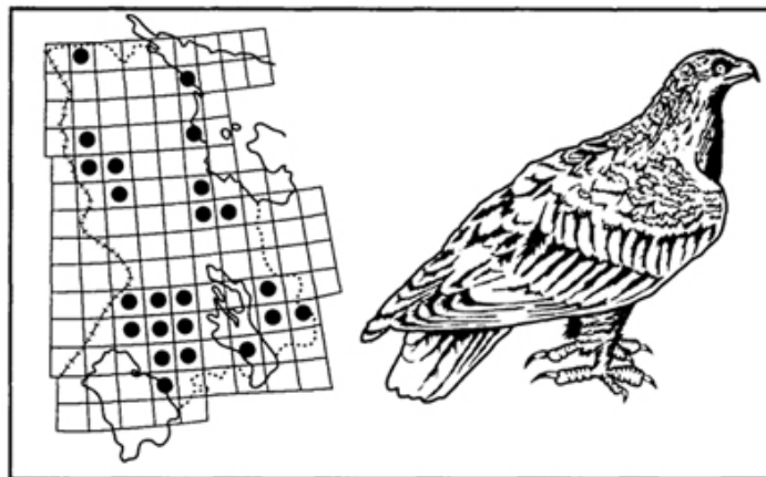
Рис. 32. Ареал беркута. Редкий гнездящийся и зимующий вид. Сетка квадратов со сторонами 50×60 км 2 (Красная книга Карелии, 1995)
