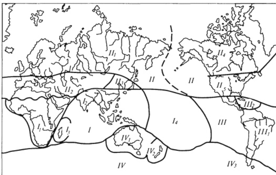
Рис. 55. Фаунистическое
