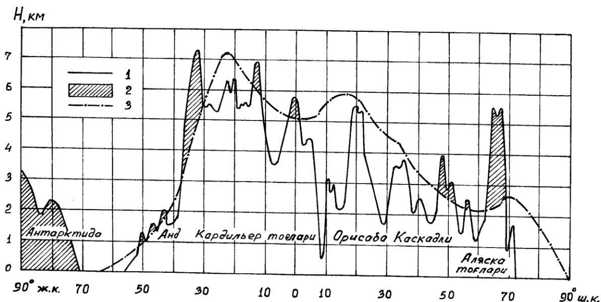
45-расм. Қор чизиғи баландлигининг Анд ва Кордильер тоғлари орқали ўтказилган кенгликлар бўйича ўзгариши (В.М.Котляков маълумоти). 1-ер юзаси рельефи, 2-музлик қоплаган ерлар, 3-қор чизиғи.
