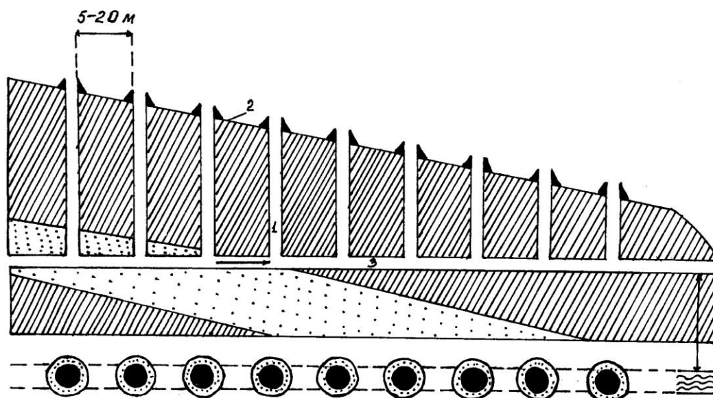
6-расм, а. Кориз-суғоришда ер ости сувларидан фойдаланишга имкон беради (А.Муҳаммаджанов). 1-қудуқ, 2-ер сирти, 3-ер ости сув йўли, → ер ости сувларининг ҳаракат йўналиши.
