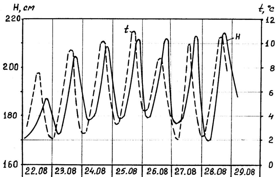
48-расм. Зарафшон дарёсининг музликка яқин қисмида сув сатҳи (H) ва ҳарорати (t) нинг тебраниши (А.К. Давидов маълумоти).
