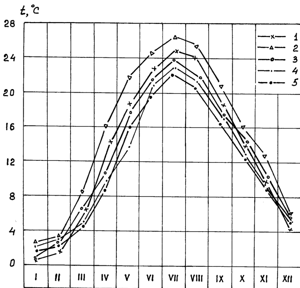
41 –расм. Сув омборларида сув ҳароратининг йил давомида ўзгариши (А.М.Никитин бўйича). Сув омборлари: 1-Қайроққум (Қайроққум шаҳри ёнида), 2-Чимқўрғон, 3-Каттақўрғон, 4-Чорбоғ, 5-Ўртатўқай.
