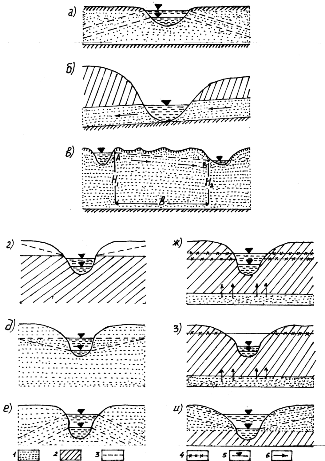
44-расм. Грунт сувларининг дарё оқими ҳисобига тўйиниши (а,б,в), грунт ҳамда дарё сувларининг гидравлик боғлиқлиги (д,е,ж,з,и). 1—сув ўтказувчи қатламлар, 2—сув ўтказмайдиган қатламлар, 3—грунт сувлари сатҳи, 4—босимли сувларнинг пьезометрик сатҳи, 5—дарё суви сатҳи, 6—ер ости сувларининг ҳаракат йўналиши.
