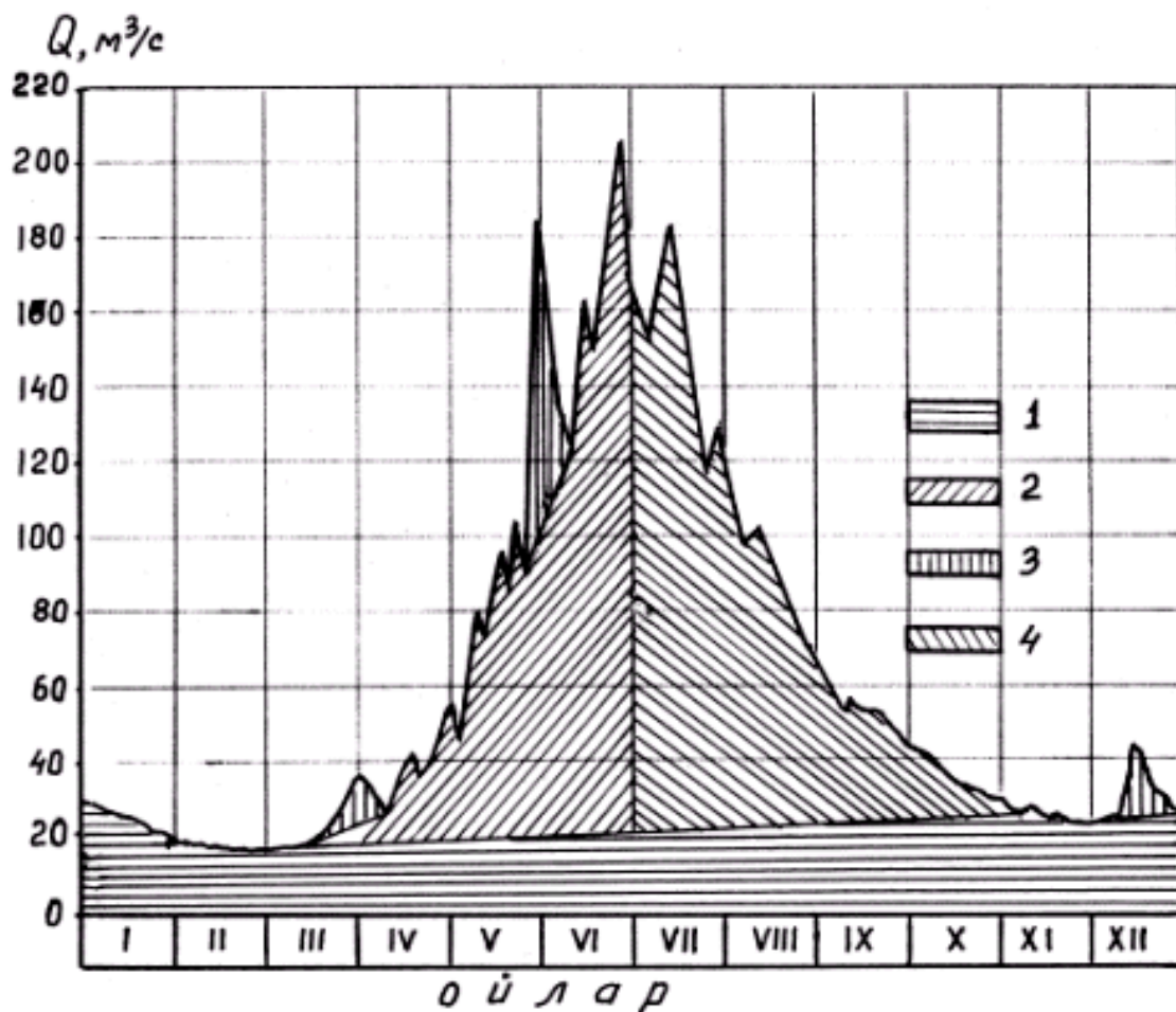
22-расм. Дарё оқими гидрографини вертикал бўлақларга ажратиш.
