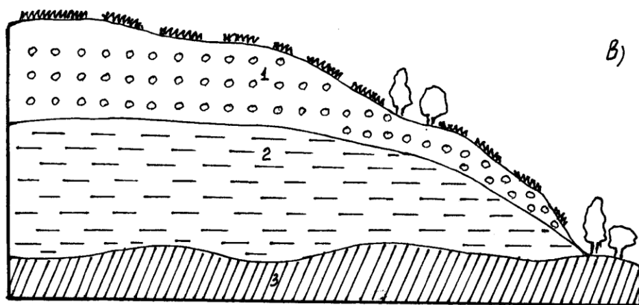
42-расм. Грунт сувларининг жойлашиши (Д.С.Иброҳимов ва А.Н.Султонхўжаевлар бўйича). а-грунт сувлари ҳавзаси, б,в-грунт сувлари оқими. 1-сув ўтказувчи қатлам, 2-суван қатлам, 3-сув ўтказмайдиган қатлам.
