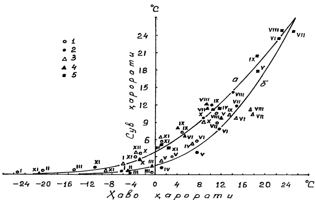
36-расм. Кўллар суви ҳароратининг ҳаво ҳарорати билан боғлиқлиги (А.М.Никитин бўйича). а-совушда, б-иссишда; Кўллар: 1-Яшилкўл, 2-Сарез, 3-Искандаркўл, 5-Судочье.
