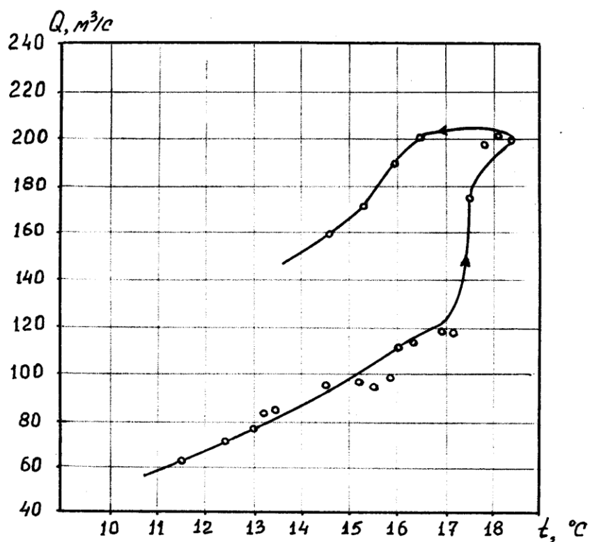
47-расм. Сельдара дарёси (Мўғсув дарёси ирмоғи) ўртача деакадали сув сарфларининг Олтинмозор метеорологик станциясида кузатишган ҳаво ҳарорати билан боғлиқлиги
