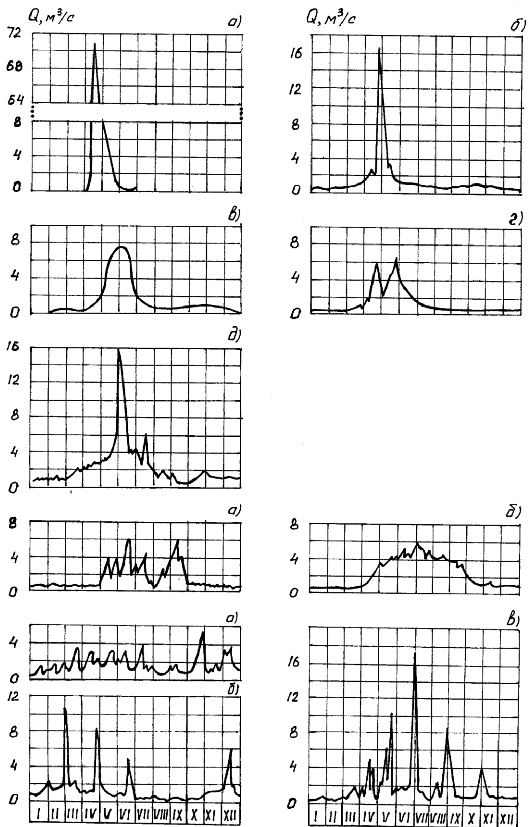
16-расм. Дарёларнинг сув режими даврлари бўйича таснифи.
