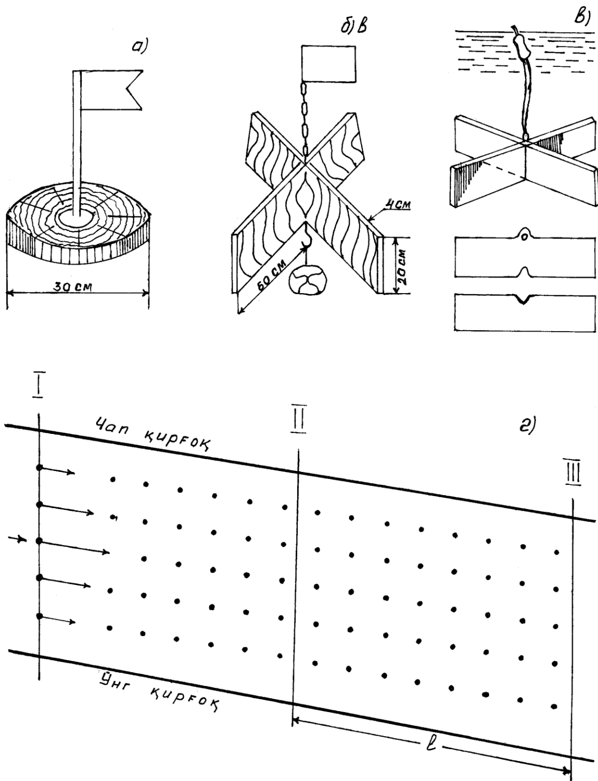
18-расм. Тезликни қалқималар ёрдамида аниқлаш(г). а,б-юза қалқималар, в-чуқурлик қалқимаси.
