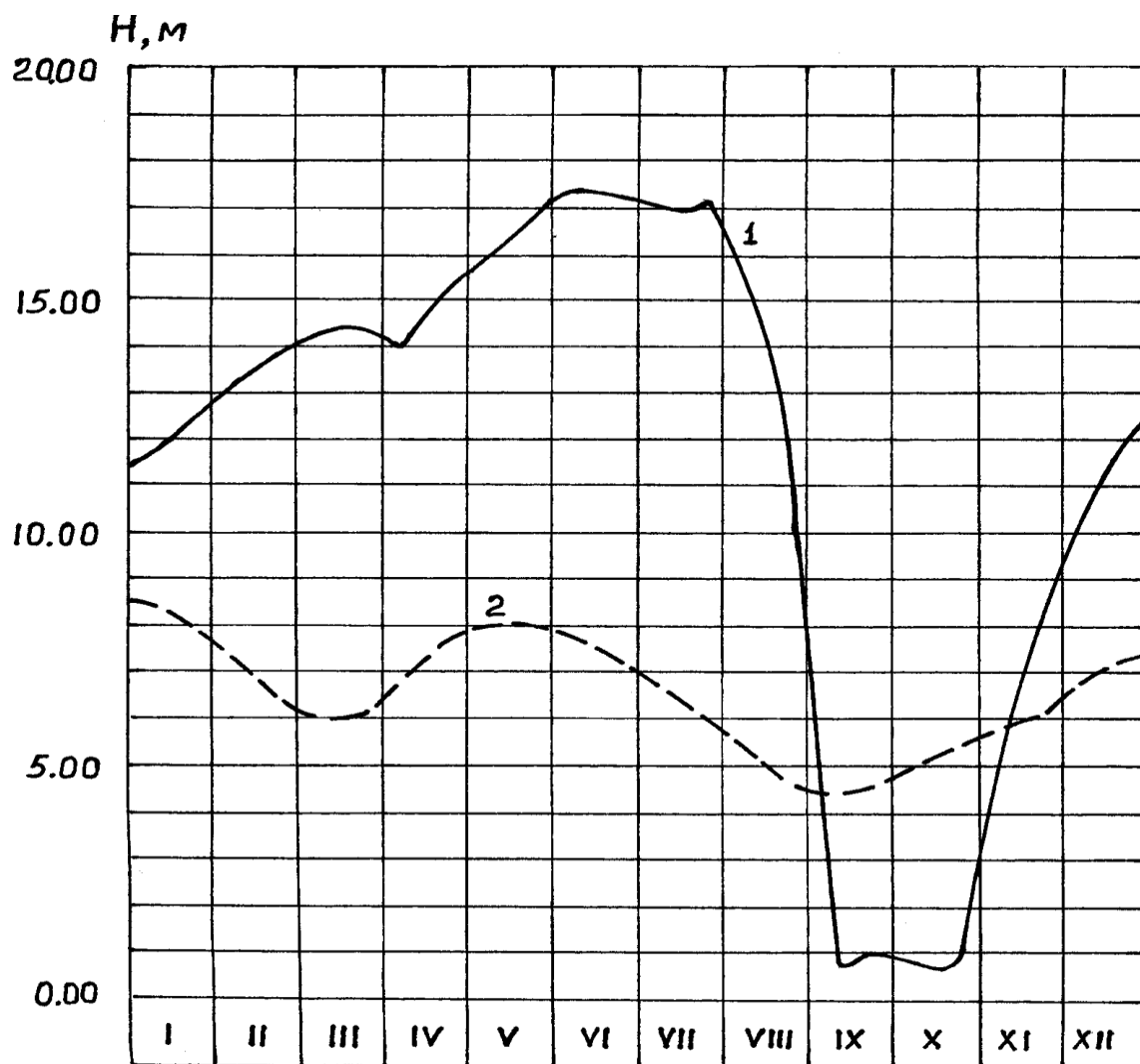
40-рассм. Сув омборларида сув сатҳининг йил давомида ўзгариши. 1-Каттақұрған сув омбори (1958 й.), 2-Қайроққұм сув омбори (1961 й.)
