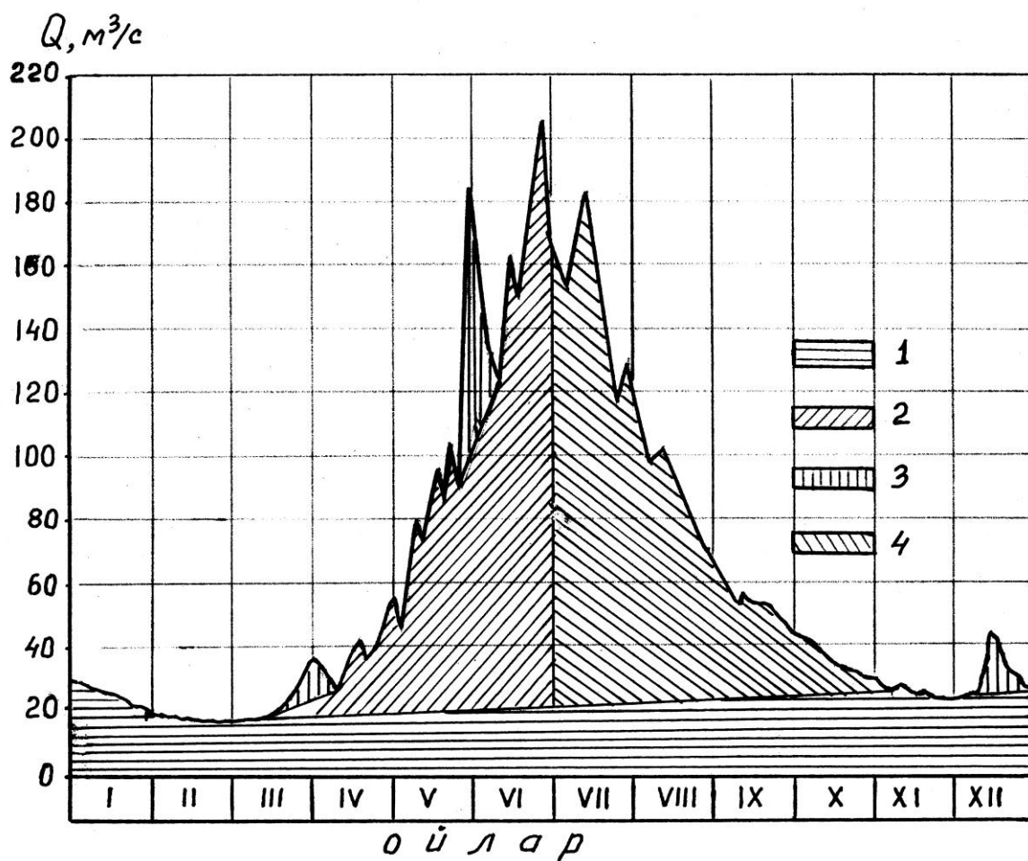
22-расм. Дарё оқими гидрографи вертикал бўлақларга ажратиш.
