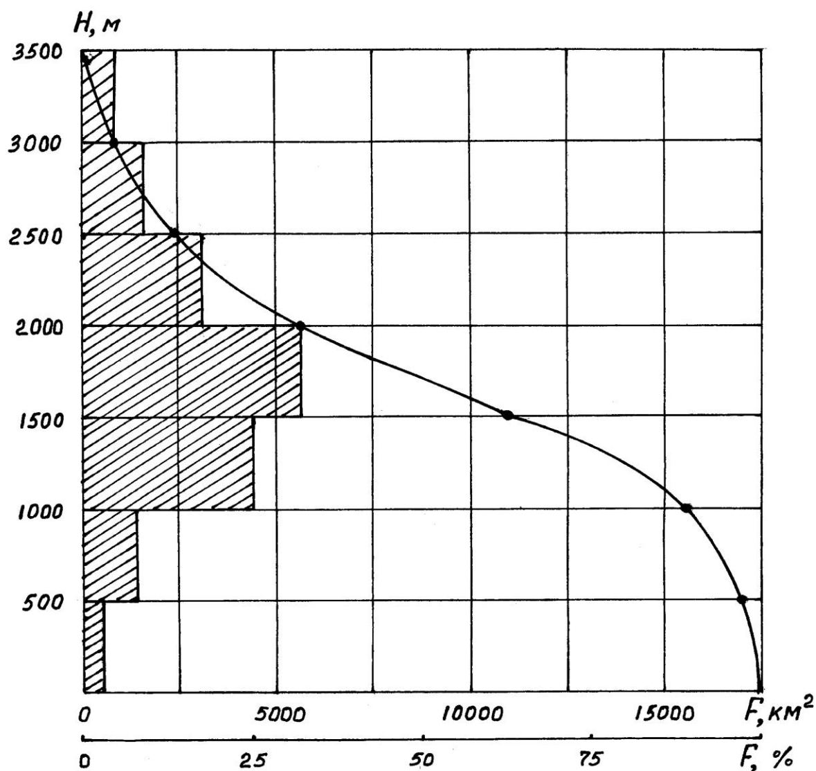
10-расм. Дарё ҳавзасининг гипсографик эгри чизиги.
