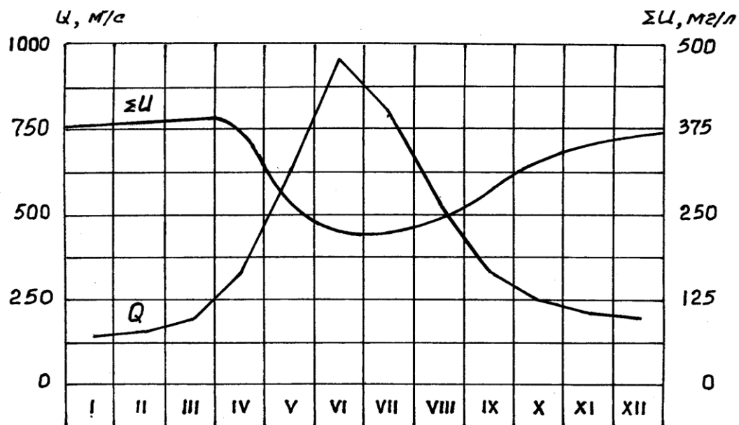
29-расм. Норин дарёси (Ўчқўргон яқинида) ўртача кўп йиллик сув сарфи ва минераллашувининг йил давомида ўзгариши.
