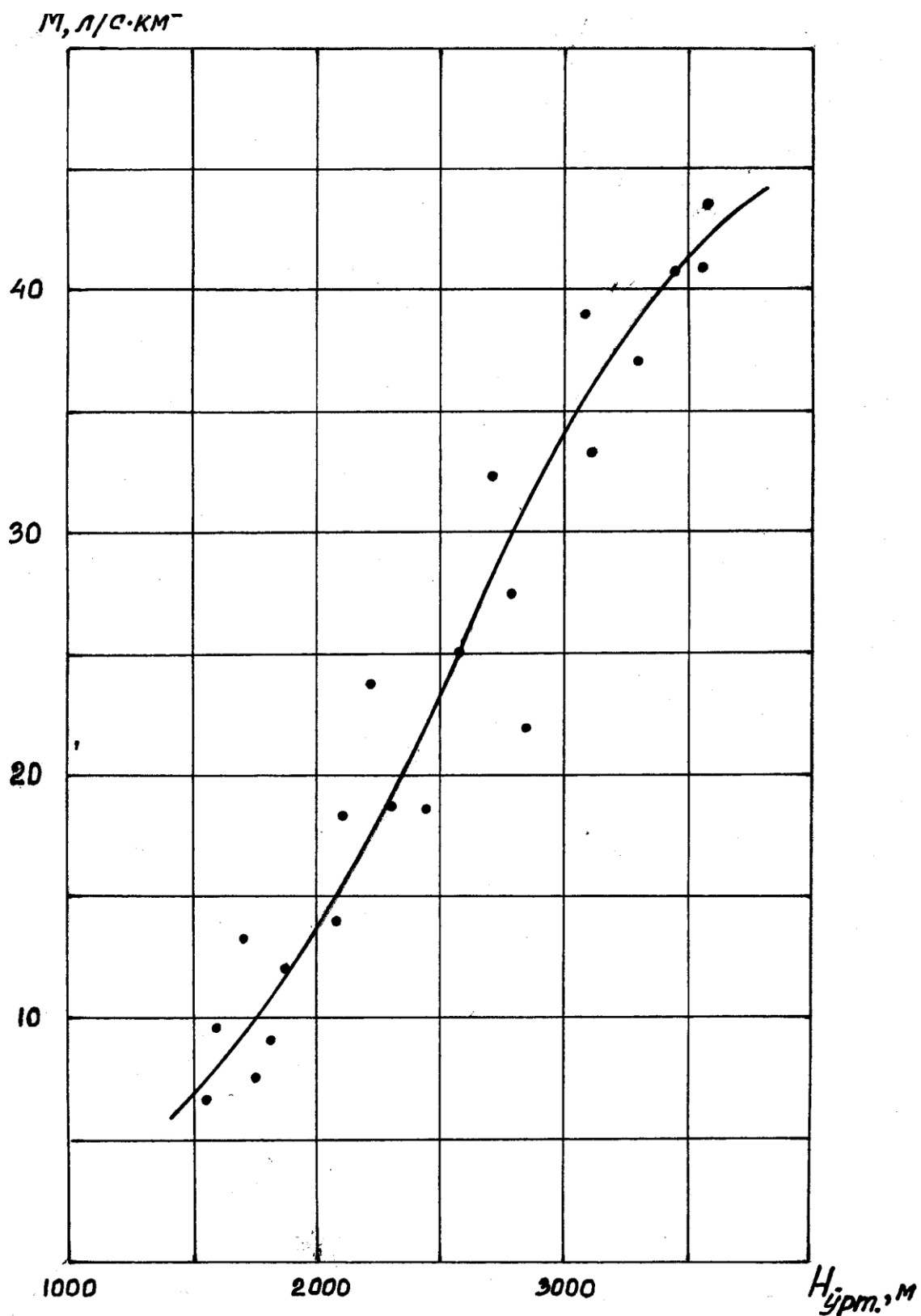
23-расм. Оқим модули ( M )нинг ҳавзанинг ўртача баландлиги ( H_{урт} ) га боғлиқлигини ифодаловчи чизма.
