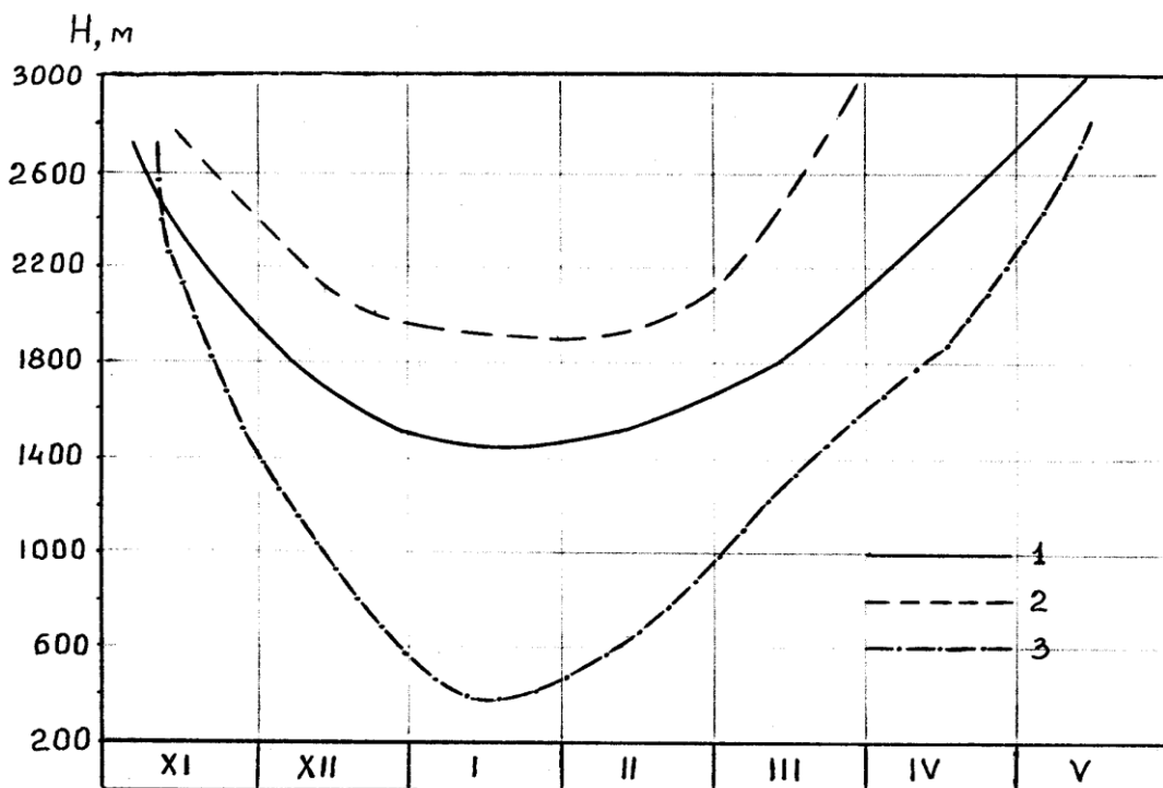
46-расм, а. Қашқадарё ҳавзасида мавсумий қор чегара — сининг фаслий ўзгариши. 1 — ўртача кўп йиллик, 2 — энг кичик, 3 — энг катта.
