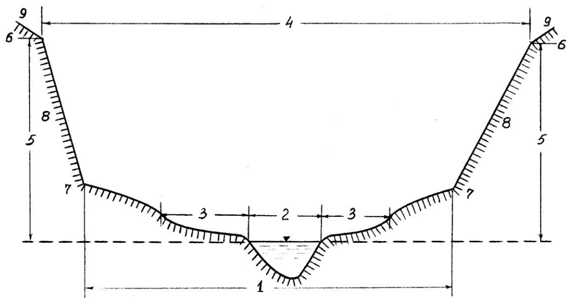
11-расм, А. Дарё водийсининг кўндаланг қирқими
