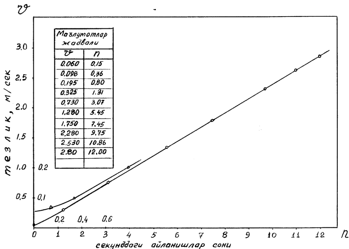
19-расм. Гидрометрик парракни даражалаш чизмаси
