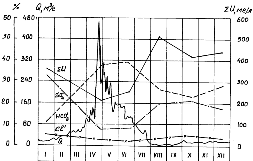
28-расм. О'зангарон дарёси сувининг (Самарское қўрғони яқинида) минераллашуви ва ундаги асосий анионлар миқдорининг йил давомида ўзгариши (1952 й.).
