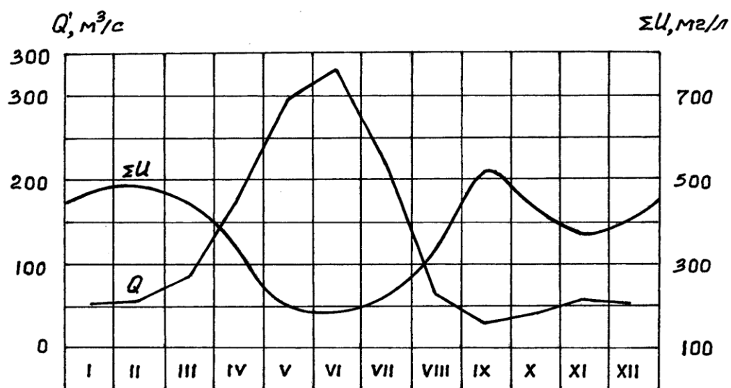
30-расм. Чирчиқ дарёси (Чиноз яқинида) ўртача кўп йиллик сув сарфи ва минераллашувининг йил давомида ўзгариши.
