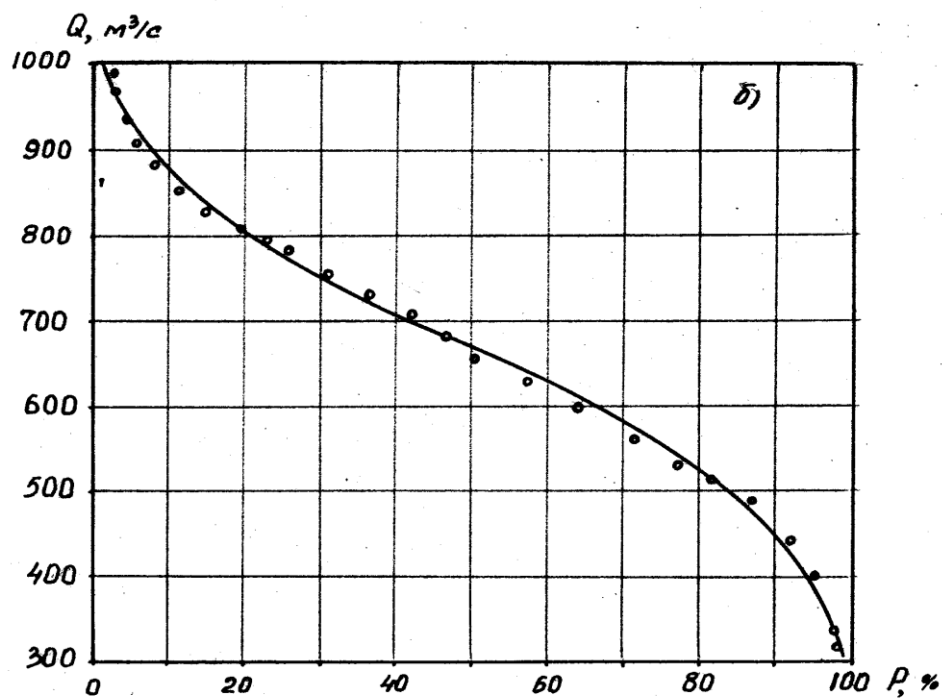
24-расм. Дарё оқимининг йиғинди (а) ва таъминланиш (б) эгри чизиқлари.
