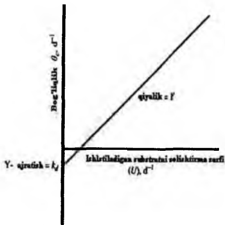
68-rasm. Y va k_d biokinetik koeffitsiyentlarni aniqlash.
