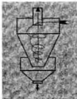
25-rasm. Siklonning tuzilishi.
