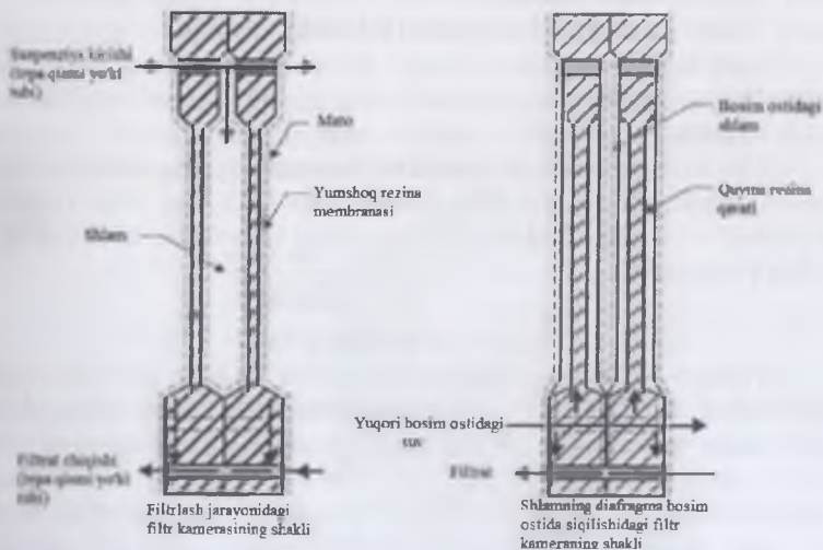
92-rasm. O'zgaruvchan hajmli plastinali pressing ko'ndalang kesimining ko'rinishi.
