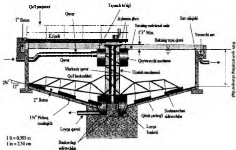
53-rasm. Gravitatsion quyuqlashtirgich sxemasi. Manba: ERA (1979) Cho'kmani qayta ishlsh va ajratib olish qo'llanmasi. , b. 5–6. AQShning atrof-muhitni muhofaza qilish agentligi.
