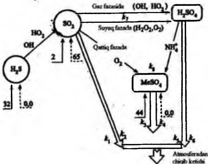
17-rasm. Oltinigugurt birikmalarining atmosferadagi aylanma harakati sxemasi.
