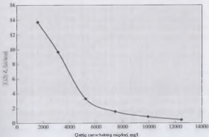
79-rasm. Qattiq zarrachalarning miqdorini cho'kish tezligiga bog'liqligi.
