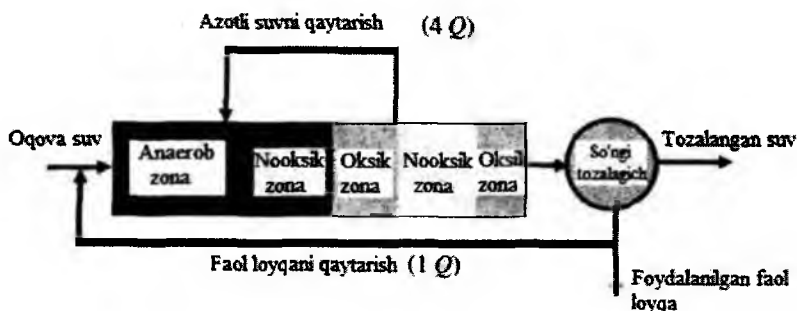
76-rasm. 5-bosqichli Bardenfo jarayoni sxemasi.
