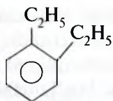
orto-dietil benzol ( o -dietil benzol)
