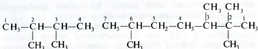
2, 3-dimetilbutan
