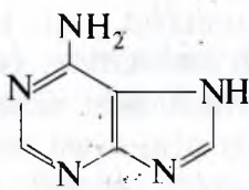
adenin
