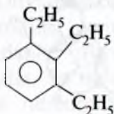
trietil benzol
