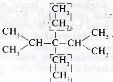
dietildiiizopropilmetan
