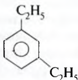
meta-dietil benzol ( m -dietil benzol)
