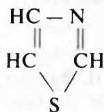
tiazol
