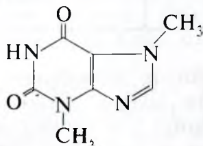
teobromin (3,7-dimetilksantin)
