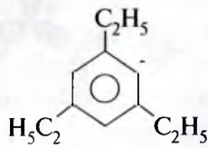
simmetrik trietil benzol
