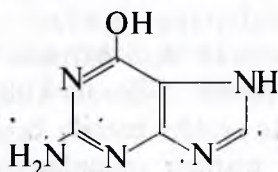
adenin
