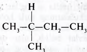
dimetiletimetan
