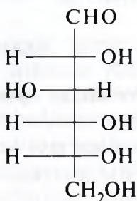
D-glukoza
