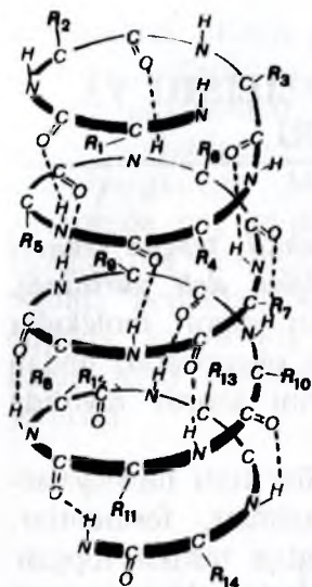
14.1-rasm. Oqsil molekulasi- ning ikkilamchi strukturasi.
