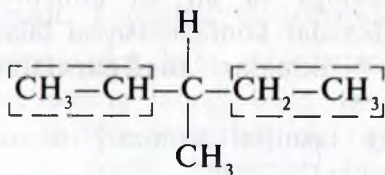
metildietimetan
