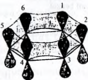
9.2-rasm. Benzol molekulasida \pi -bog'larning hosil bo'lish sxemasi.
