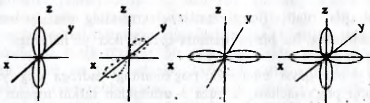
p - elektron orbitalining shakllari ya fazoda mumkin bo'lgan yo'nalishlari.
