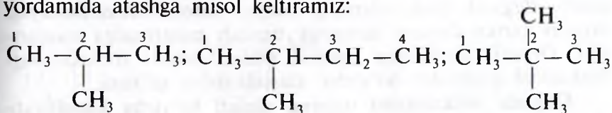
2, 2-dimetilpropan
