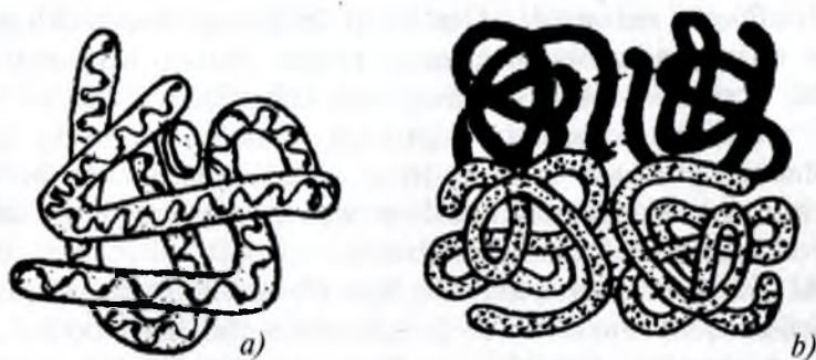
14.2-rasm. Oqsil molekulasining: a —uchlamchi, b —to'rtlamchi strukturasi.
