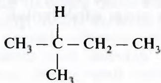
dimetiletilmetan
