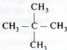
tetrametilmetan
