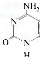
sitozin
