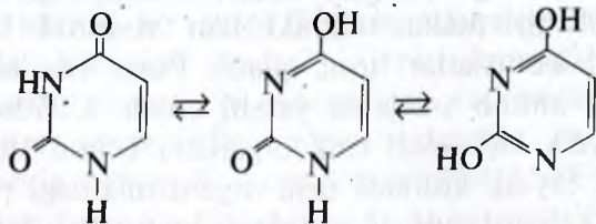
uraesil va uning tautomer shakllari
