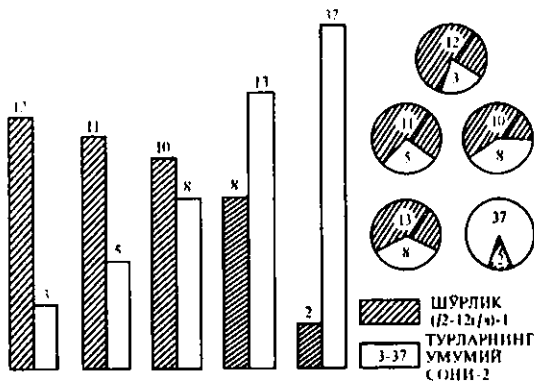
31-расм. Ўрта Осиё шароитида сувнинг шўрлигининг (1) ортиши билан Scenedesmus туркуминининг турлар сонининг (2) ўзгариши.
