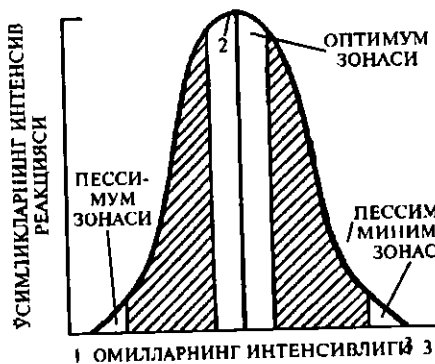
5-расм. Экологик омилларнинг ўсимликларга таъсир қилиши (Одум, 1975)
