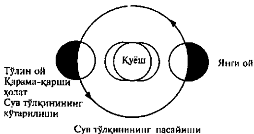
36-расм. Ойнинг фазалари (Гремажск, 1988)
