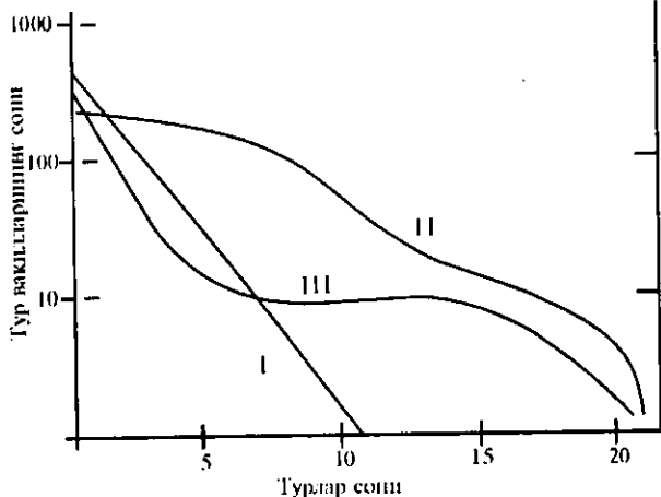
65-рәсм. Турларнинг ҳар хиллигини кўрсатувчи схема (20 турга 1000 та тур вакили, ориг.).
