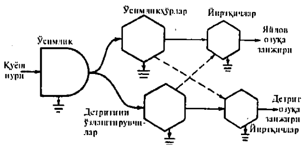
78-расм. Озуқа занжирлари
