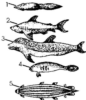
33-расм. Актив сузувчи гидробионтларнинг таъна шаклининг ўхшашлиги: 1-бошоқлик моллюскалар; 2-акула; 3-дельфин; 4-дюгонь; 5-дирижабл (Зернов, 1949)
