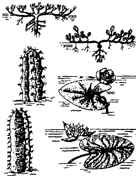
37-расм. Ўсимликларнинг ҳаётий шакллари (Раункиер буйича).
