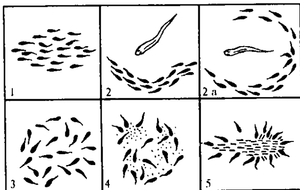
56-расм. Пелагик балиқларнинг гал. бўлиб яшаш типлари: 1—сузиб юриш вақти; 2—ҳимоя вақти; 3—сиза шакли; 4—озикланиш вақти; 5—йиртқичларнинг озиқга ташланиши (Радкевич, 1983)
