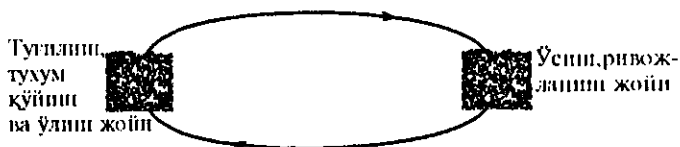
62-расм. Ҳайвонларнинг бир томонга миграцияси
