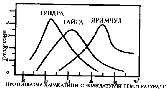
24-расм. Ўсимликларнинг тарқалиши ва уларнинг иссиқликка чидамлилиги ўртасидаги муносабат (Кислюк ва бошқ.)
