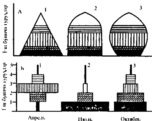
54-расм. Хайвонлар популяциясында ёш бүйиңча тузулиши. А— умумий схема; Б— молоскалар популяциясинин турли-ёшли гуруҳларининг фазслар бүйиңча ўзгариши (Одум, 1975).
