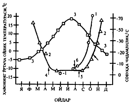
23-расм. Ўсимликларнинг чидамлилиги: тоғда ўсувчи Salix rauciflora (1), S.sachal (2)ларнинг совуққа чидамлилигида йилнинг ўртача ҳарорати (3); 4—баргнинг чиқиши; 5—баргнинг саргайиши; 6—куртақларнинг тугилиши (Бигон, 1989)
