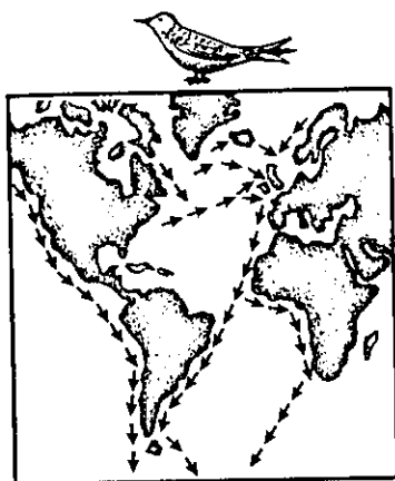
61-расм. Кутб крачкасини ( Sterna paradisaea ) миграция йўли
