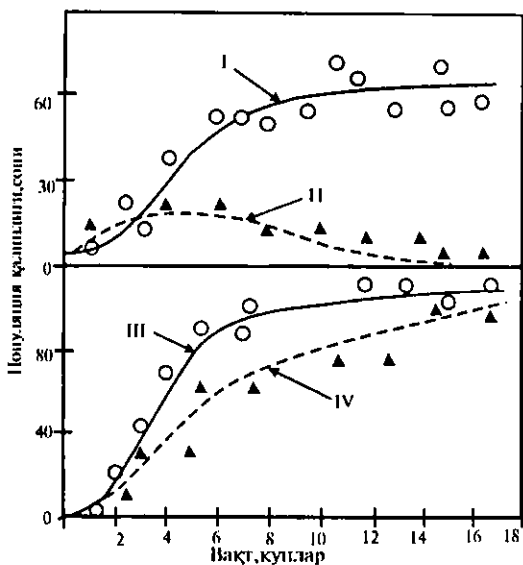
44-расм. Бир-бирига яқин тубан организмларнинг икки тури ўртасидаги рақобат: I— Paramecium caudatum ни доим озикли жойда алоҳида ўсиши; III— Paramecia ни алоҳида ўсиши; II, IV— икки турни бирликда ўсиши (Одум, 1986).
