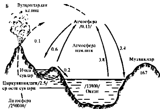
84-расм. Табиатда сувнинг айланиши (Хатчинсон буйича)
