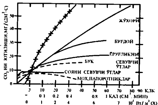
15-расм. Турли ўсимликларнинг фотосинтез жараёнига ёруғликнинг таъсири (Лархер бўйича)
