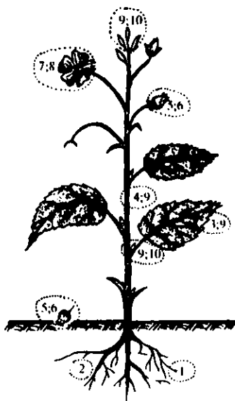
64-расм. Организмларни озиқланиш бўйича экологик нишаларни (Одум, 1986): 1-илдиз; 2-илдиздан ажратилган моддалар; 3-барг; 4-поя, тана; 5—6-уруғ ва мева; 7—8-гул, чанг; 9-шира; 10-куртак.
