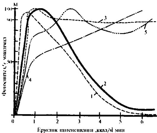
76-расм. Яшил (1), диатом (2) сувўтлари, эмон (3), қарагай (4) ва қизил (5) дарахтларда фотосинтез ва ёруғлик активлигининг бир-бирига боғлиқлиги (Реклефс, 1979)
