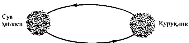
60-расм. Организмларнинг кун давомидаги миграцияси.
