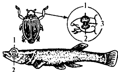
17-расм. Сув юзасида сузувчи сузгич кўнғиз ( Quyrinus ) ва Тўрткўз балиқнинг ( Anableps ) кўз тузилиши: 1 — кўзни ҳавода кўришга мослашган юқорги қисми; 2 — кўзни сувда кўришга мослашган пастки қисми; 3 — сузгич кўнғизни тукини ўрнашган жойи (Чернова, Былова, 1988).
