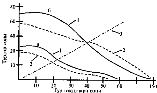
68-расм. Икки хил каналда яшил ва диатом сувўтларнинг турлар бўйича тузилиши: а-ифлос канал; б-тоза канал; 1-диатом сувўтлар; 2-яшил сувўтлар; 3-сувнинг ифлосланиш чизиги (ориг.).
