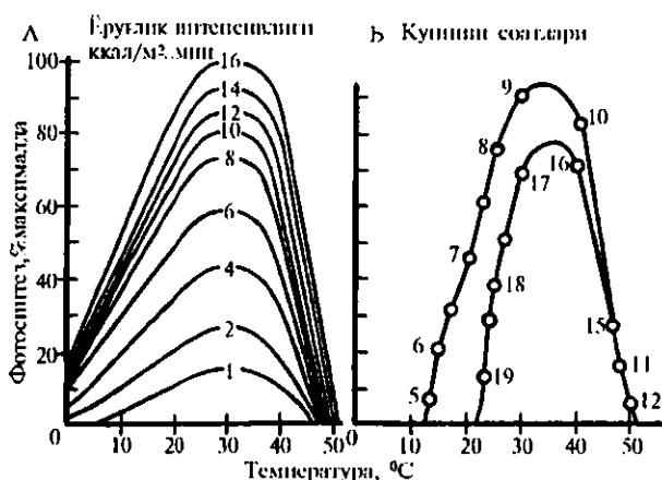
77-расм. Фотосинтез активлигининг барг ҳарорати ва нурунинг тушшига (А) боғлиқлиги. Фотосинтезнинг кун давомида ўзгариши (Б) (Реклефе бўйича)
