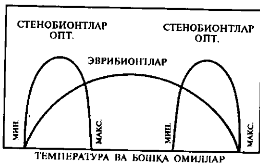
7-расм. Турларнинг экологик валентлиги (Одум, 1975, 1986)
