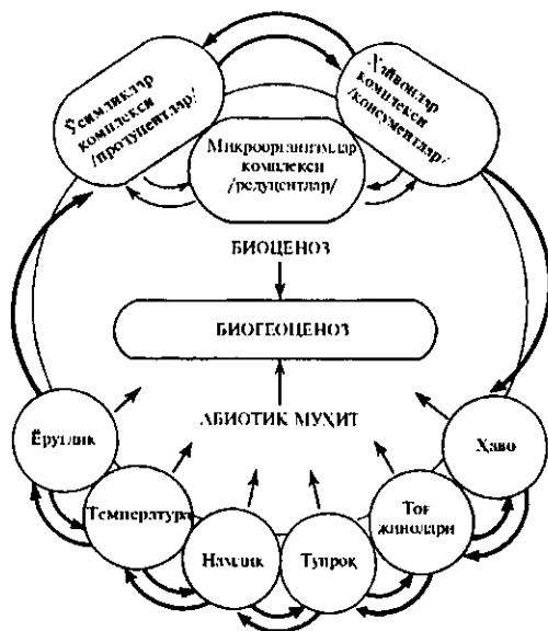
69-расм. Биогеоценоз ичидagi алоқаларнинг тузилиши (Понамарева, 1975).
