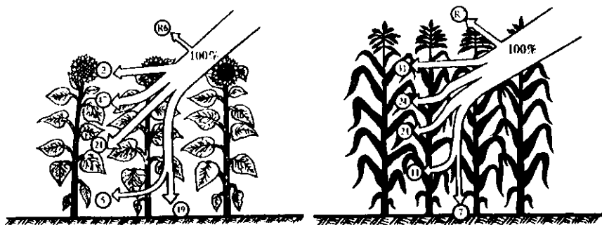
13-расм. Турли ўсимликлар қопламига қуёш нурунинг ўтиши (Лархер, 1975).
