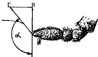
34-расм. Сув юзасида яшайдиган кананинг ( Velia ) олдинги оёқларидаги тарзус ҳаракати: \alpha -юза қисм бурчак деформациясида; F-тахминан 90 — 180^{\circ} атрофида тепага (в) кўтарилиш кучи ҳосил бўлади (Дажо, 1975).
