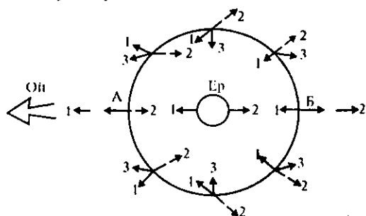
35-расм. Ер юзида тўлқинлар ҳосил қилувчи кучлар: 1-ойнинг тортиш кучи; 2-марказдан қочирма куч; 3-тўлқинлар ҳосил қилувчи куч. А-ойнинг юқори чўққанда туриши; Б-ойнинг орқа томони
