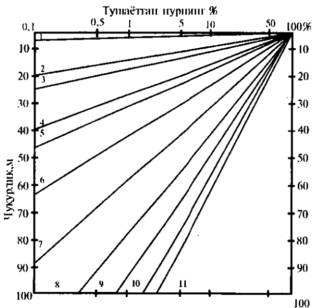
29-расм. Турли табиий сувларининг тиниқлиги (чириклар сарик яшил нурлар-5000-6000 А); (Дажо, 1975)
