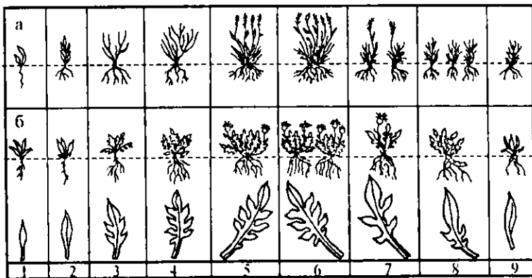
53-расм. Ўтлоқзордаги ёввойи суяги (А) ва сибир кўзтикон (Б) популяциясининг ёш бўйича тақсимланиши: 1-ўсимта; 2-ювениль ўсимлик; 3-имматур ҳолат; 4-виргинал; 5-ёш генератив; 6-ўрта ёшдаги генерация; 7-қари генерация; 8-9-қурган синеал ҳолатлар (Чернова, Билова бўйича)
