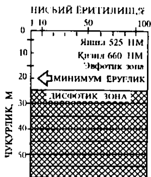
12-расм. Мўътадил зонадаги эвтроф кўлни ёздаги стратификация пайтида радиациянинг ўзгариши (Лархер, 1975).
