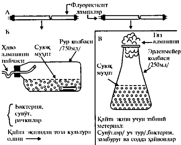
74-расм. Лаборатория микроэкоцистемаси: А— ёруғлик манбаи; Б, В— берк идиш
