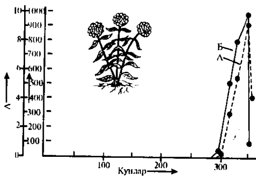
59-расм. Бир йиллик Phlox drummondii ўсимлигининг кўпайиш динамикаси. А — уруғ сонининг ўзгариши; Б — бутун популяцияда етишган уруғ сони (Бигон бўйича)
