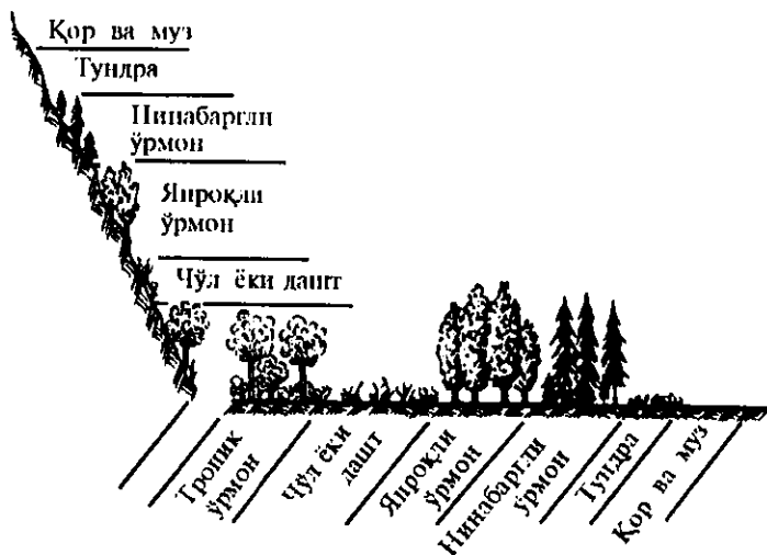
20-расм. Ҳосимликларнинг вертикал ва кенгликда зоналаниши (Горишина, 1971)
