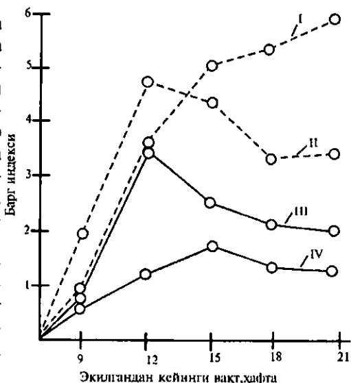
46-расм. Себарога турларининг яшаш ҳолати: I — Trifolium fragiferum алоҳида, тоза экилган; II — T. repens тоза экилган; III — T. repens аралаш экилган; IV — T. fragiferum аралаш экилган (Одум, 1986).
