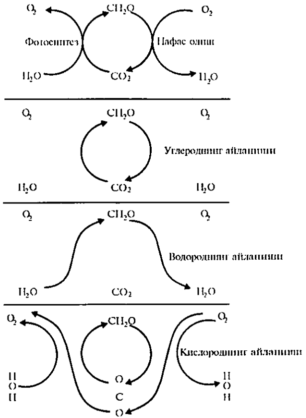
81-расм. Углерод, водород ва кислороднинг табиатда айланиши (Риклефе, 1979)
