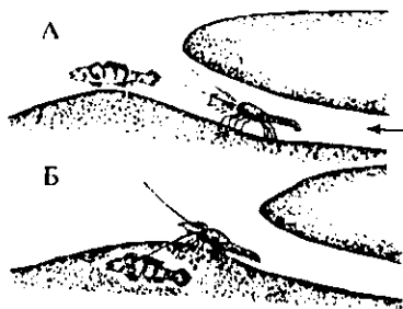
48-расм. Мутализм жараёнида криветка ( Alpheus djiboutensis ) ва балиқ ( Sturteocentrus ) уядан олдинма кейин чиқмоқда (А); Б— криветка шидан чиққан, бир антеннаси балиққа тегиб турипти (Битон, 1989)
