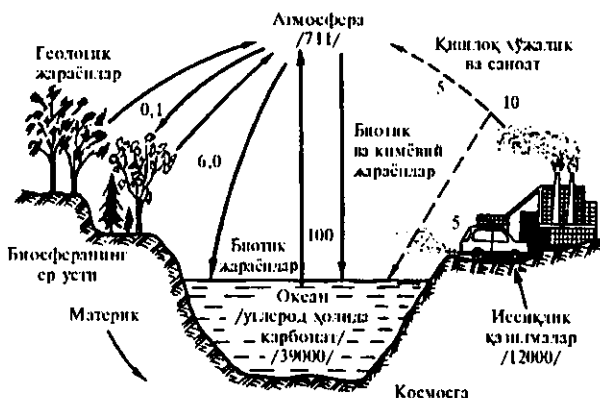
80-расм. Углероднинг табиатда айланиши (сонлар млрд.т.) ва биосферанинг қисмларида ўзгариши (Одум бўйича)
