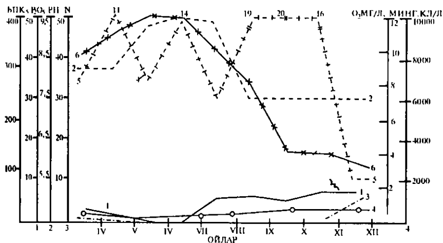
75 а-расм. Чирчик биологик ҳовузларида фитопланктоннинг ривожланиши (6) билан оқова сувларнинг кимёвий (мг/л) таркибининг ўзгариши: 1-фосфор; 2-pH; 3-умумий азотнинг миқдори; 4-БПК 5 ; 5-CO 2 ; 6-фитопланктоннинг миқдори
