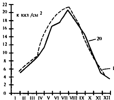
10-расм. Ўрта Осиёда қуёш радиациясининг ойлар бўйича миқдори, ккал/см². 1—1968 йил; 2—1988йил.
