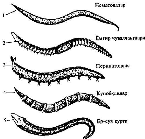
41-расм. Чувалчангсимон гидробийонтларнинг ҳаётий формалари (Шарова ва Свешникова, 1988)
