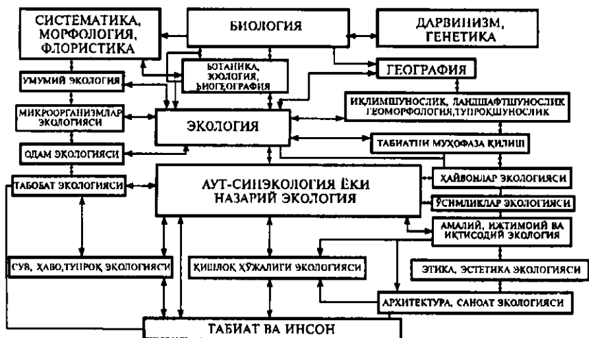
2-расм. Экологиянинг бошқа фанлар билан алоқаси
