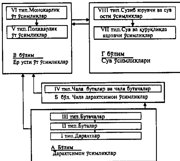
40-расм. Серебряковнинг ўсимликлар ҳаётий формаларига оид схемаси
