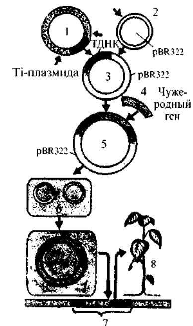
Рис. 12. Основные этапы получения трансгенного растения.
