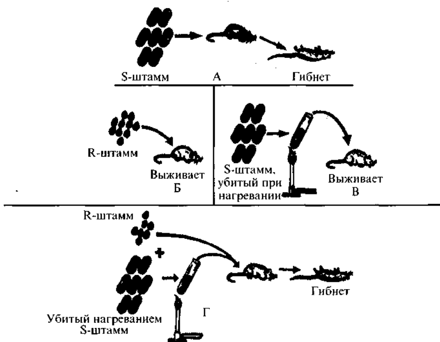
Рис. 4. Схематическое изображение опыта Гриффита: А — мышь, зараженная патогенной (болезнетворной) пневмококковой бактерией (S-штамм), погибает; В — мышь, зараженная непатогенной (?-штамм) пневмококковой бактерией, выживает; В — мышь, зараженная патогенной бактерией, убитой нагреванием, выживает; Г — при смешивании S- и Л-штаммов бактерий и введении этой смеси мыши она погибает. В ее крови обнаруживается живой S-штамм. Это свидетельствует о том, что при введении в организм мыши смеси, состоящей из непатогенного R- и убитого S-штаммов, ген наследственности молекулы S-штамма, вызывающий болезнь, переносится в наследственную молекулу живого R-штамма и придает ей свои свойства, т. е. происходит трансформация.
