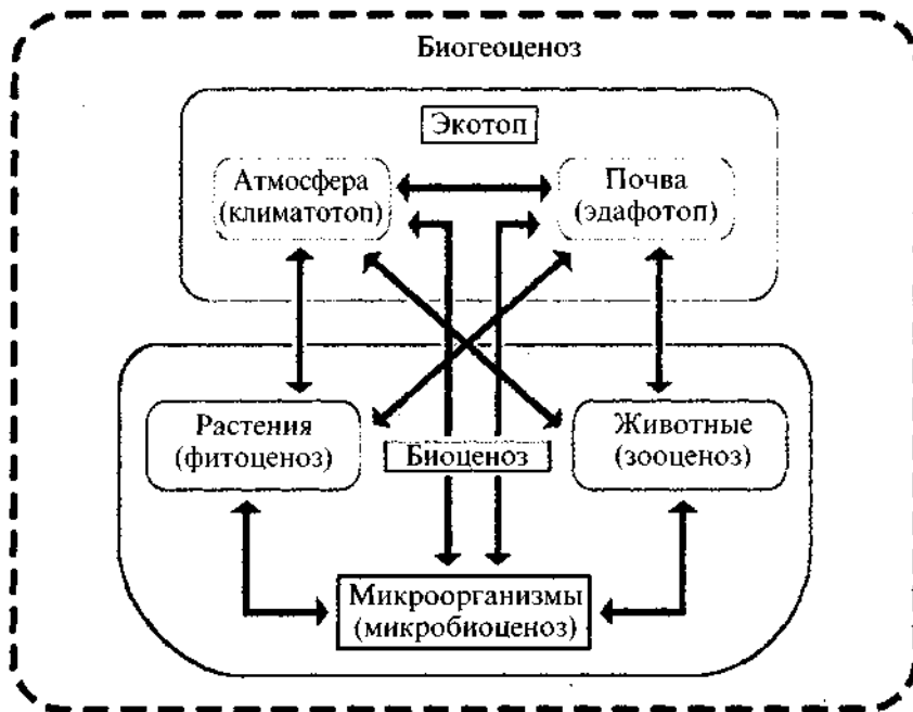
Р и с. 66. Схема биогеоценоза.
