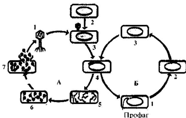
Рис. 6. Жизненный цикл фагов:
