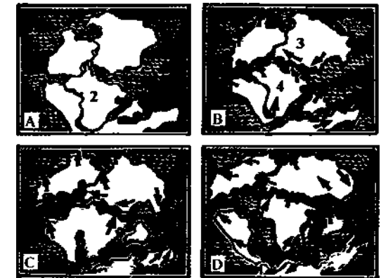
Рис. 52. Образование континентов в историческом процессе: 1 — Тетис; 2 — Пангея; 3 — Лавразия; 4 — Гондвана.
