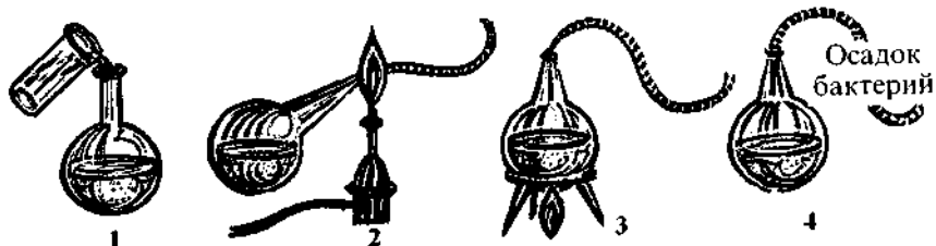
Р и с. 55. Опыты Луи Пастера.
