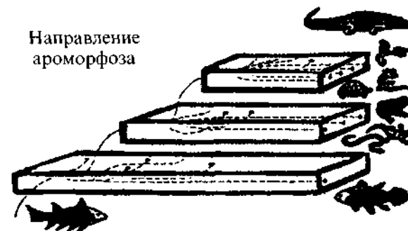
Р и с. 60. Различные направления эволюционного прогресса. Схематически изображены ароморфоз, идиоадаптация и общая дегенерация.
