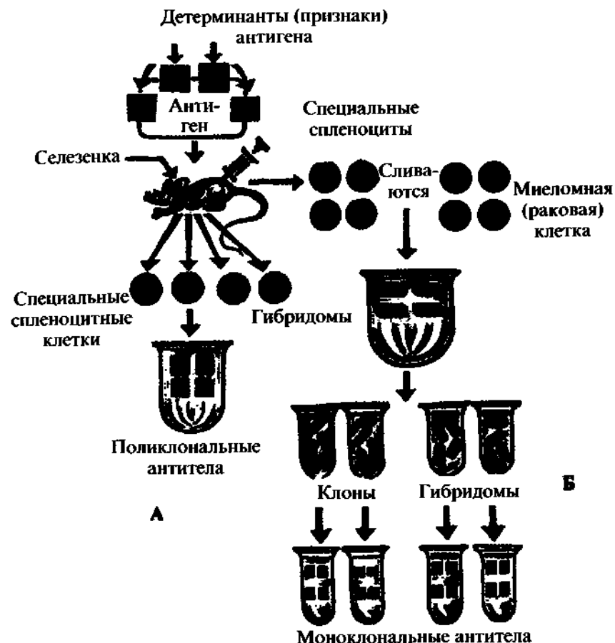
Р и с . 15. Схема получения поликлональных и моноклональных антител. А — получение поликлонального антитела. Мышь иммунизируется каким-нибудь антигенным веществом. В клетках селезенки образуются специальные спленоциты, синтезирующие антитела отдельно для каждой антигенной группы вещества. Они могут распознавать только свою соответствующую антигенную группу. Образовавшаяся смесь различных антител называется поликлональными антителами. Б — получение гибридом и синтез моноклонального антитела.
