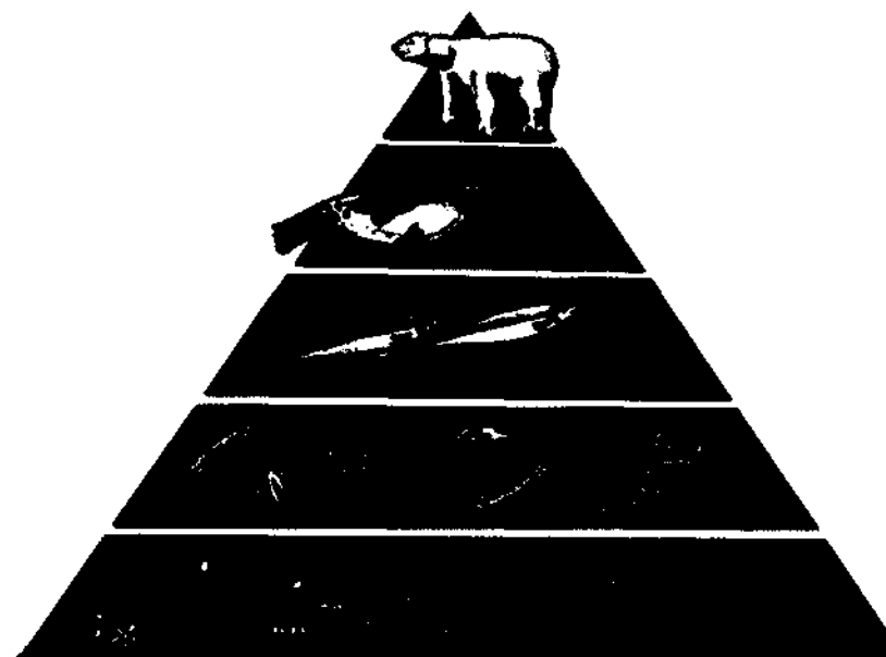
Рис. 68. Упрощенная экологическая пирамида.
