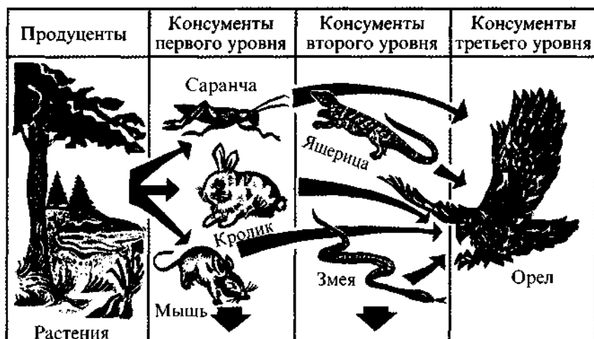
Рис. 67. Пищевая цепь.
