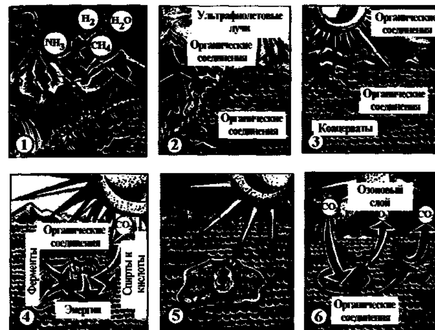
Р и с. 56. Развитие жизни на Земле: 1 — первичная атмосфера; 2 — образование органических веществ; 3 — образование коацерватов; 4 — простое брожение; 5 — образование нуклеиновых кислот; 6 — образование фотосинтеза и процессов дыхания.
