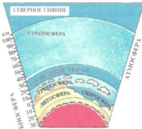
Рис. 74. Геосфера Земли.
