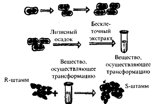
Рис. 5. Трансформация R-штамма в S-штамм путем смешения R-штамма с бесклеточным экстрактом, выделенным при расщеплении бактериальных клеток из пневмококка S-штамма.
