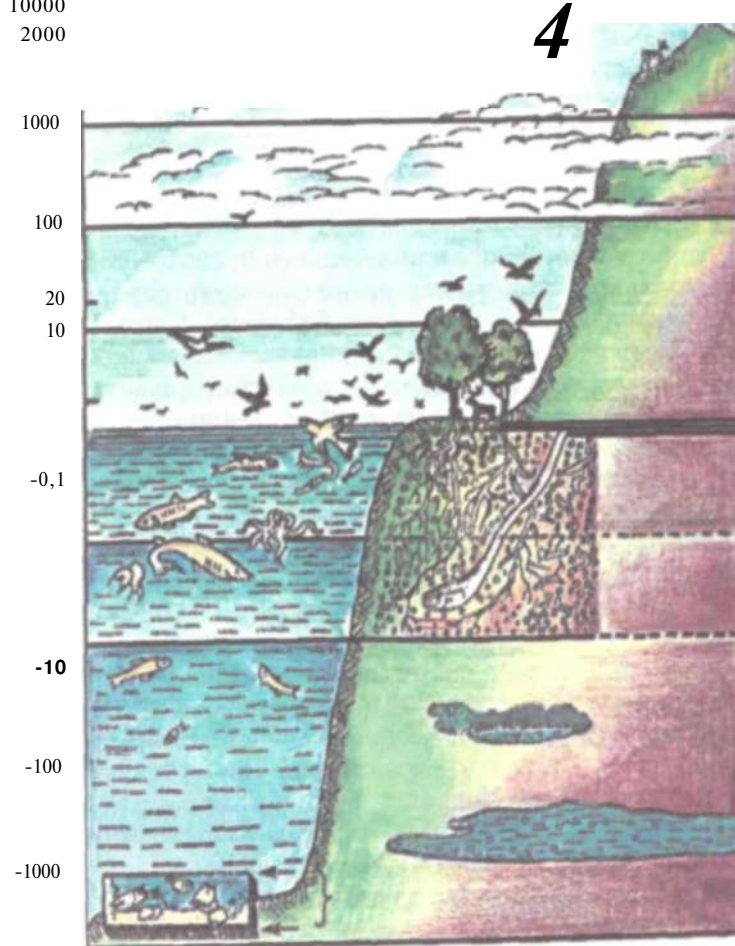
Рис. 75. Границы распространения жизни в биосфере.
