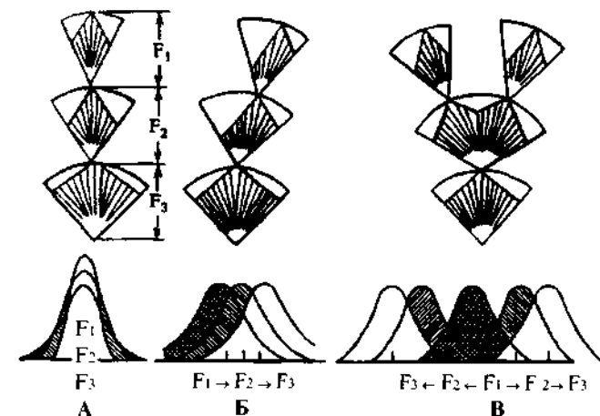
Рис. 31. Формы естественного отбора: схема действия стабилизирующего (А), движущего (Б) и дизруптивного (В) отбора; F — поколения. Заштрихованные участки — виды, вымершие на популяционной волне. Размер дуги окружности отбора внутри одного рода соответствует его норме реакции.
