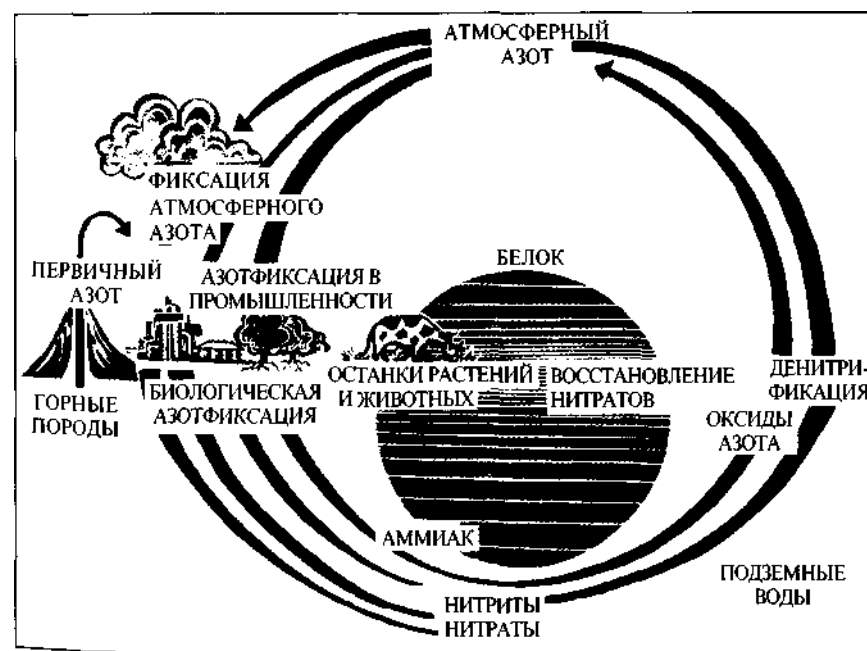
Рис. 77. Круговорот азота в биосфере.
