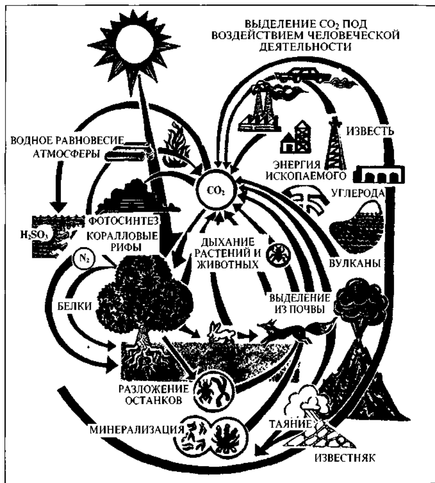
Рис. 76. Круговорот углерода в биосфере.
