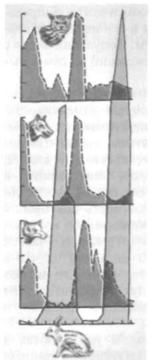
Рис. 42. Популяционные волны.
