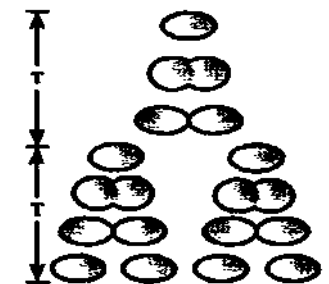
Рис. 1. Рост и размножение бактерий. Т — время, в течение которого бактериальная клетка делится один раз.
