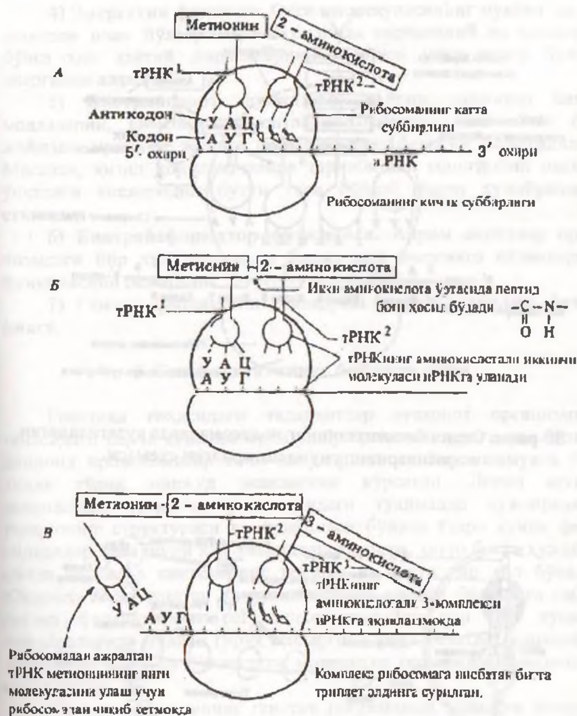
79-расм. Оксил биосинтези (трансляция) молекуляр механизмининг схемаси.
