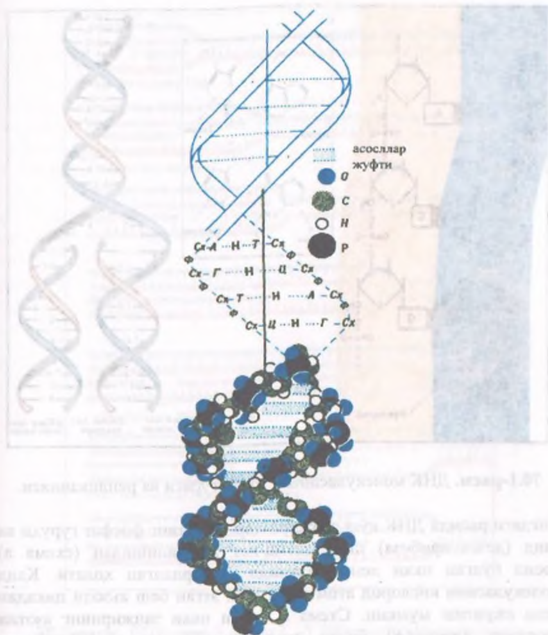
67-расм. ДНК молекуласи структурасининг изоҳли модели.
