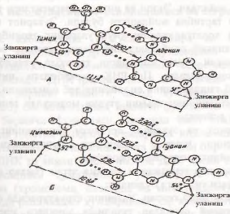
69-расм. ДНК молекуласида нуклеотидларнинг комплементар боғланиш тартиби.
