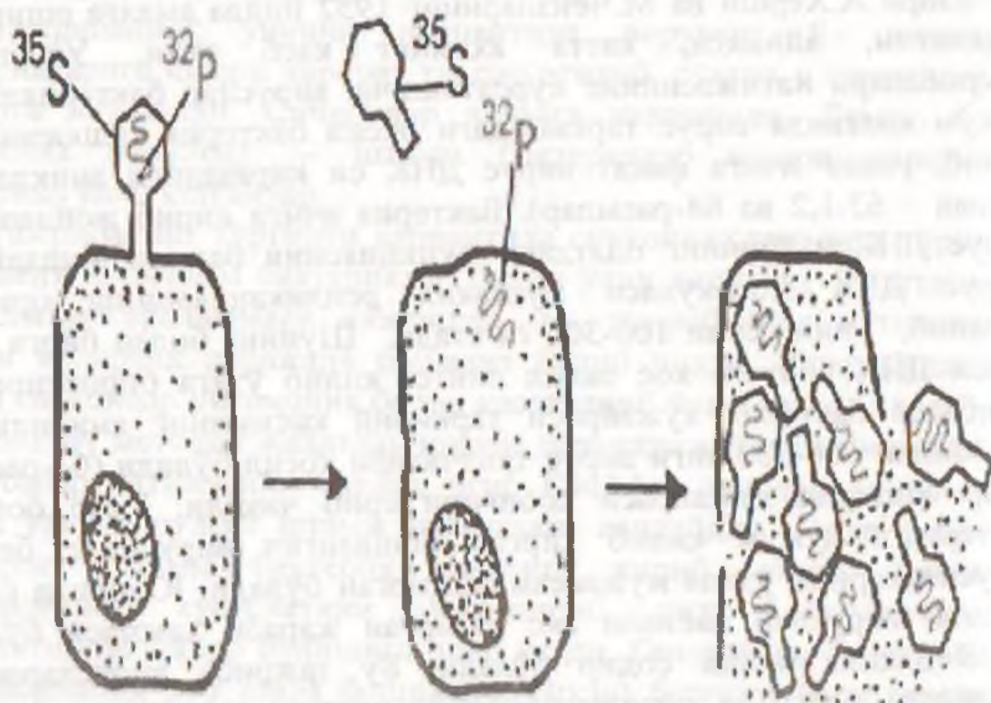
64-расм. T2 бактериофагининг ДНК орқали кўпайиш схемаси.
