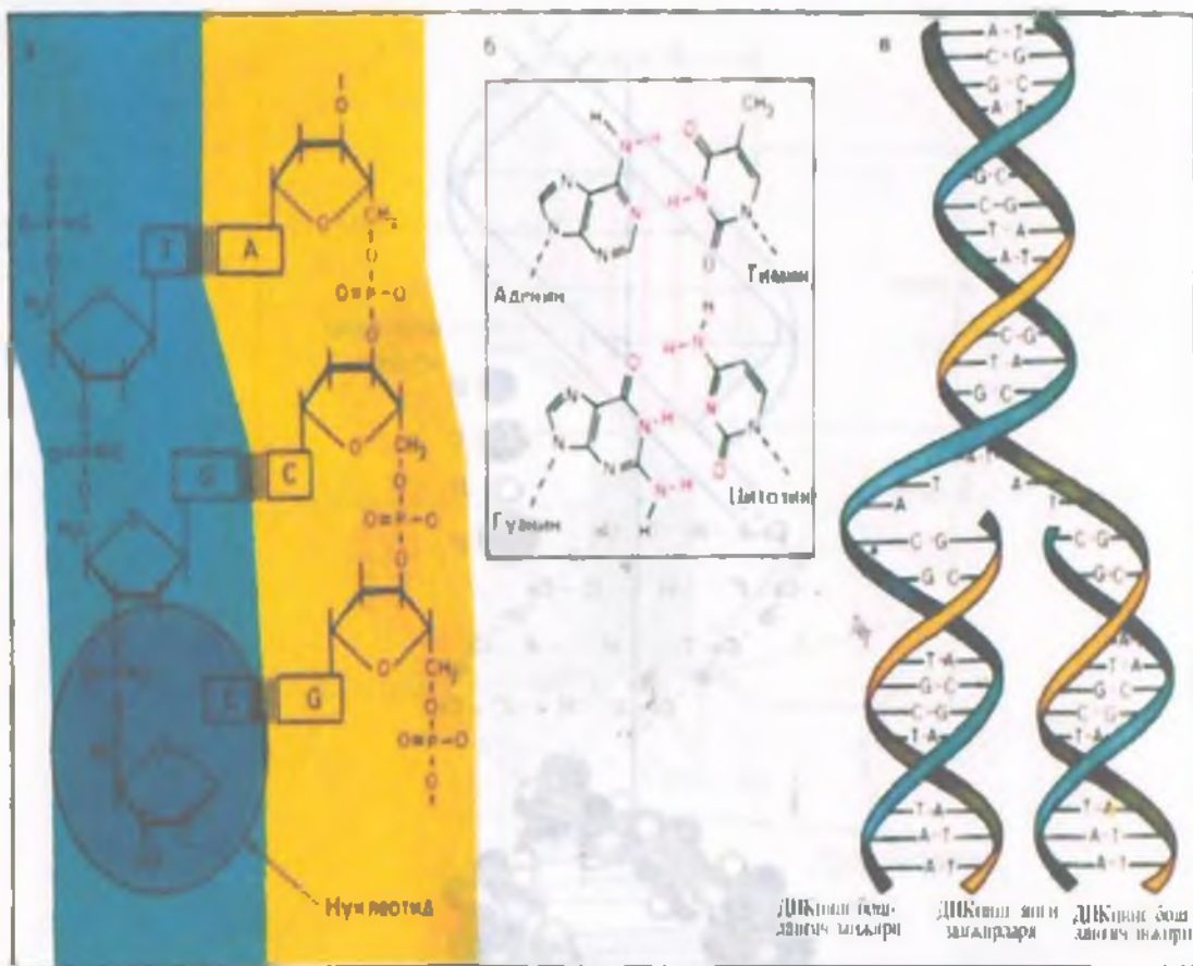
70.1-расм. ДНК молекуласининг структураси ва репликацияси.
