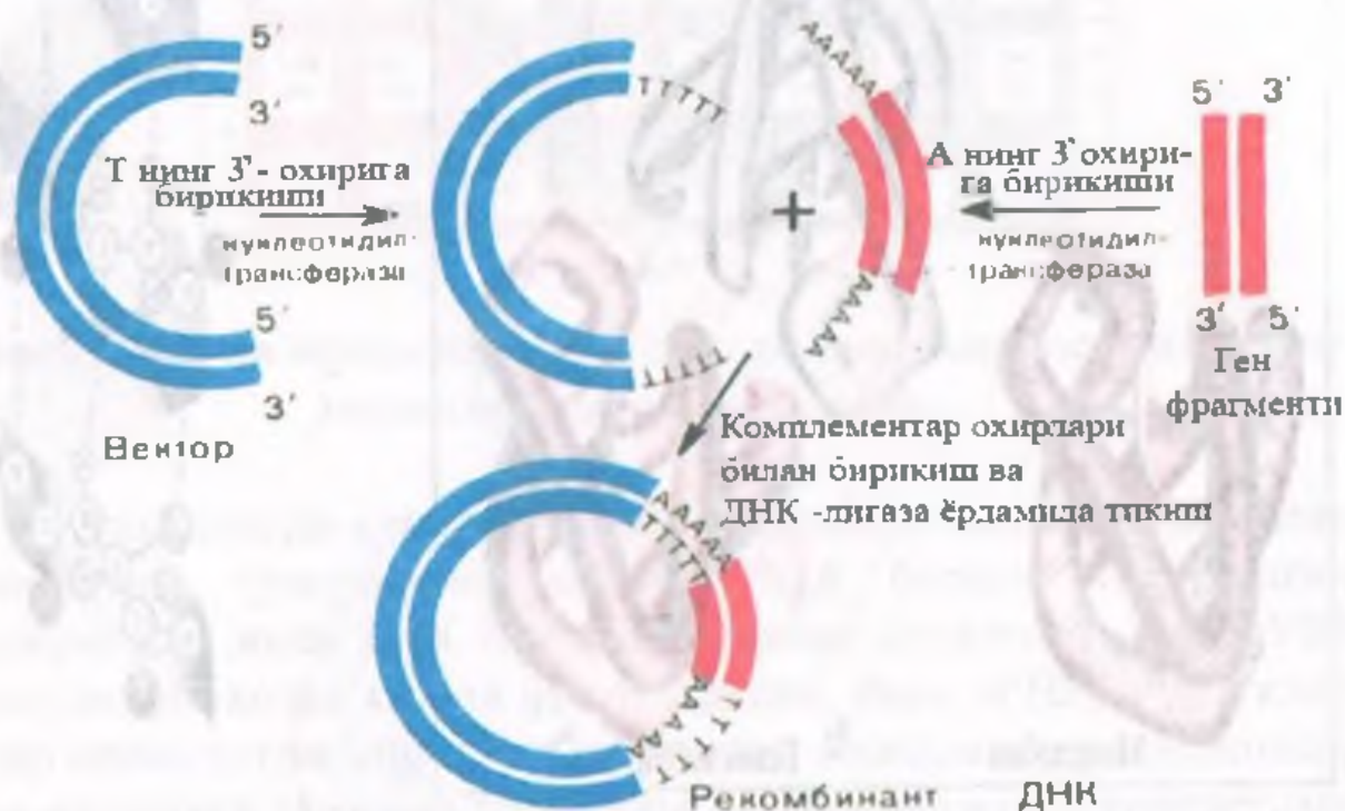
86-расм. Рекомбинант ДНК синтез қилинишининг схемаси.
