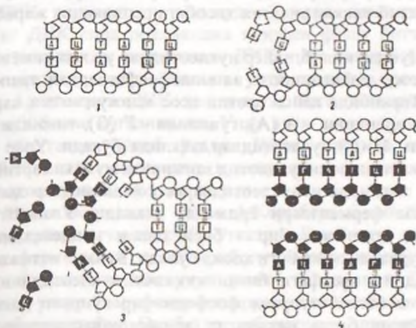
71-расм. ДНК репликациясининг ярим консерватив механизмининг схемаси:
