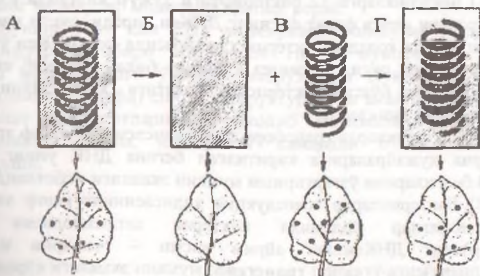
66-расм. Тамаки мозаика вирусига (ТМВ) РНКнинг ирсий ахборот роли.
