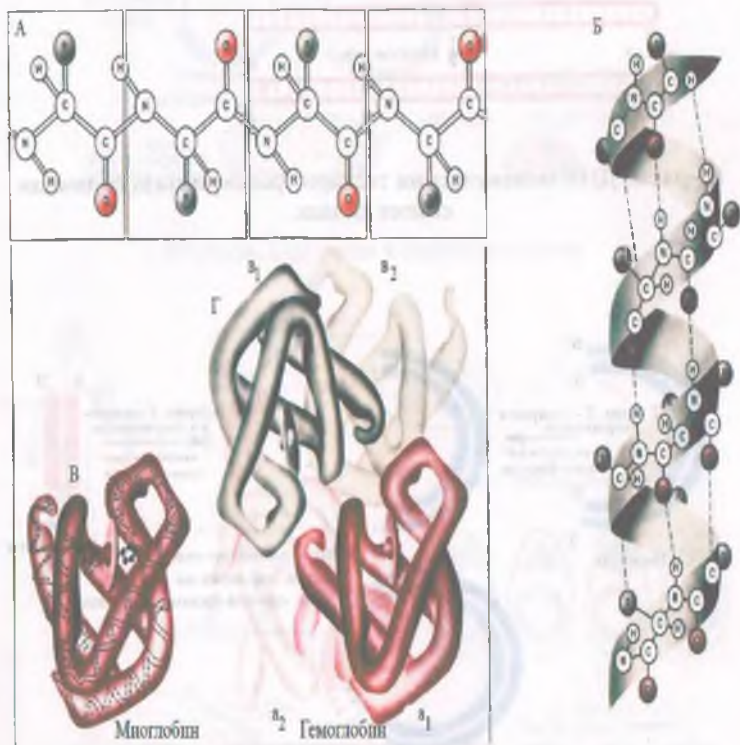
82-расм. Оксилнинг иккиламчи, учламчи ва тўртламчи структураси.
