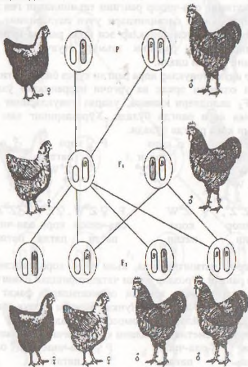
43.2-расм. Товукларда жинс билан бириккан ҳолда ирсийланиш.
