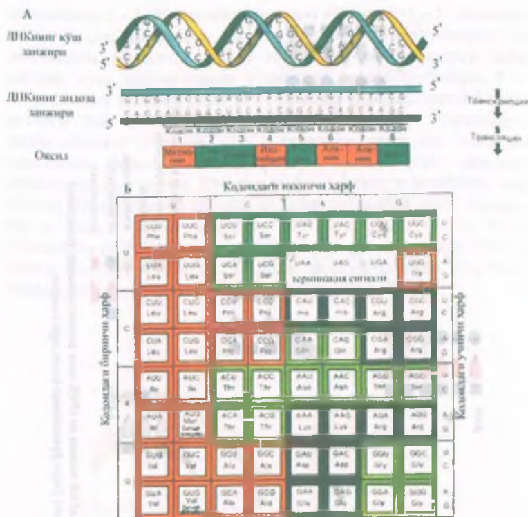
77-расм. ДНК да ифодаланган генетик коднинг маъносини аниқлаб топиш принциплари схемаси.
