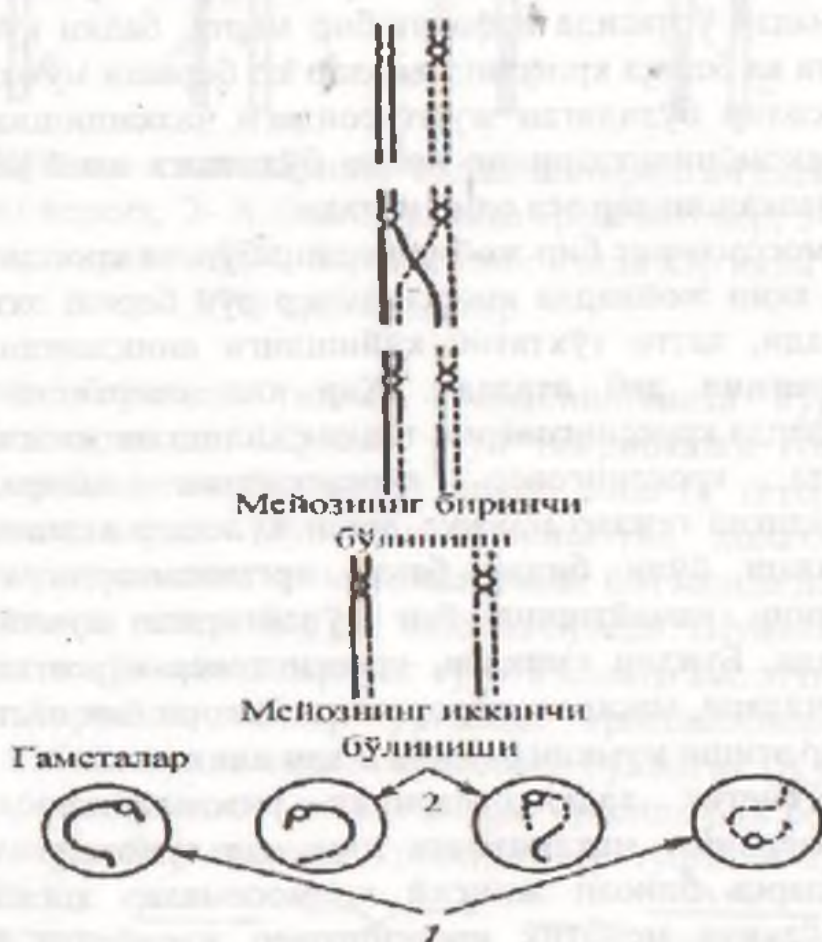
48-расм. Якка кроссинговердан сўнг гаметаларнинг ҳосил бўлиши.
