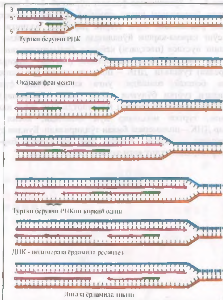
70.2-расм. ДНКнинг 5' -3' ва 3' -5' йўналишдаги нуклеотид занжирларининг репликацияси.
