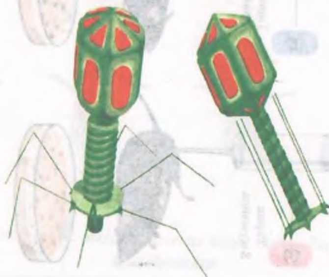
63.2-расм. T2 бактериофагнинг катта модели.
